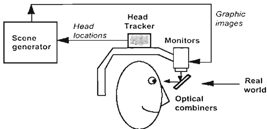
รูปที่ 32 แผนผังระบบความจริงเสริมแบบใช้ Optical See-through Head-Mounted Display [22]
