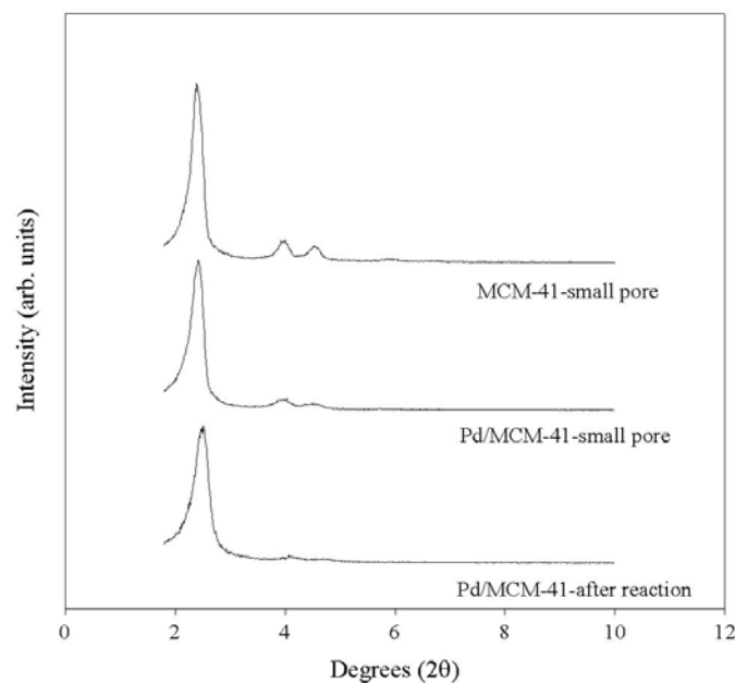
รูปแสดง XRD Patterns ของ MCM-41 และตัวเร่งปฏิกิริยา Pd/MCM-41 ก่อนและหลังทำปฏิกิริยา
