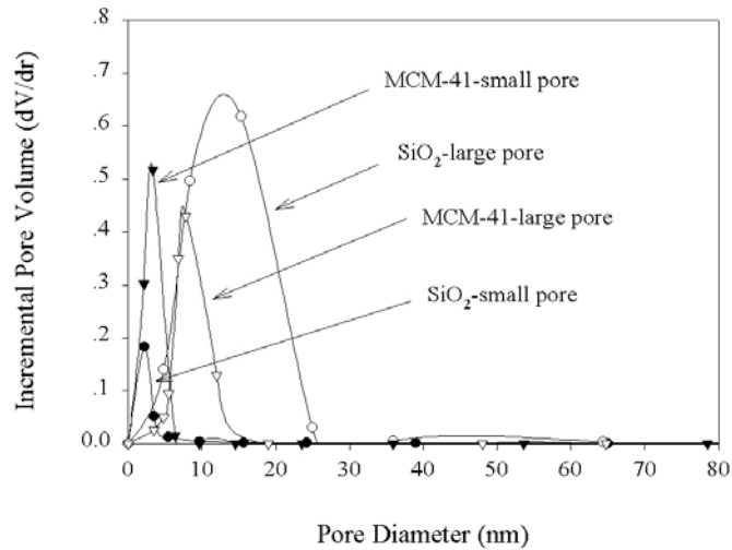
รูปแสดง Pore Size Distribution ของซิลิกาและ MCM-41
