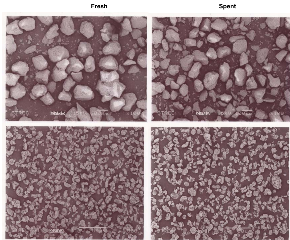
รูปแสดง SEM micrographs ของตัวเร่งปฏิกิริยาต่างๆ แกวบน \text{Pd-Cl/SiO}_2 แกวล่าง \text{Pd-Cl/MCM-41} ก่อนและหลังทำปฏิกิริยา
