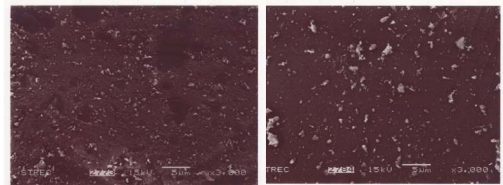
Pd-Cl/SiO 2
