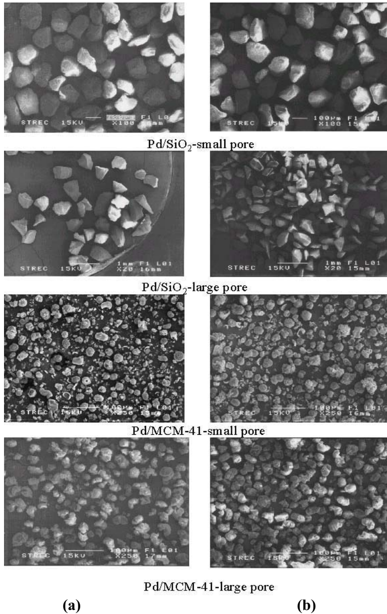
รูป SEM Micrographs ของตัวเร่งปฏิกิริยา (a) ก่อนทำปฏิกิริยาและ (b) หลังทำปฏิกิริยา
