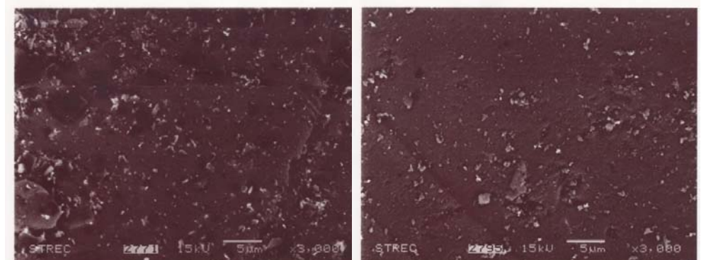
Pd-NO 3 /SiO 2
