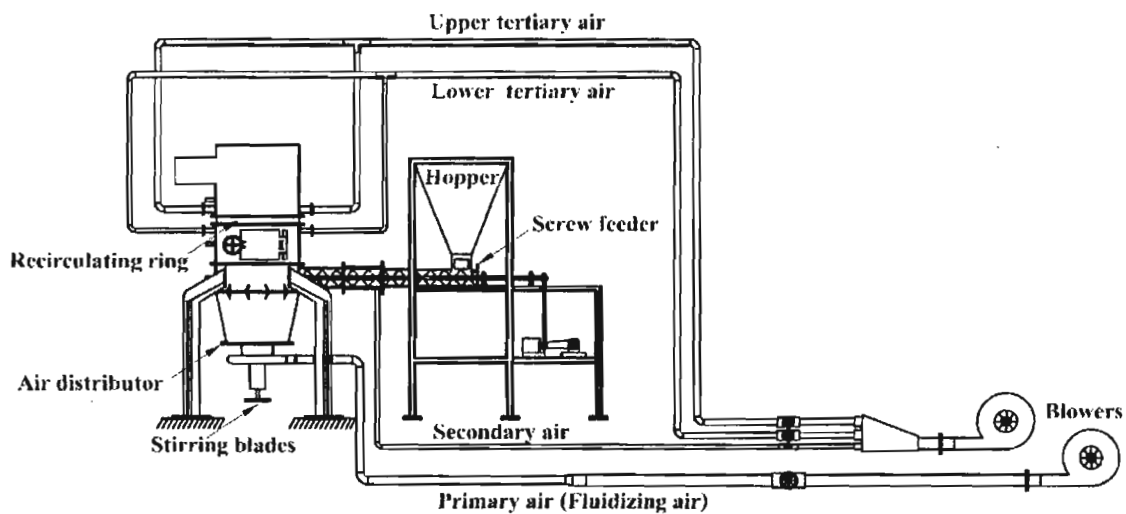
รูปที่ 1(ก) แสดงไดอะแกรมของเตาเผาไหม้ฟลูอิดาเบดแบบห้องเผาไหม้สันขนาด 250 kW th
