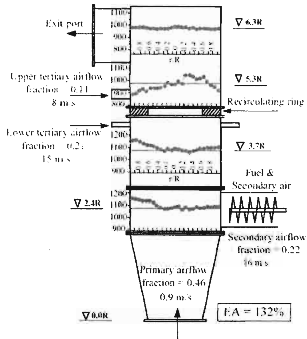
รูปที่ 4 การกระจายอุณหภูมิในแนวนอนของเตาเผาไหม้ที่ระดับต่างๆ
