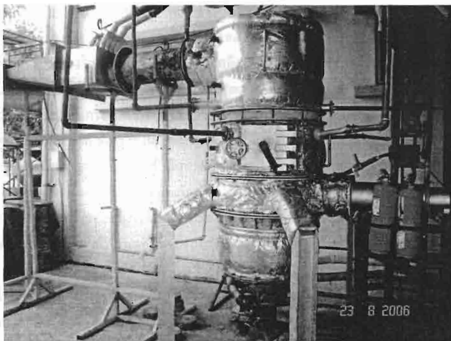
รูปที่ 1(ข) แสดงภาพถ่ายของเตาเผาไหม้ฟลูอิดาเบดแบบห้องเผาไหม้สันขนาด 250 kW th
