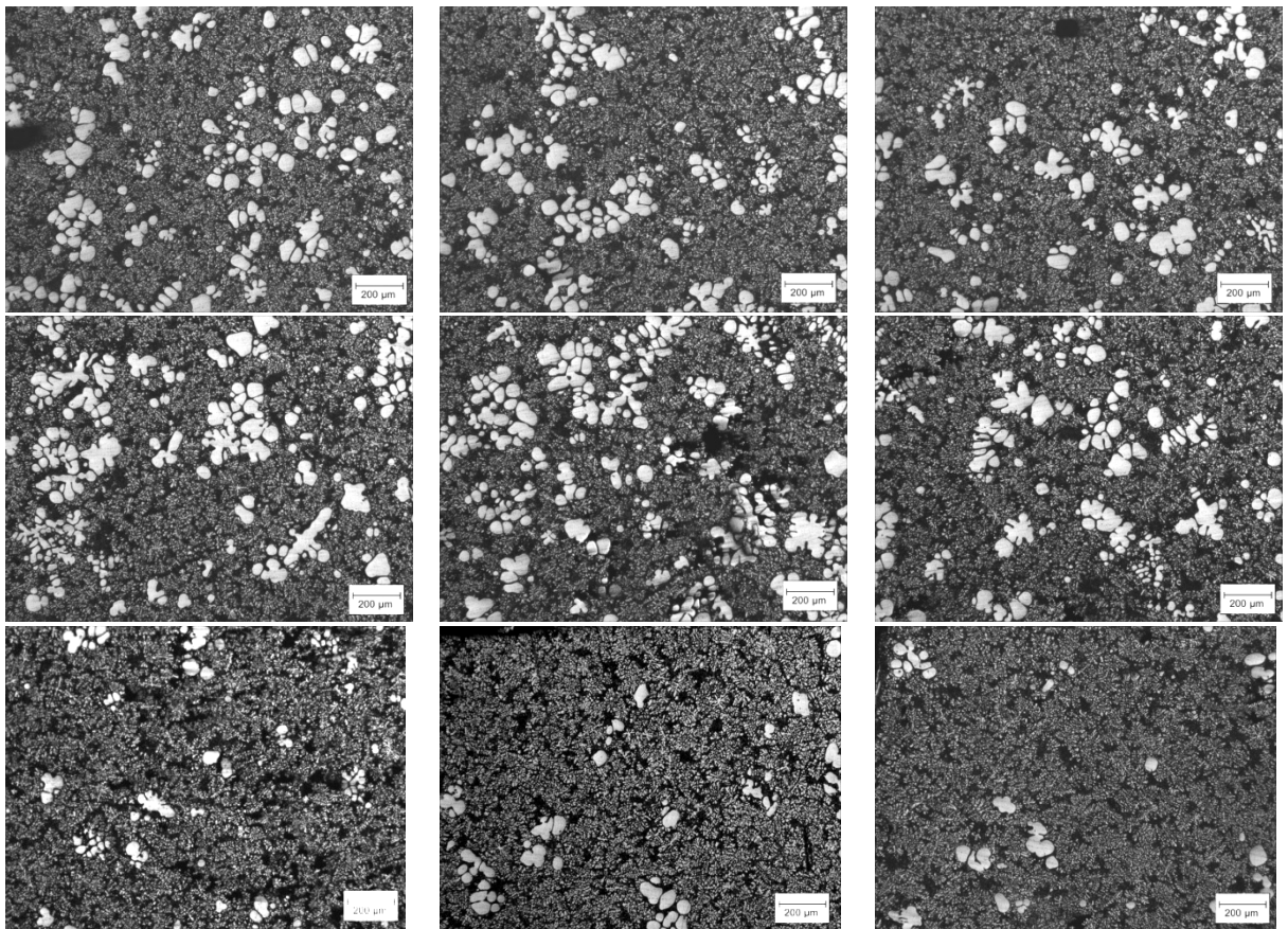
รูปที่ 3-7 โครงสร้างจุลภาคหลังจากจุ่มแท่งกราไฟต์เป็นเวลา 60 วินาที (50x)
