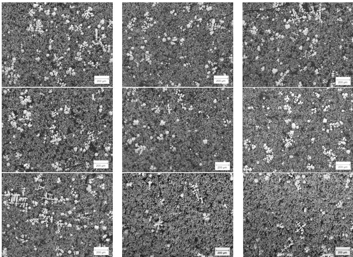
รูปที่ 3-5 โครงสร้างจุลภาคหลังจากจุ่มแท่งกราฟไฟต์เป็นเวลา 20 วินาที (50x)
