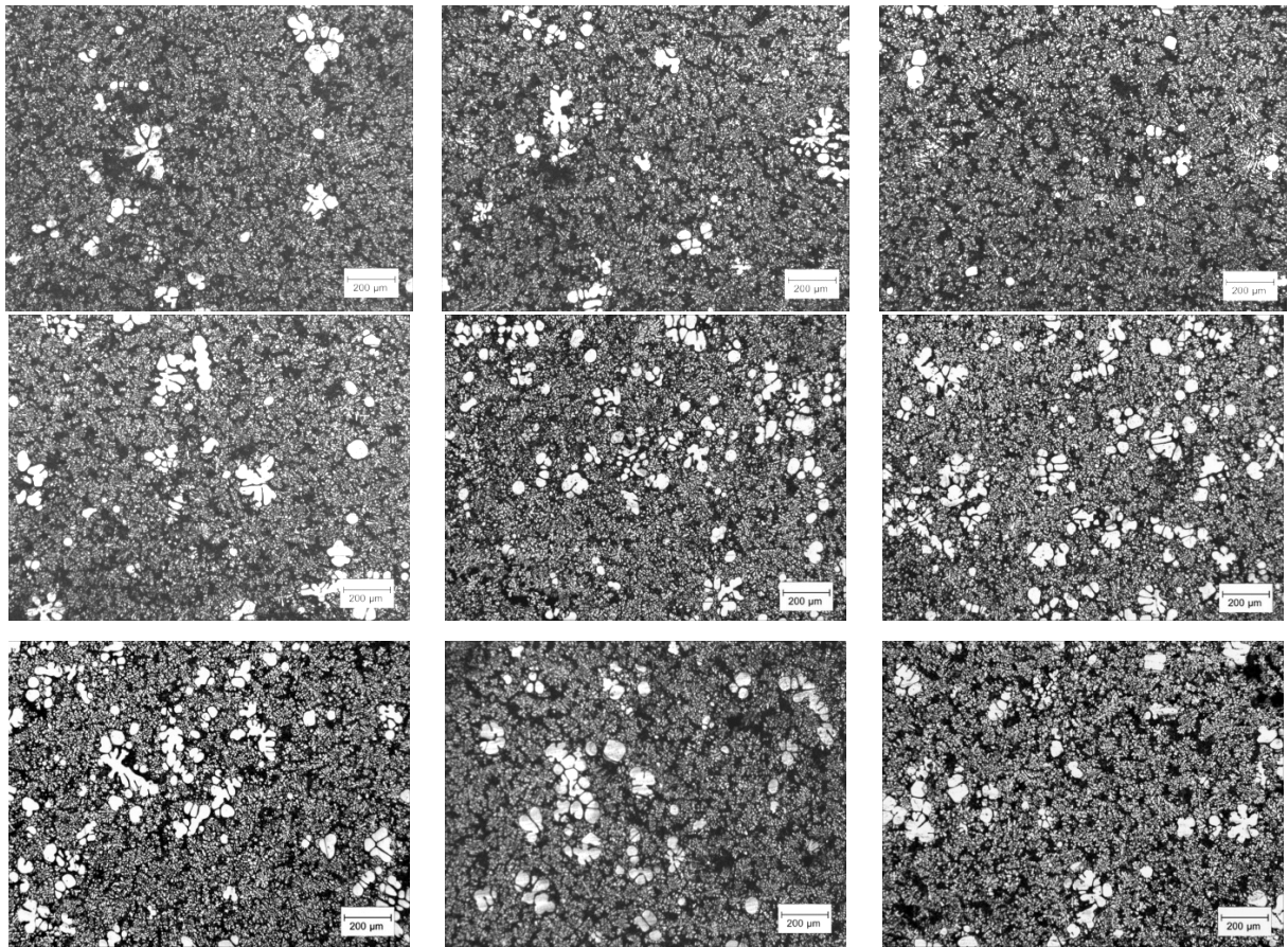
รูปที่ 3-6 โครงสร้างจุลภาคหลังจากจุ่มแท่งกราไฟต์เป็นเวลา 28 วินาที (50x)
