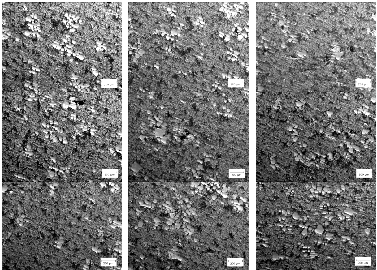
รูปที่ 3-19 โครงสร้างจุลภาคหลังจากจุ่มแท่งกราไฟต์เป็นเวลา 60 วินาที ส่วนล่าง (50x)
