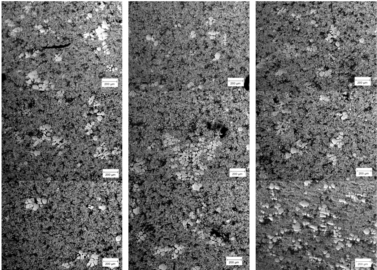
รูปที่ 3-18 โครงสร้างจุลภาคหลังจากจุ่มแท่งกราไฟต์เป็นเวลา 60 วินาที ส่วนบน (50x)
