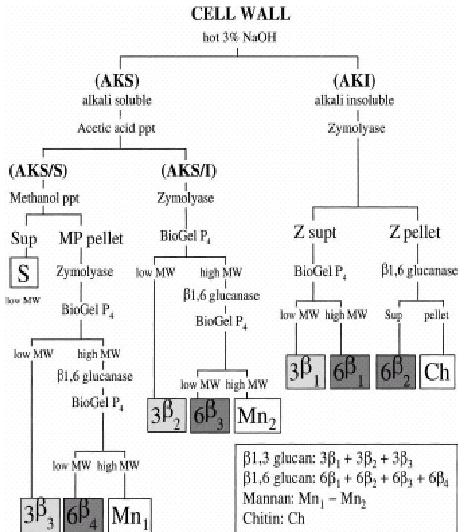
ภาพที่ 5 ลำดับขั้นการแยกองค์ประกอบผนังเซลล์ด้วยการสกัดด้วยกรดและด่าง ที่มา: Magnelli และคณะ (2002)
