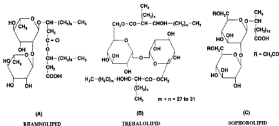
ภาพที่ 1 โครงสร้างของไกลโคไลปิดที่ใช้ในอุตสาหกรรม
