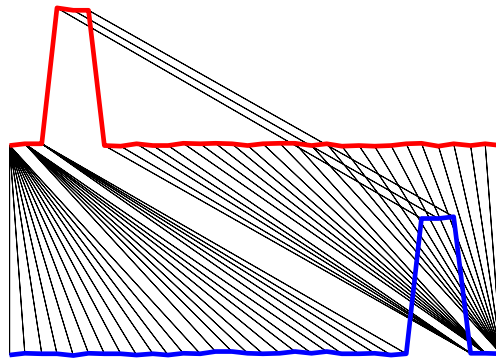
รูปที่ 2.2 การปรับแนวในการหาระยะทางอย่างที่ไม่เหมาะสมของวิธีไดนามิกโทมวอร์ปิ้ง [14]
