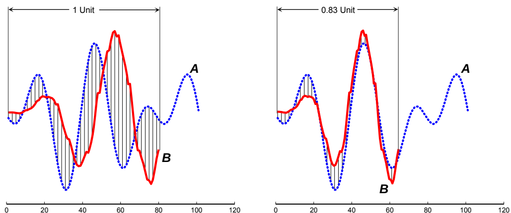
รูปที่ 2.5 การคำนวณค่าระยะทางด้วยวิธีการปรับขนาดเอกรูป
