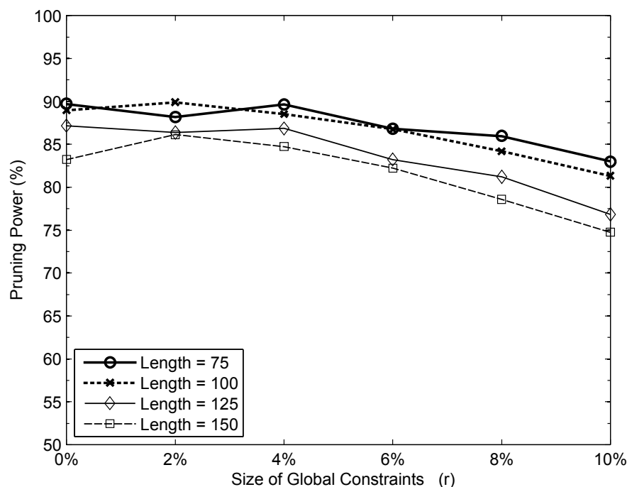
รูปที่ 4.2 ความสามารถในการลดปริมาณข้อมูลที่จะต้องคำนวณค่าระยะทางจริงของข้อมูลสอบถามที่มีความยาว และความกว้างของเงื่อนไขบังคับโดยรวมแบบซิกโม-ซิบะที่ขนาดต่าง ๆ
