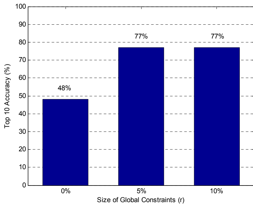
รูปที่ 4.5 เปรียบเทียบความแม่นยำในการค้นหาเพลง 10 ลำดับแรก เมื่อความกว้างของเงื่อนไข บังคับโดยรวมแบบซิกโมอิดมีขนาดต่าง ๆ
