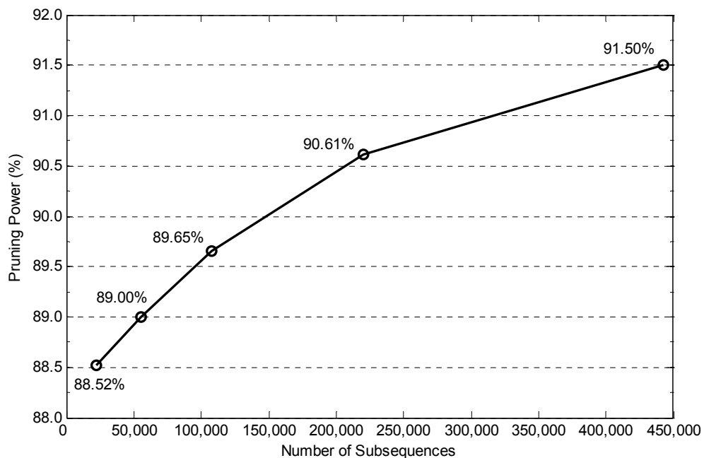
รูปที่ 4.3 ความสามารถในการลดปริมาณข้อมูลที่ต้องคำนวณค่าระยะทางจริง เมื่อฐานข้อมูลมีขนาดต่าง ๆ
