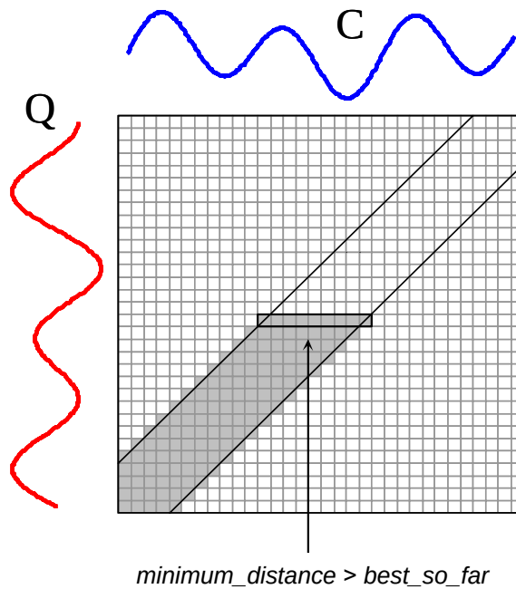
รูปที่ 3.7 วิธีการหยุดคำนวณในตอนต้นของวิธีไดนามิกโปรแกรมมิ่ง ถ้าค่าระยะทางน้อยสุดในแถวมีค่ามากกว่าค่า best_so_far ให้หยุดการคำนวณระยะทางดังกล่าวทันที
