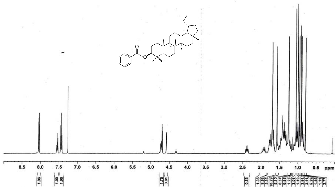
รูป 26 ^1\text{H-NMR} สเปกตรัมของ lupeol benzoate (400 MHz) ใน \text{CDCl}_3
