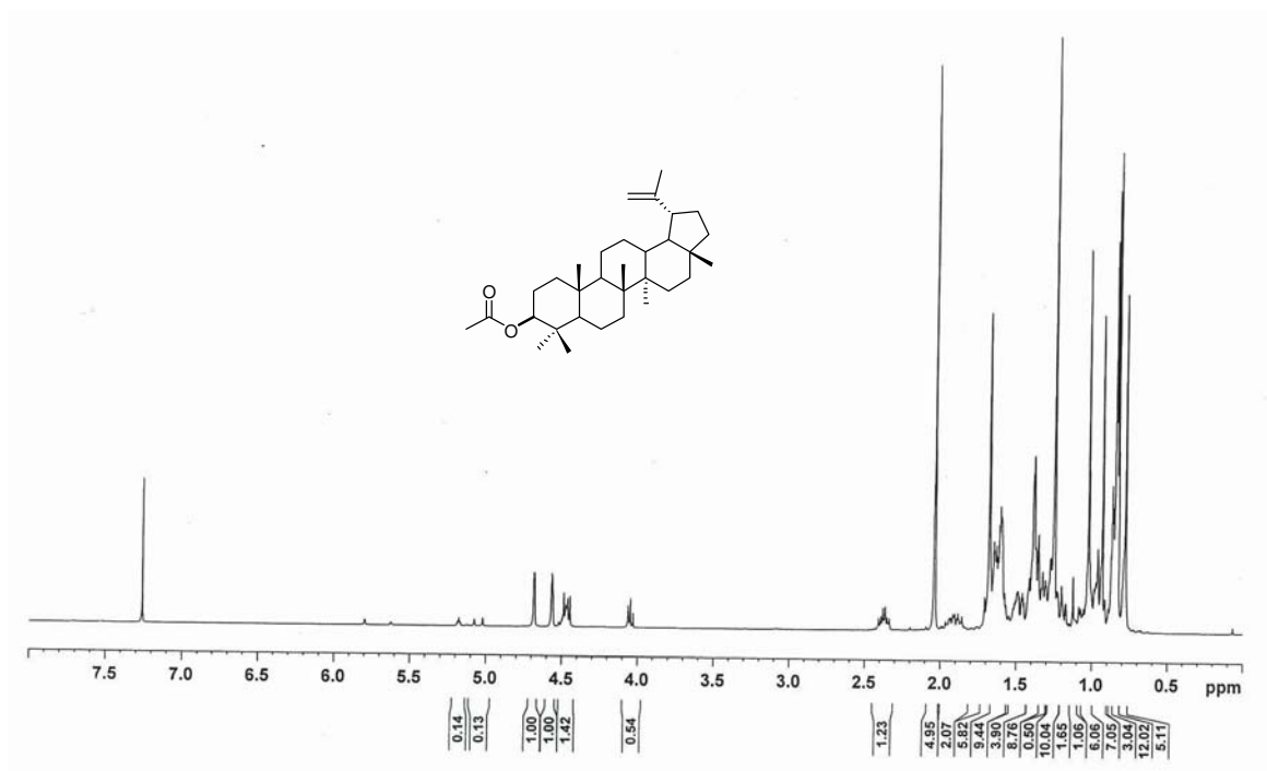
รูป 20 1 H-NMR สเปกตรัมของ lupeol acetate (400 MHz) ใน CDCl 3
