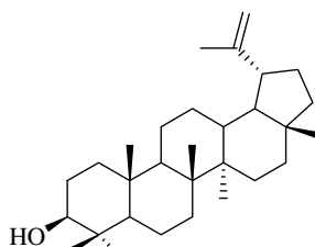
lupeol (4)
