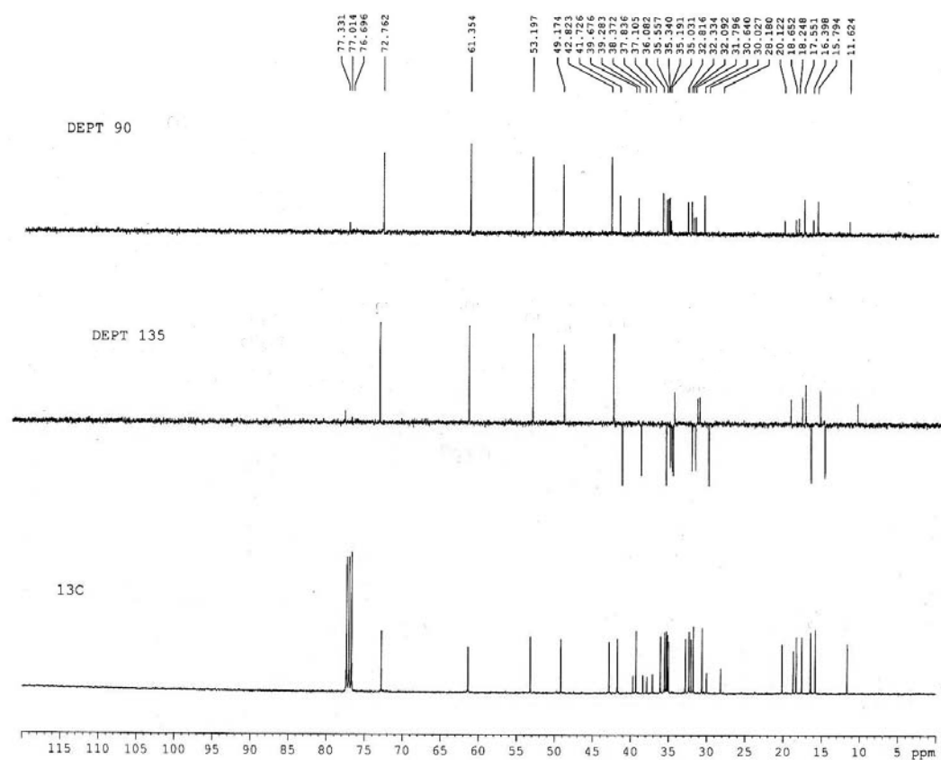
รูป 10 ^{13}\text{C} , DEPT135, DEPT90 NMR สเปกตรัมของ 3 \alpha -friedelanol (100 MHz) ใน \text{CDCl}_3
