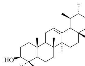
\alpha -Amyrin (5)
