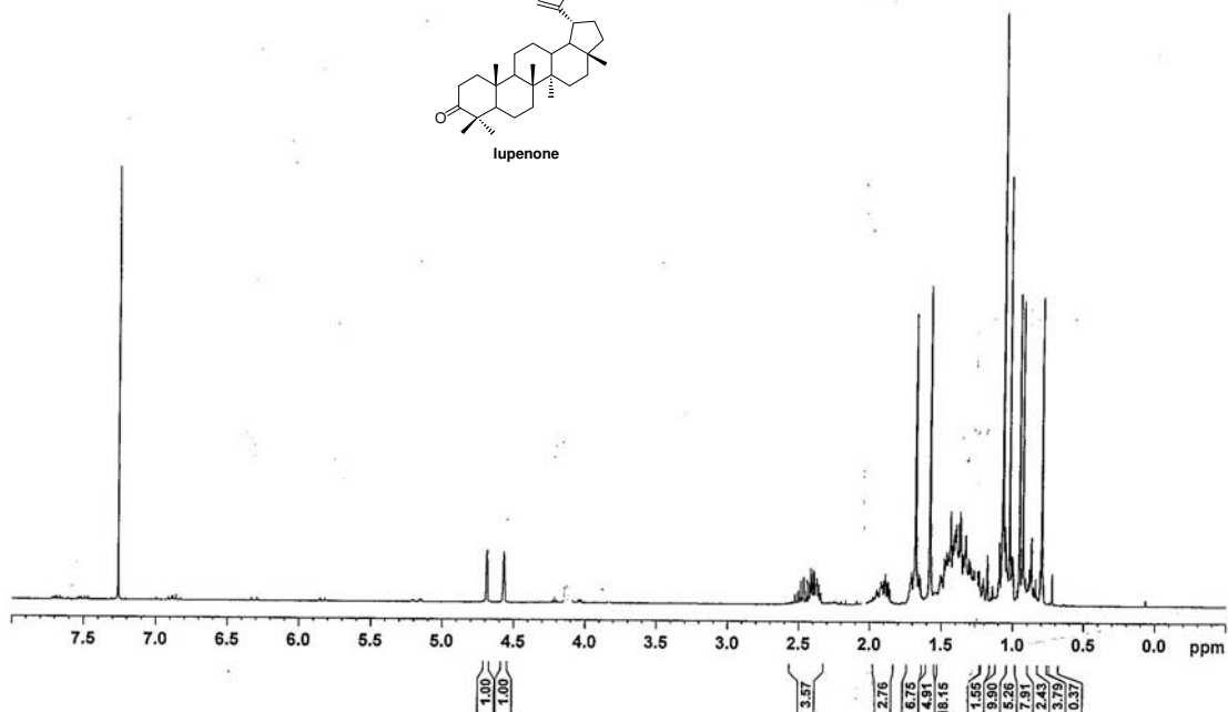
รูป 1 ^1\text{H-NMR} สเปกตรัมของ lupenone (400 MHz) ใน \text{CDCl}_3
