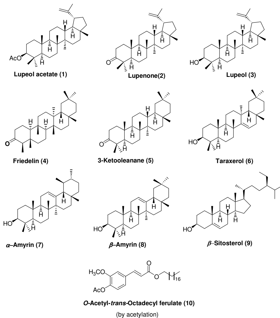
รูป 9 โครงสร้างของสารที่เป็นองค์ประกอบในสารสกัด AMH-R
