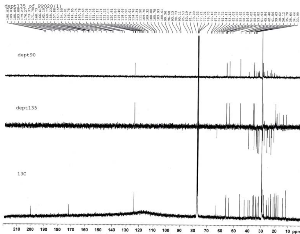
รูป 33 13 C, Dept135 NMR สเปกตรัมของ stigmast-4-ene-3-one (100 MHz) ใน CDCl 3
