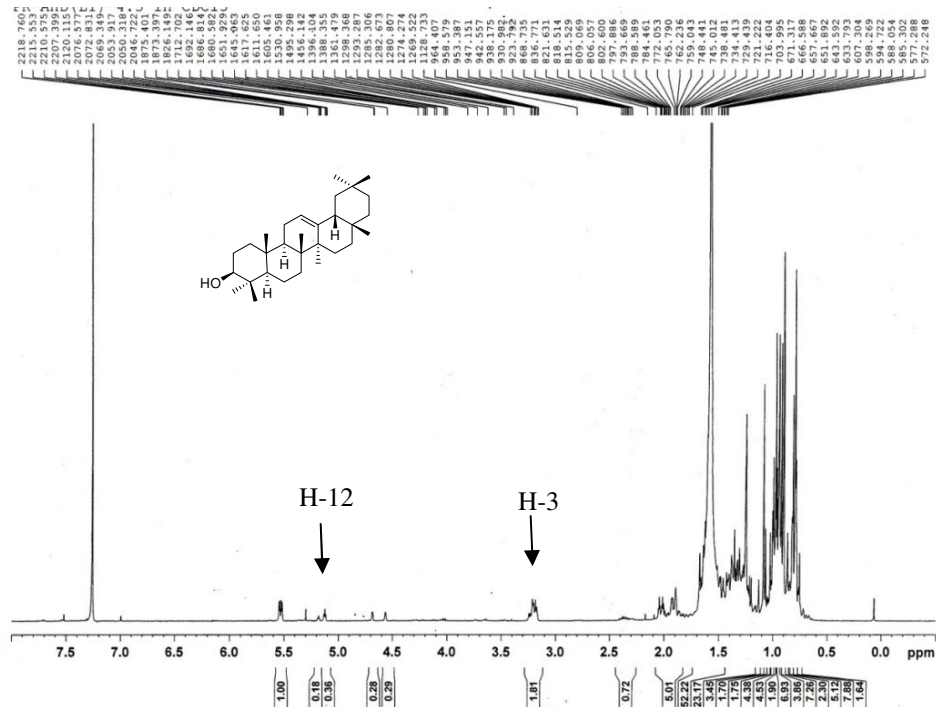
รูป 18 ^1\text{H-NMR} สเปกตรัมของ \beta -amyrin (องค์ประกอบรอง) (400 MHz) ใน \text{CDCl}_3
