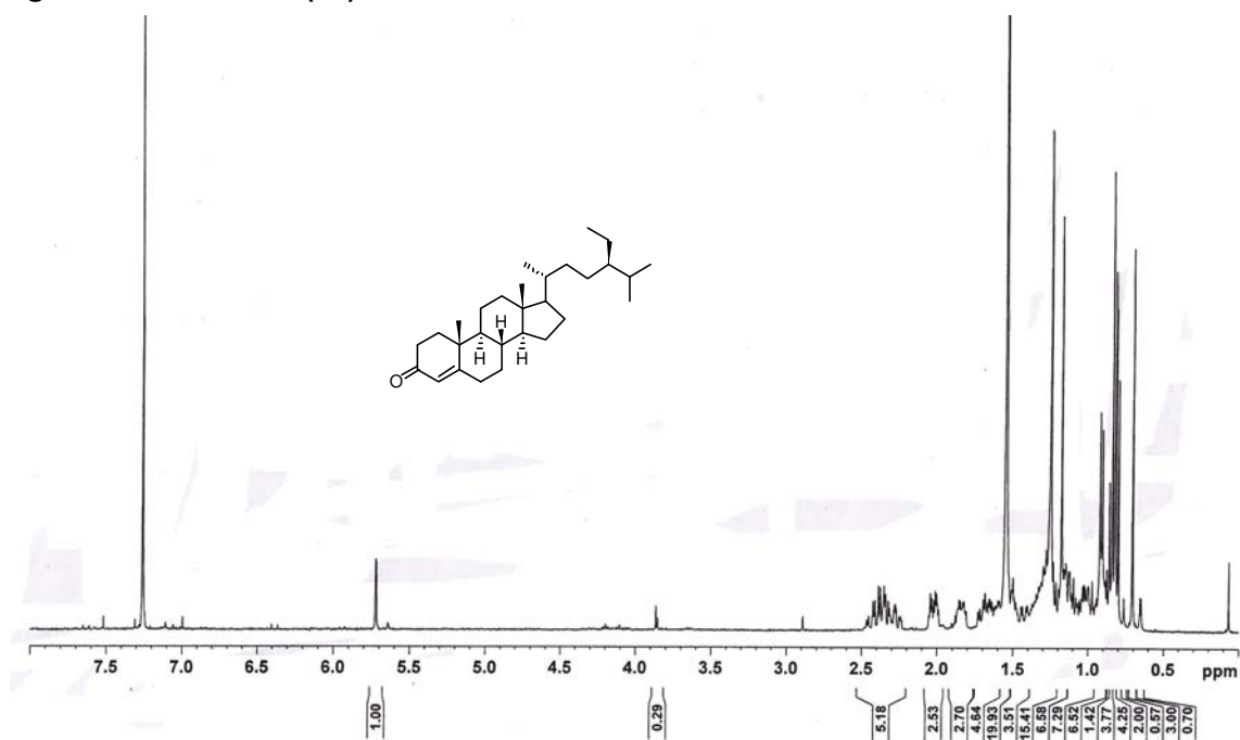
รูป 32 1 H-NMR สเปกตรัมของ stigmast-4-ene-3-one (400 MHz) ใน CDCl 3
