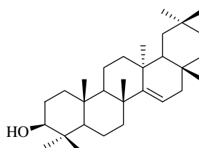
taraxerol (7)
