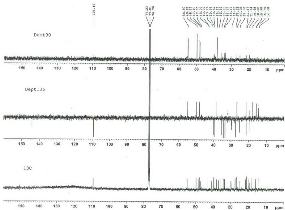
รูป 2 ^{13}\text{C} , Dept135, Dept90 NMR สเปกตรัมของ lupenone (100 MHz) ใน \text{CDCl}_3
