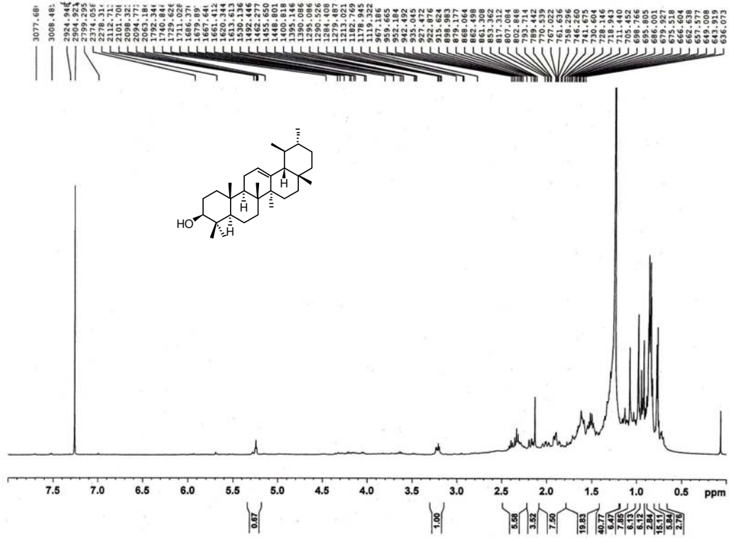
รูป 17 ^1\text{H-NMR} สเปกตรัมของ \alpha -amyrin (400 MHz) ใน \text{CDCl}_3
