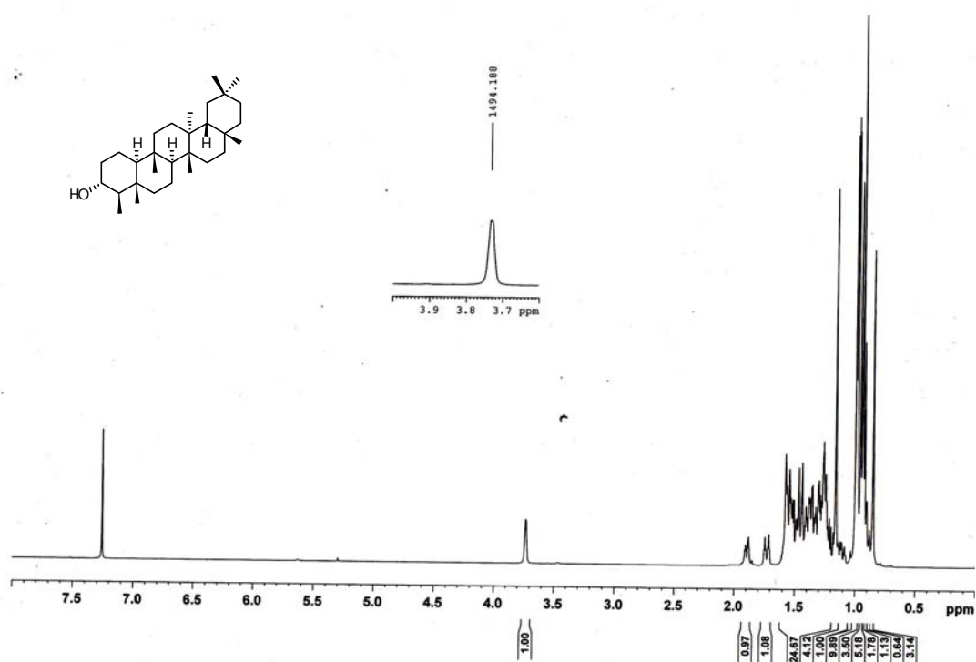
รูป 9 ^1\text{H} -NMR สเปกตรัมของ 3 \alpha -friedelanol (400 MHz) ใน \text{CDCl}_3
