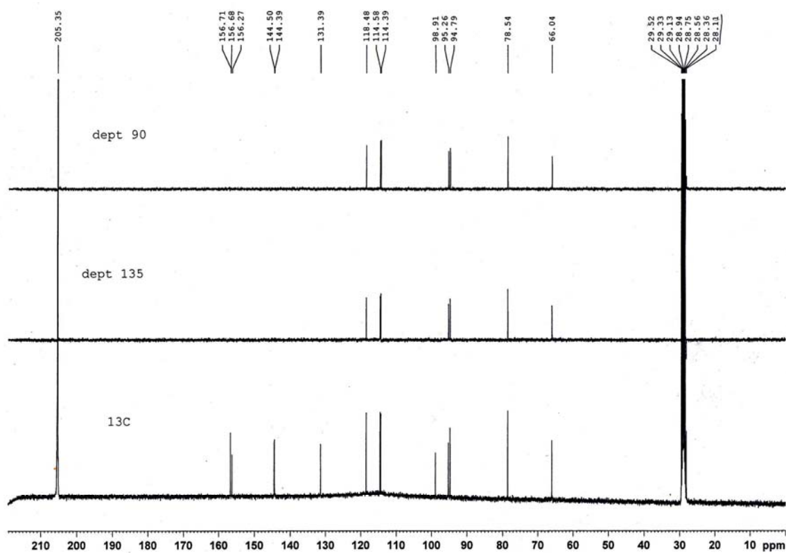
รูป 47 ^{13}\text{C} , DEPT 135, DEPT 90 สเปกตรัมของ epicatechin (100 MHz) ใน \text{acetone-}d_6
