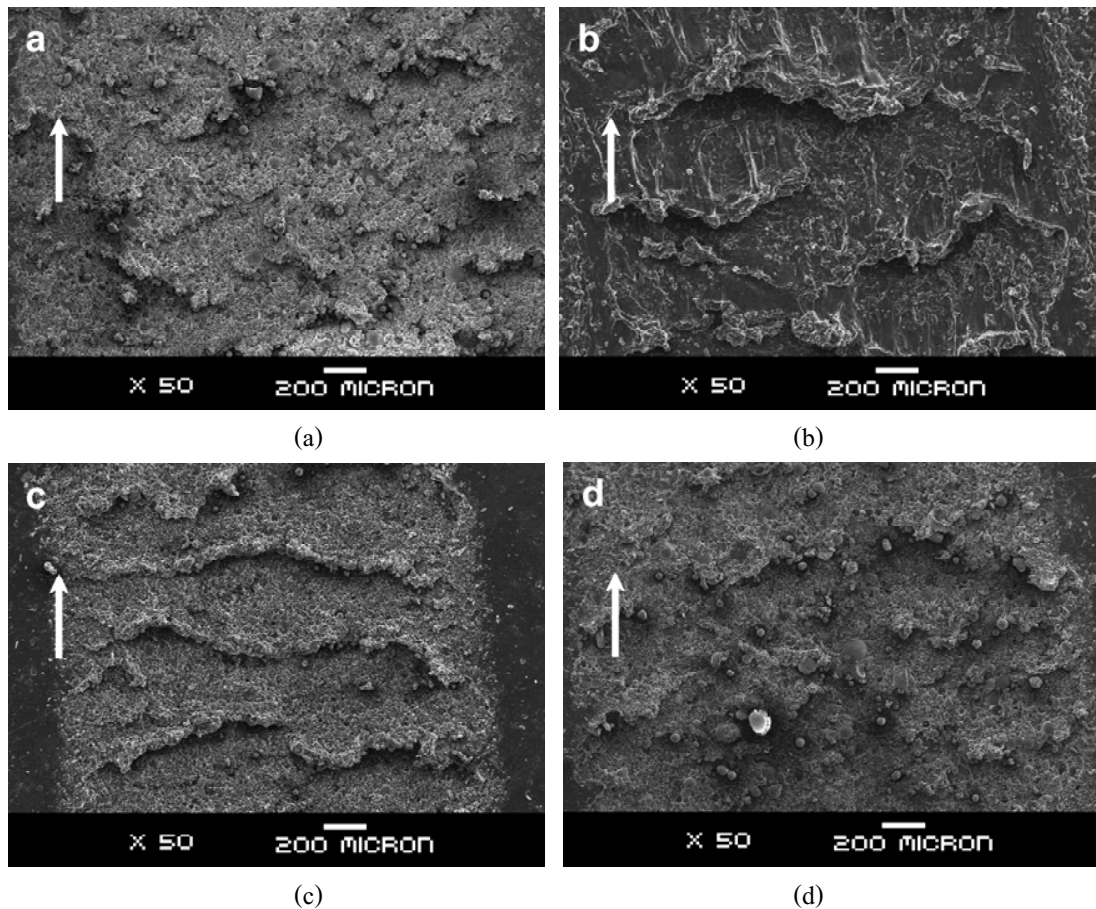
รูปที่ 30 ภาพ SEM ของผิวที่สึกหรอของยางธรรมชาติที่เติมซิลิกาถูกผสม FASi/PSi ปริมาณ 40 phr ลูกศรแสดงทิศทางการเคลื่อนผ่านของลูกบอลเหล็กบนชิ้นงานยางขณะทดสอบ
