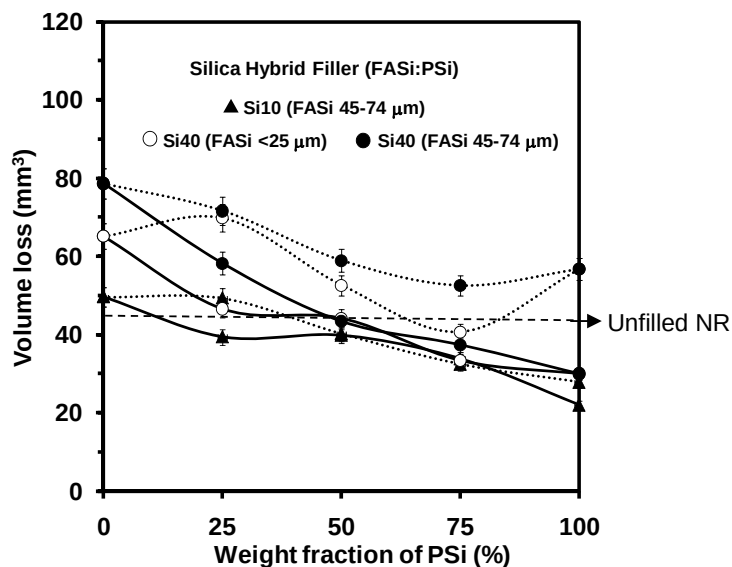
รูปที่ 24 กราฟแสดงความสัมพันธ์ระหว่างปริมาณยางที่สูญเสียไปกับสัดส่วนพรีซิพิเตตซิลิกาของซิลิกา
