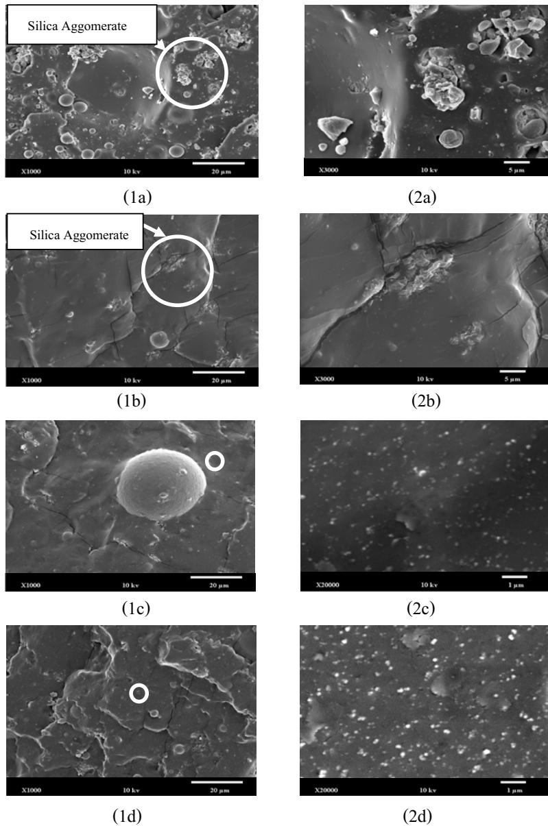
รูปที่ 20 ลักษณะสัณฐานวิทยาของยางธรรมชาติที่เติมซิลิกาลูกผสมระหว่างเถ้าลอยและพรีซิปิเตชันซิลิกาใน ปริมาณ 40 phr
