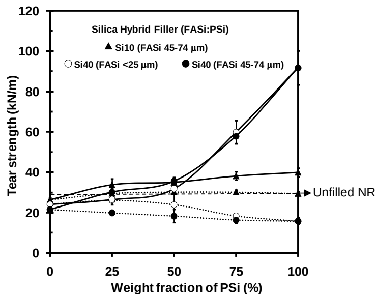
รูปที่ 22 กราฟแสดงความสัมพันธ์ระหว่างความทนแรงฉีกขาดกับสัดส่วนพรีซิพิตชันซิลิกาของซิลิกาถูกผสม FASi/PSi ในยางธรรมชาติ
