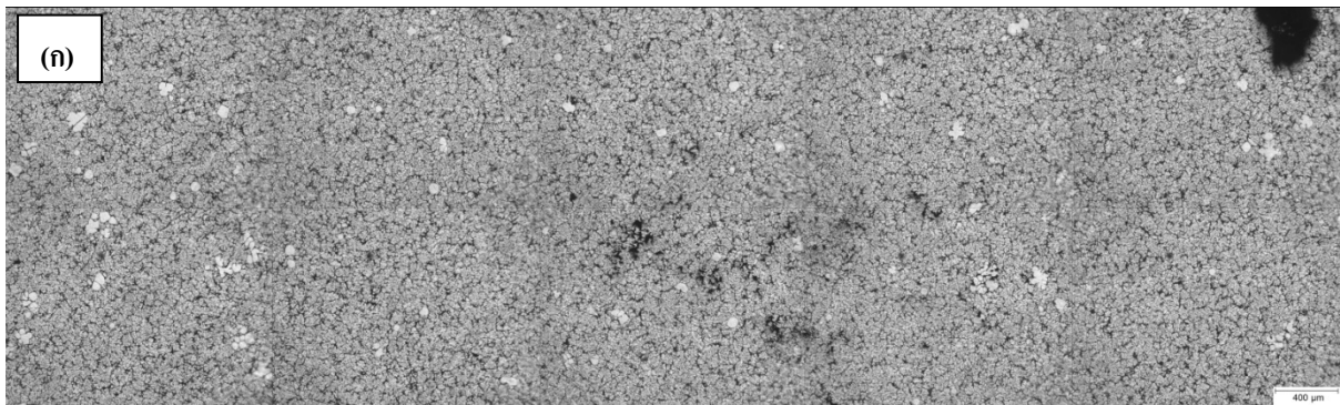
รูปที่ 3 - 61แสดงโครงสร้างจุลภาคที่อุณหภูมิแห้งแ่งไฟต์ 200°C จุ่มแ่งไฟต์เป็นเวลา 20วินาที (ก) ส่วนบน (ข) ส่วนกลาง และ (ค) ส่วนล่าง
