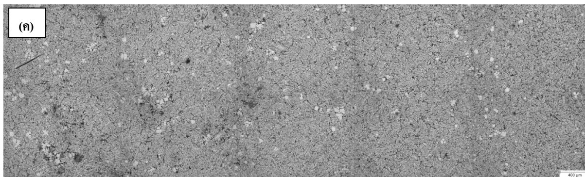
รูปที่ 3 - 62 แสดงโครงสร้างจุลภาคที่อุณหภูมิแห้งแกรไฟต์ 300°C จุ่มแห้งแกรไฟต์เป็นเวลา 20 วินาที (ก) ส่วนบน (ข) ส่วนกลาง และ (ค) ส่วนล่าง
