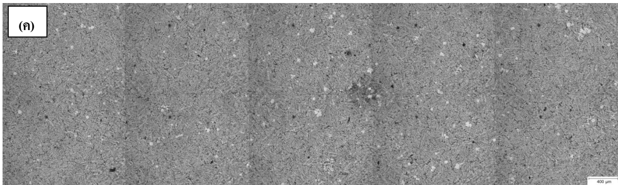
รูปที่ 3 - 57แสดงโครงสร้างจุลภาคที่อุณหภูมิแท่งแกรไฟต์ 200°C จุ่มแท่งแกรไฟต์เป็นเวลา 10วินาที (ก) ส่วนบน (ข) ส่วนกลาง และ (ค) ส่วนล่าง
