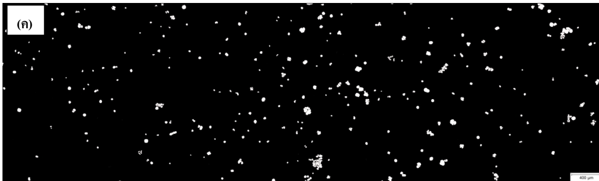
รูปที่ 3 - 69แสดงโครงสร้างจุลภาคที่อุณหภูมิแท่งแกรไฟต์ 200°C จุ่มแท่งแกรไฟต์เป็นเวลา 10วินาที
