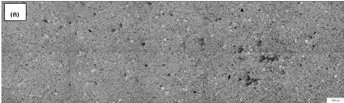
รูปที่ 3 - 58 แสดงโครงสร้างจุลภาคที่อุณหภูมิแห้งแกรไฟต์ 300°C จุ่มแห้งแกรไฟต์เป็นเวลา 10 วินาที (ก) ส่วนบน (ข) ส่วนกลาง และ (ค) ส่วนล่าง
