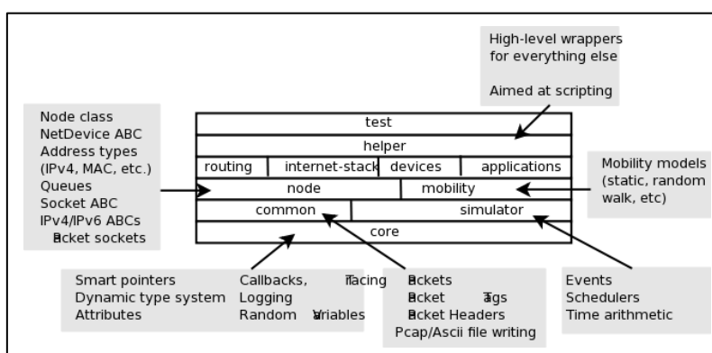
รูปที่ 4-6 รูปแบบของส่วนจำเพาะของโปรแกรมจำลองเครือข่าย NS-3 [24]
