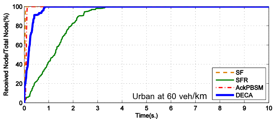
รูปที่ 2-13 กราฟแสดงความเร็วในการกระจายข้อมูลบนถนนในเมืองที่ความหนาแน่นแตกต่างกัน
