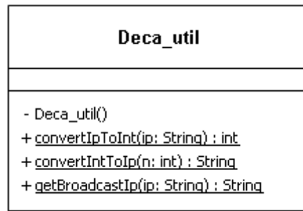
รูปที่ 5-22 รายละเอียดของ Class Deca_util
