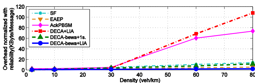
รูปที่ 3-25 ผลการทดลองค่าใช้จ่าย
