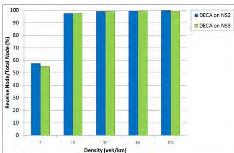
รูปที่ 4-13 ผลการทดลองค่าความเชื่อถือได้
