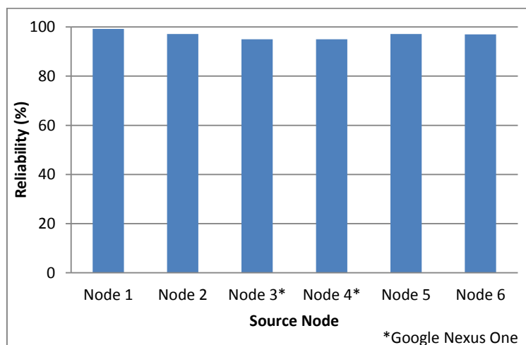
รูปที่ 5-41 ผลการทดลองค่าความเชื่อได้ของโหนดต้นทางแต่ละโหนด
