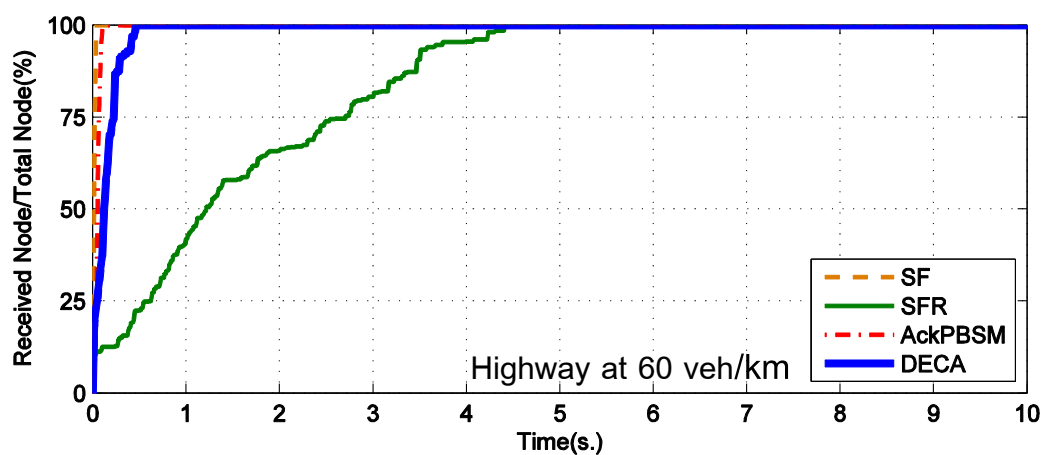
รูปที่ 2-12 กราฟแสดงความเร็วในการกระจายข้อมูลบนถนนทางหลวงที่ความหนาแน่นแตกต่างกัน
