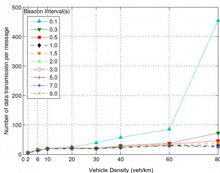
รูปที่ 2-1 กราฟแสดงจำนวนการส่งข้อความในช่วงเวลาการทำบีมคอนต่างกัน
