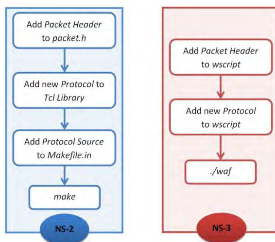
รูปที่ 4-9 การเพิ่มโปรโตคอลใหม่บนโปรแกรมจำลองเครือข่าย NS-2 และ NS-3
