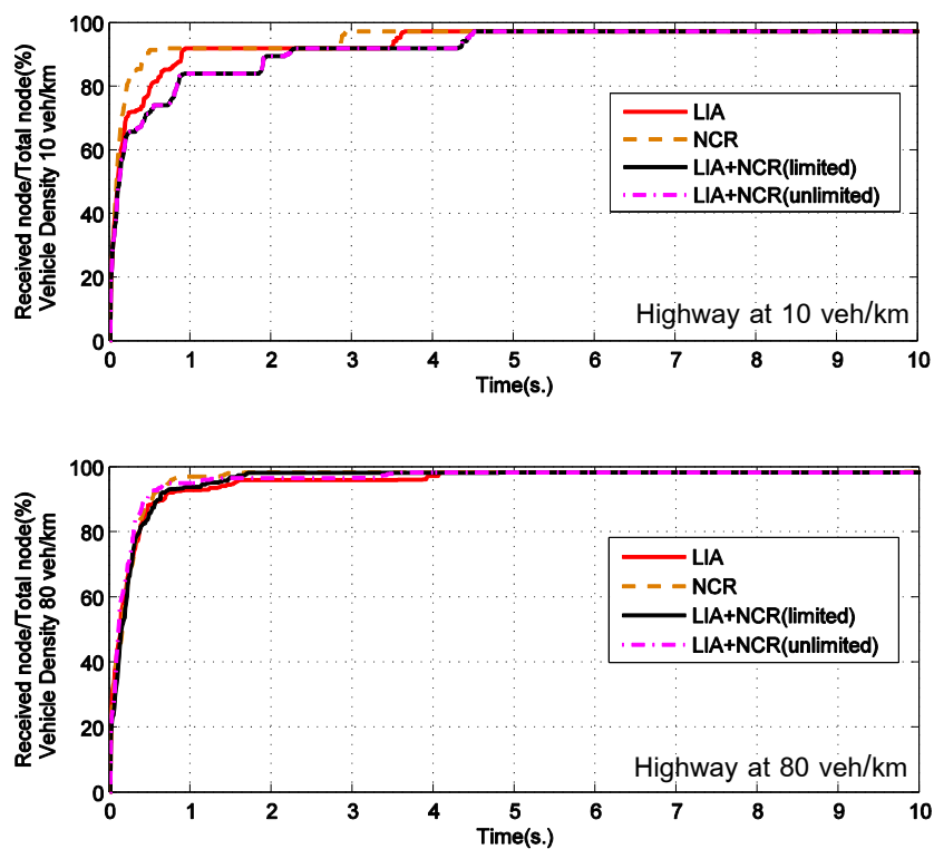
รูปที่ 3-7 ผลการทดลองความเร็วของการกระจายข้อมูลบนถนนทางหลวงโดยใช้วิธี LIA+NCR
