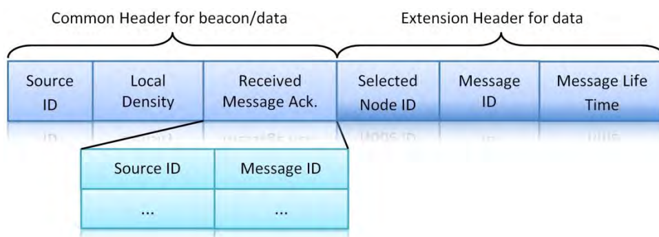
รูปที่ 3-22 โครงสร้างบิตคอนของโปรโตคอล DECA
