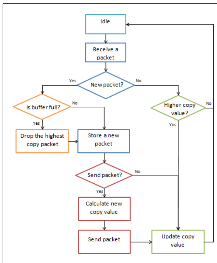
รูปที่ 3-11 แผนภาพแสดงการทำงานของนโยบายการทิ้งข้อมูล
