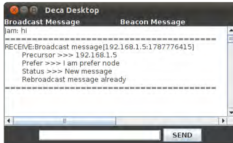
รูปที่ 5-34 ผลการทดลองการกระจายข้อมูลซ้ำทันทีเมื่อโหนดถูกเลือกให้เป็นโหนดส่งต่อข้อความ
