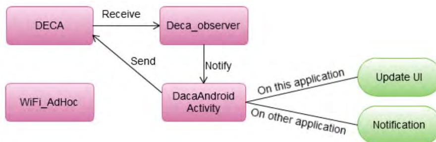
รูปที่ 5-23 การทำงานระหว่างแอปพลิเคชันแอนดรอยด์กับโปรโตคอล DECA
