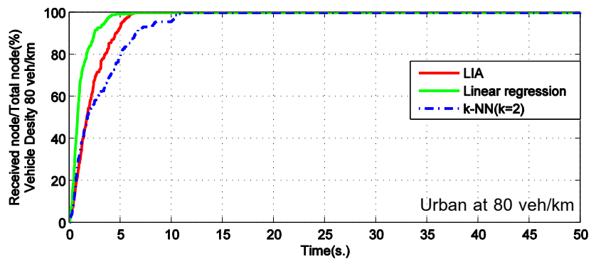
รูปที่ 3-6 ผลการทดลองความเร็วของการกระจายข้อมูลบนถนนในเมือง โดยใช้วิธี Linear regression และ K-Nearest Neighbor
