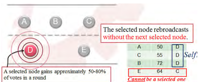
รูปที่ 4-25 ปัญหาการเลือกตัวเองเป็นผู้กระจายข้อมูลลำดับถัดไป
