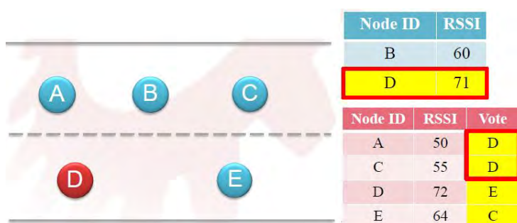
รูปที่ 4-21 สรุปผลการเลือกโหนดของขั้นตอนการโหวตแบบอาร์เอสเอสไอ
