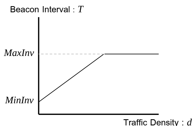
รูปที่ 2-2 กราฟแสดงการคำนวณช่วงเวลาปรับตัวแบบเชิงเส้น
