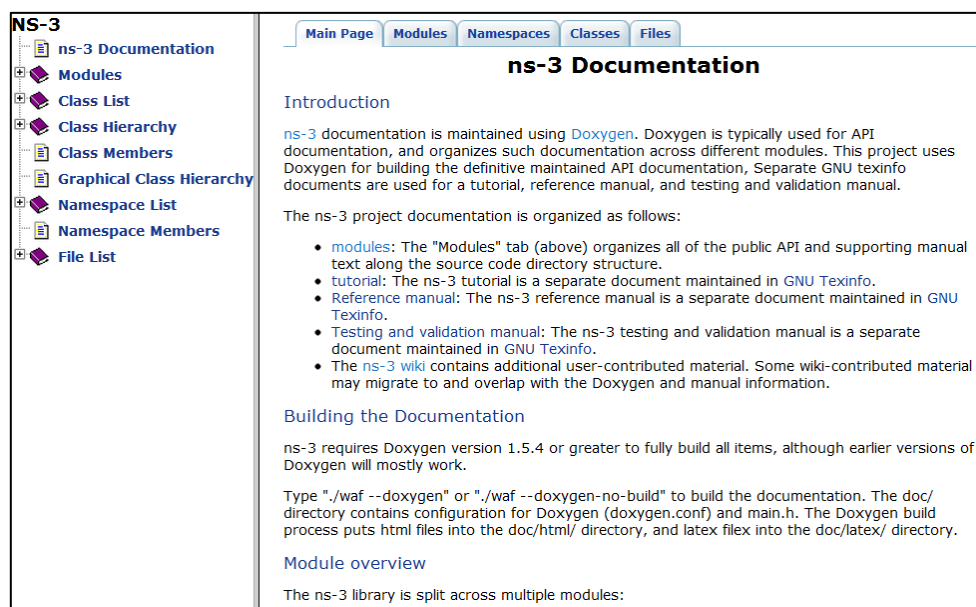
รูปที่ 4-1 ตัวอย่างเอกสารประกอบ API ของโปรแกรมจำลองเครือข่ายเวอร์ชัน 3 [23]
