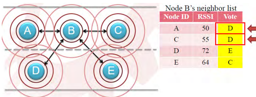
รูปที่ 4-19 ขั้นตอนที่สองของขั้นตอนการโหวตแบบอาร์เอสเอสไอ
