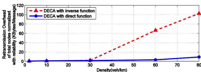
รูปที่ 3-21 กราฟแสดงผลการทดลองค่าใช้จ่ายจากการกระจายข้อความซ้ำด้วยการคำนวณเวลาที่แตกต่างกัน
