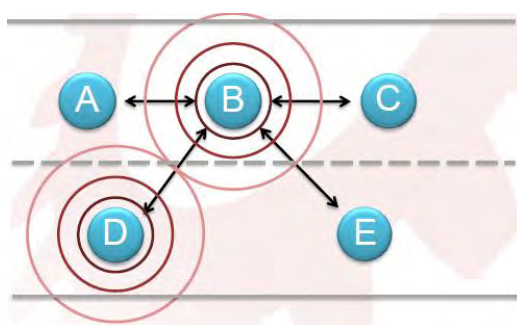
รูปที่ 4-20 ขั้นตอนที่สามของอัลกอริทึมการโหวตแบบอาร์เอสเอสไอ
