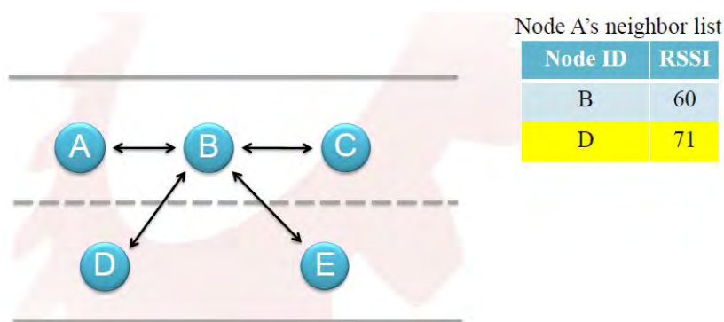
รูปที่ 4-18 ขั้นตอนหนึ่งของขั้นตอนการโหวตแบบอาร์เอสเอสไอ
