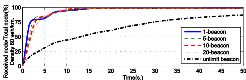
ค) ความเร็วในการกระจายที่ความหนาแน่น 60 คัน/กม.
