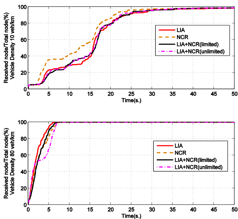
รูปที่ 3-8 ผลการทดลองความเร็วของการกระจายข้อมูลบนถนนในเมืองโดยใช้วิธี LIA+NCR
