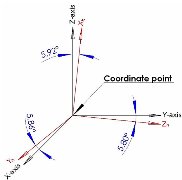
ภาพผนวกที่ ค4 องศาของมุมที่เปลี่ยนแปลงไปจากทิศทางการสั่นสะเทือนในรถไฟใต้ดินตาม
