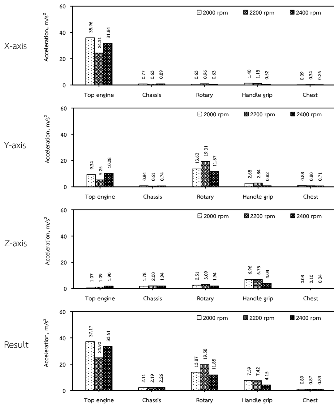
ภาพที่ 58 ค่าความเร่งของการสั่นสะเทือนของรถไถเดินตามล้อเหล็กเงื่อนไขไฟฟ้าพวณดินเที่ยวที่ 2 ด้วยใบมีดจอบหมุนญี่ปุ่นรูปตัวซี 14 ใบ
