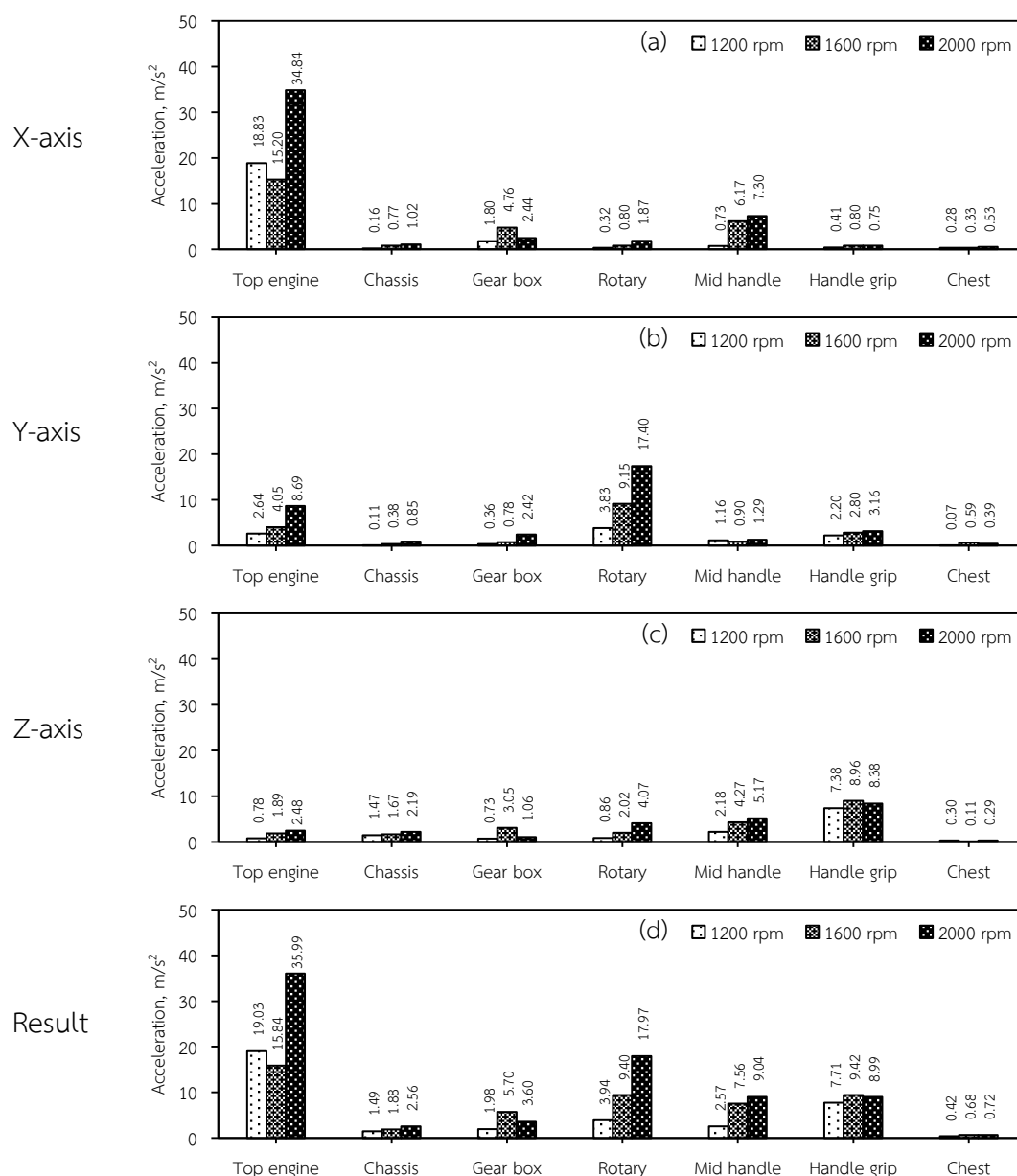
ภาพที่ 51 ค่าความเร่งของการสั่นสะเทือนที่ของรถไถเดินตามล้อเหล็กที่เงื่อนไขการเคลื่อนที่บนแปลงเกษตรกรรม
