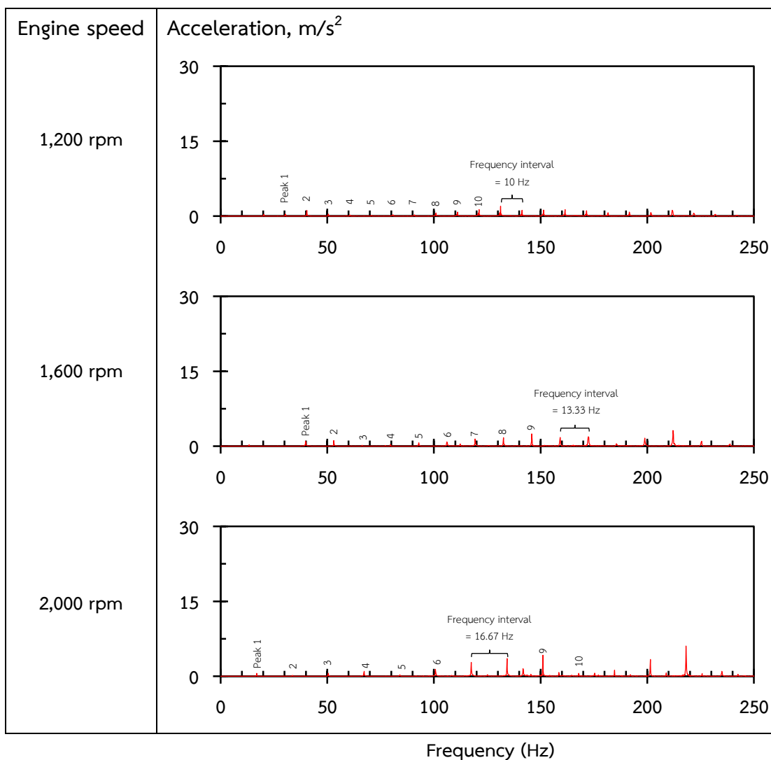
ภาพที่ 36 สเปกตรัมของการสั่นสะเทือนในแนวตั้ง (Z-axis) ที่ตำแหน่งผิวบนเครื่องยนต์ กรณียรถไถเดินตามล้อเหล็กเงื่อนไขไม่เคลื่อนที่
