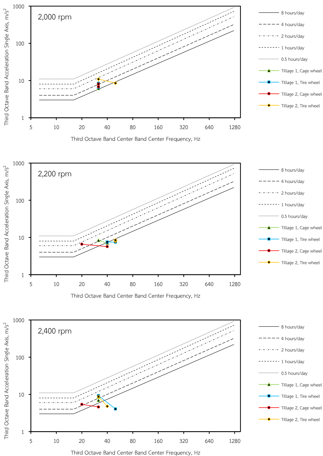
ภาพที่ 73 ค่ามาตรฐานความสั่นสะเทือนที่มือตามข้อเสนอแนะของ ANSI เครื่องไถพรวนดินด้วยใบมีดจอบหมุนต้นแบบ 14 ใบ
