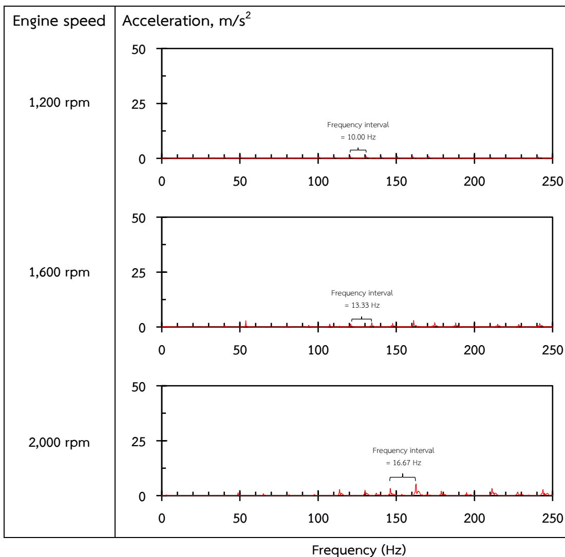
ภาพที่ 49 สเปกตรัมของการสั่นสะเทือนในแนวดิ่ง (Z-axis) ที่ตำแหน่งพืบนเครื่องยนต์ กรณีรถไถเดินตามล้อเหล็กเงื่อนไขการเคลื่อนที่บนแปลงเกษตรกรรม
