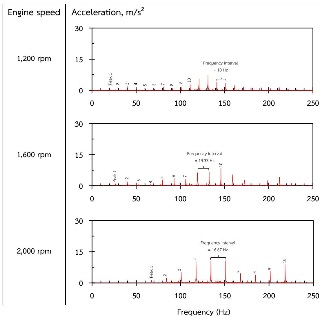
ภาพที่ 35 สเปกตรัมของการสั่นสะเทือนในแนวขวางของรถไถเดินตาม (Y-axis) ที่ตำแหน่งพืวบนเครื่องยนต์ กรณีรถไถเดินตามล้อเหล็กเงื่อนไขไม่เคลื่อนที่
