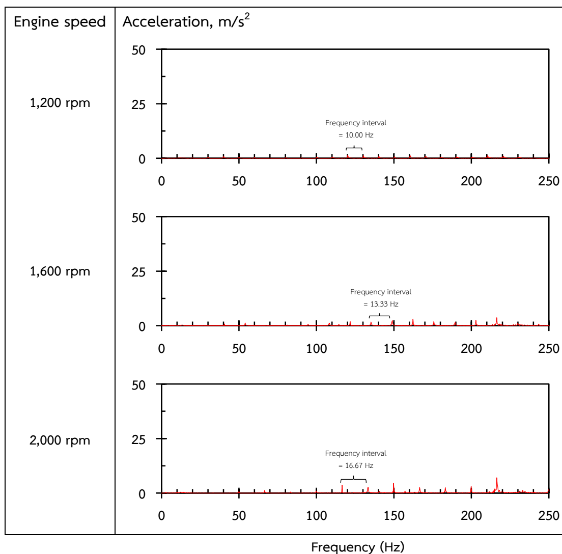
ภาพที่ 43 สเปกตรัมของการสั่นสะเทือนในแนวตั้ง (Z-axis) ที่ตำแหน่งผิวบนเครื่องยนต์ กรณีรถไถเดินตามล้อเหล็กเงื่อนไขการเคลื่อนที่บนถนนลาดยาง
