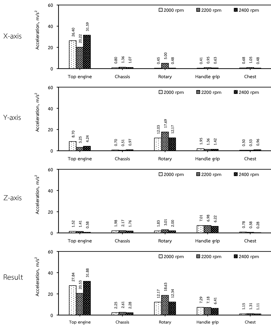
ภาพที่ 63 ค่าความเร่งของการสั่นสะเทือนของรถไถเดินตามล้อยางเงื่อนไขไถพรวนดินเดี่ยวที่ 1 ด้วยใบมีดจอบหมุนต้นแบบ 14 ใบ
