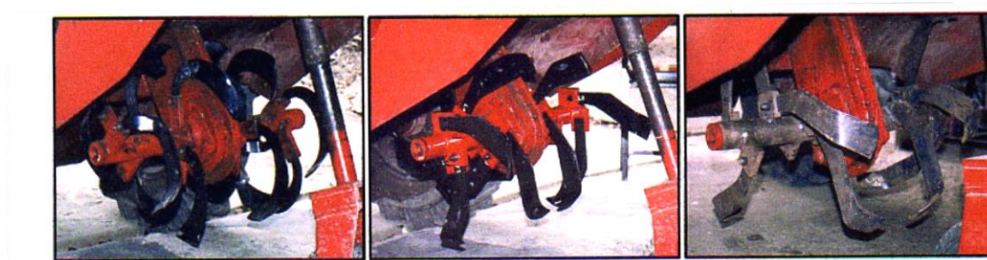
ภาพที่ 27 ลักษณะการติดตั้งไบมีดจอบหมุนกับเพลารถไถพรวนจอบหมุน
