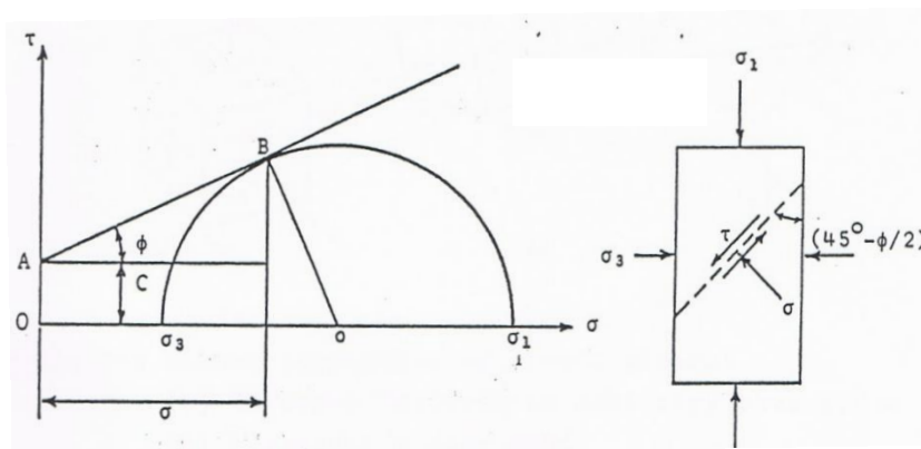
ภาพที่ 23 Coulomb's model แสดงระนาบวิบัติเฉือน
