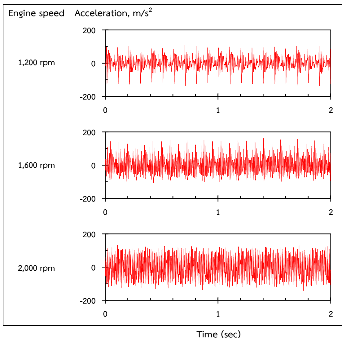
ภาพที่ 31 สัญญาณการสั่นสะเทือนในแนวการเคลื่อนที่ของรถไถเดินตาม (X-axis) ที่ตำแหน่งผิวบนเครื่องยนต์ กรณีรถไถเดินตามล้อหลักเงื่อนไขไม่เคลื่อนที่
