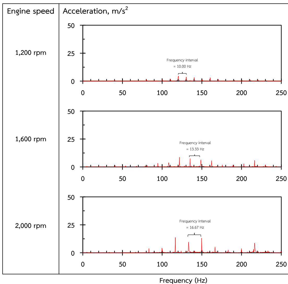
ภาพที่ 42 สเปกตรัมของการสั่นสะเทือนในแนวขวางของรถไถเดินตาม (Y-axis) ที่ตำแหน่งพืบบนเครื่องยนต์ กรณีรถไถเดินตามล้อหลักเงื่อนไขการเคลื่อนที่บนถนนลาดยาง
