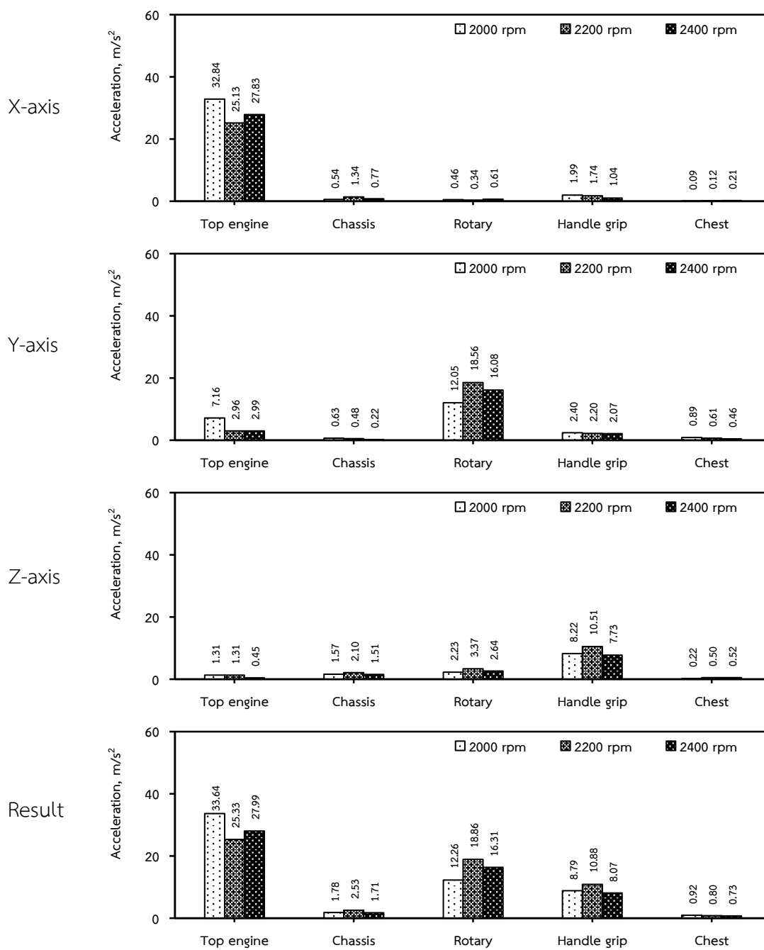
ภาพที่ 68 ค่าความเร่งของการสั่นสะเทือนของรถไถเดินตามล้อยางเอนไซไกวพรุนดินเที่ยวที่ 2 ด้วยใบมีดจอบหมุนต้นแบบ 10 ใบ
