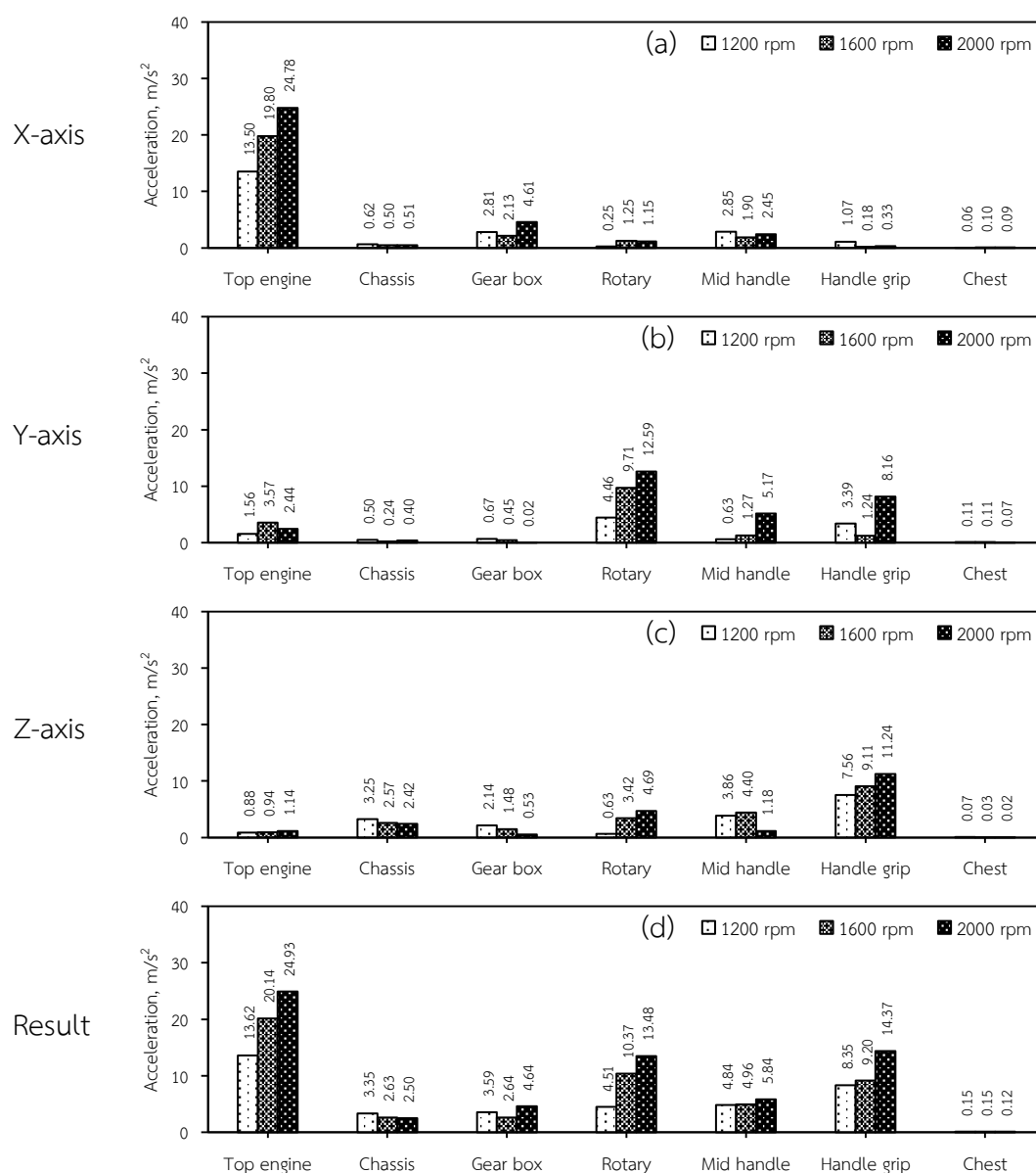
ภาพที่ 38 ค่าความเร่งของการสั่นสะเทือนที่ตำแหน่งต่างๆ บนรถไถเดินตาม กรณีรถไถเดินตามล้อเหล็กเงื่อนไขไม่เคลื่อนที่
