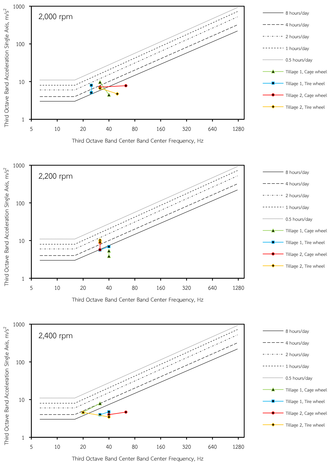
ภาพที่ 72 ค่ามาตรฐานความสั่นสะเทือนที่มือตามข้อเสนอแนะของ ANSI เครื่องไถพรวนดินด้วยใบมีดจอบหมุนญี่ปุ่นรูปตัวซี 14 ใบ
