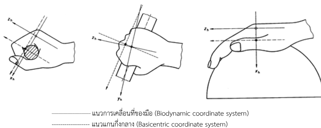
ภาพที่ 3 การสั่นสะเทือนในแนวแกนอ้างอิงต่างๆ ของมือ
