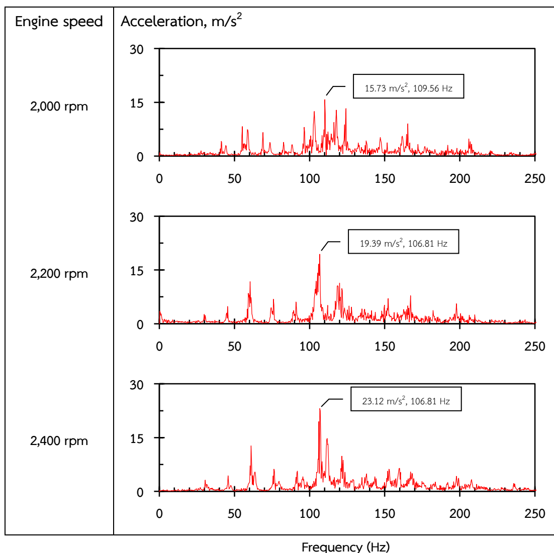
ภาพที่ 56 สเปกตรัมของค่าความเร่งลัพธ์ของการสั่นสะเทือนที่ตำแหน่งผิวบนเครื่องยนต์ กรณีสถิตไถเดินตามล้อเหล็กเงื่อนไขไถพรวนดินเที่ยวที่ 1 โดยใช้ใบมีดจอบหมุนญี่ปุ่นรูปตัวซี 14 ใบ
