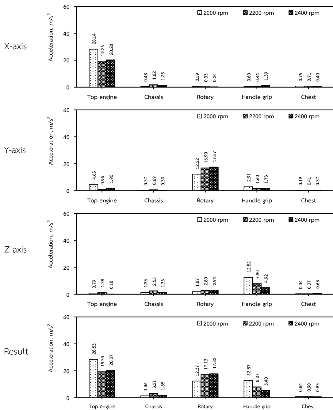
ภาพที่ 67 ค่าความเร่งของการสั่นสะเทือนของรถไถเดินตามล้อยางเงื่อนไขไถพรวนดินเดี่ยวที่ 1 ด้วยใบมีดจอบหมุนต้นแบบ 10 ใบ
