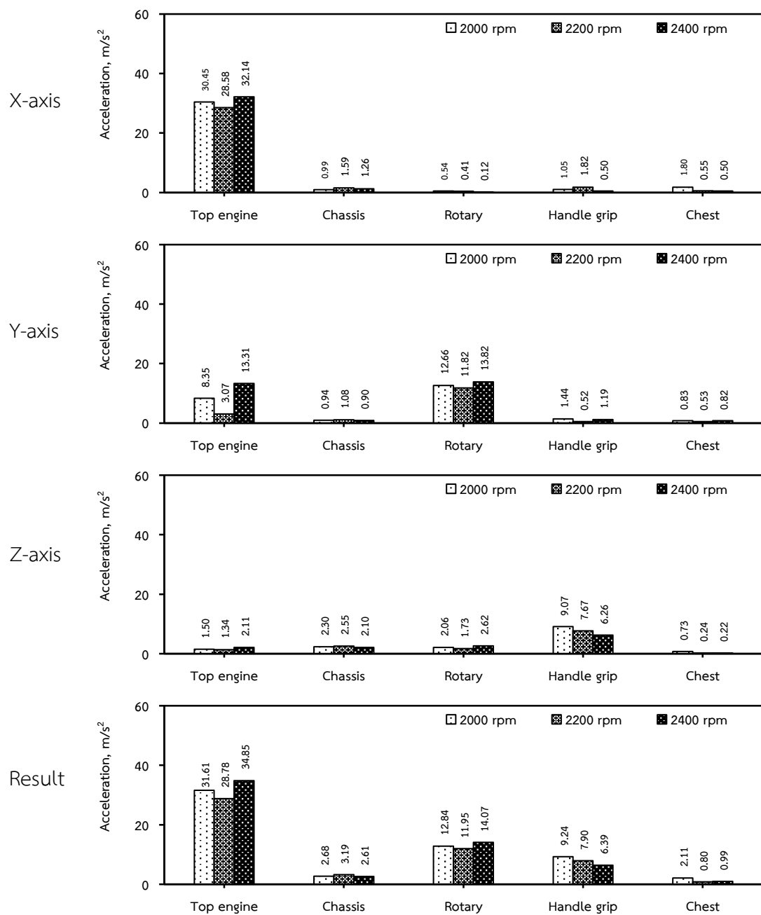
ภาพที่ 64 ค่าความเร่งของการสั่นสะเทือนของรถไถเดินตามล้อยางเส้นไขว้ไถพรวนดินเดี่ยวที่ 2 ด้วยใบมีดจอบหมุนต้นแบบ 14 ใบ
