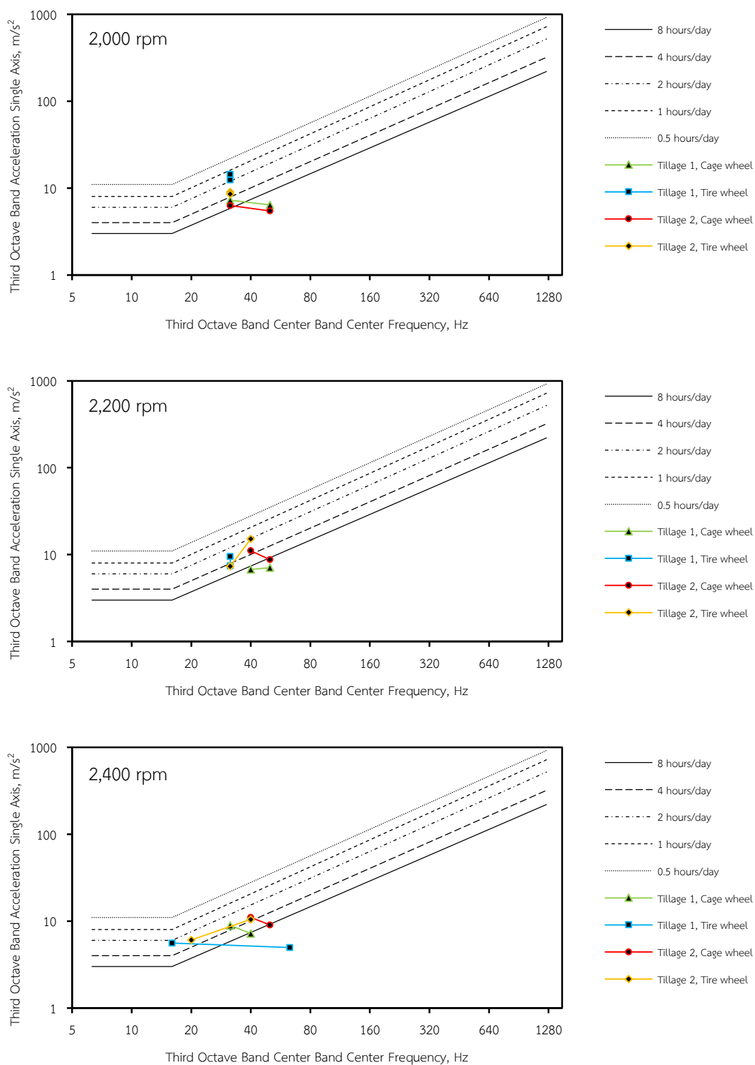
ภาพที่ 74 ค่ามาตรฐานความสั่นสะเทือนที่มือตามข้อเสนอแนะของ ANSI เครื่องไถพรวนดินด้วย ใบมีดจอบหมุนต้นแบบ 10 ใบ
