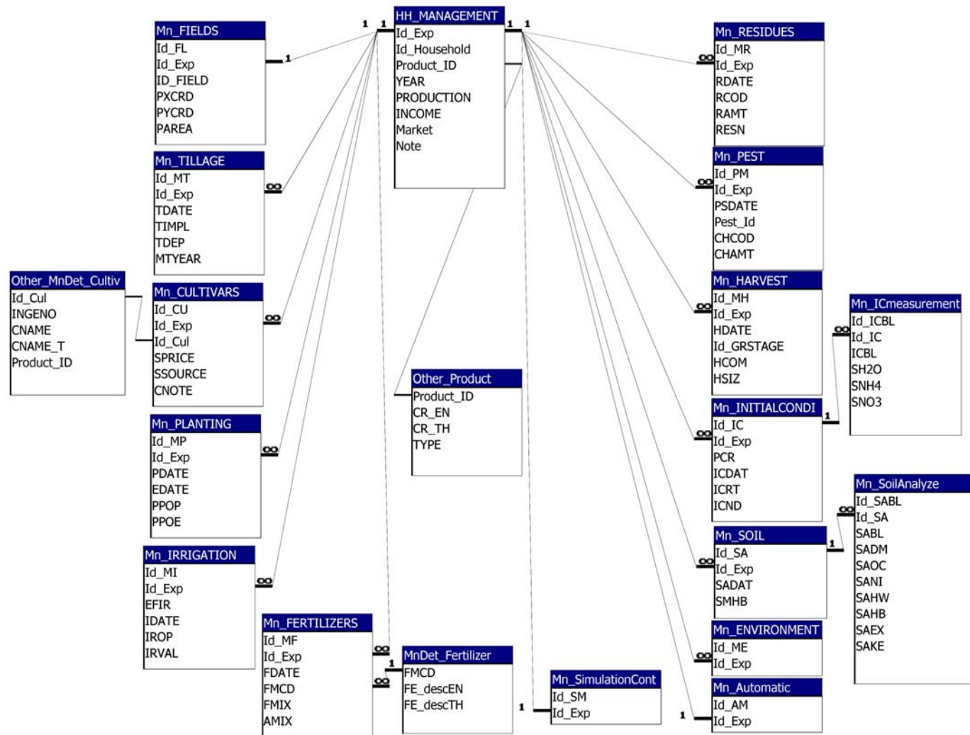
ภาคผนวก 5 แผนภาพความสัมพันธ์ของตารางข้อมูลในฐานข้อมูล CPM.mdb
