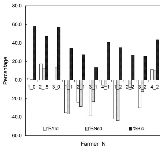
รูป 3: เปรียบเทียบความแตกต่างระหว่างค่าวัดจริงกับแบบจำลองของผลผลิต (Yld) จำนวนเมล็ดต่อตารางเมตร, (Nsd) และน้ำหนักมวลทั้งหมด (Bio) ของข้าวพันธุ์สันป่าตอง 1 ในปี 2545 เลขตัวหน้าของ Farmer_N คือเกษตรกร และเลขตัวหลังคือระดับปุ๋ยเรียงตามตาราง 1
