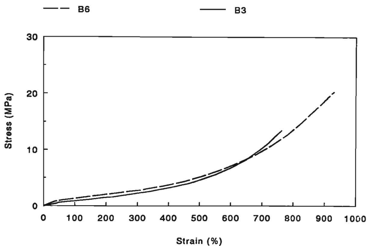
รูปที่ 4.17 กราฟเปรียบเทียบแสดงความเค้น-ความเครียด (Stress-strain curves) ระหว่าง B3 (50% SBR) และ B6 (50% ULDPE) ทดสอบด้วยอัตราเร็ว 500 มม./นาที
