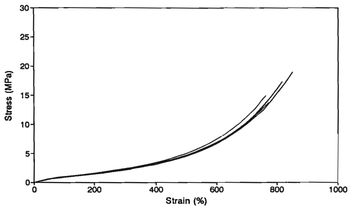
รูปที่ 4.6 กราฟแสดงความเค้น-ความเครียด (Stress-strain curves) ของ B3(50% SBR) ทดสอบด้วยอัตราเร็ว 500 มม./นาที
