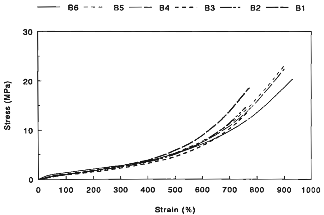
รูปที่4.18 กราฟเปรียบเทียบแสดงความเค้น-ความเครียด(Stress-strain curves)ของยางผสมB1-B6 ทดสอบด้วยอัตราเร็ว 500 มม./นาที
