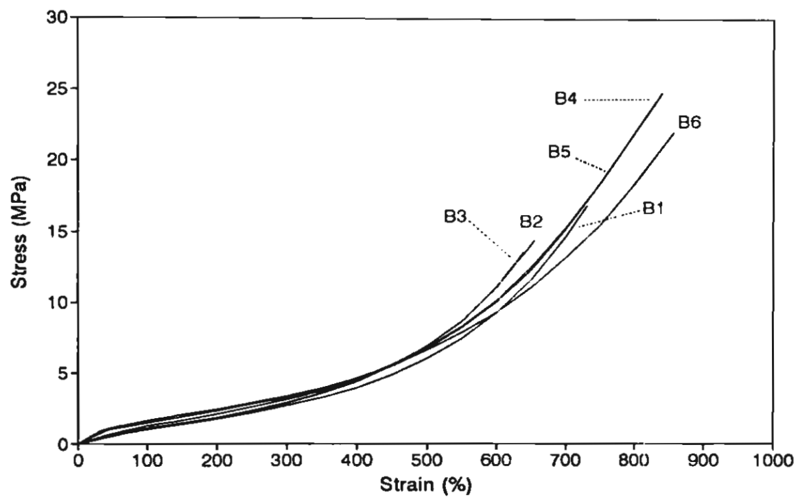
รูปที่ 5.2 กราฟเปรียบเทียบแสดงความเค้น-ความเครียด (Stress-strain curves) ของยางผสม B1-B6 ทดสอบด้วยอัตราเร็ว 500 มม./นาที
