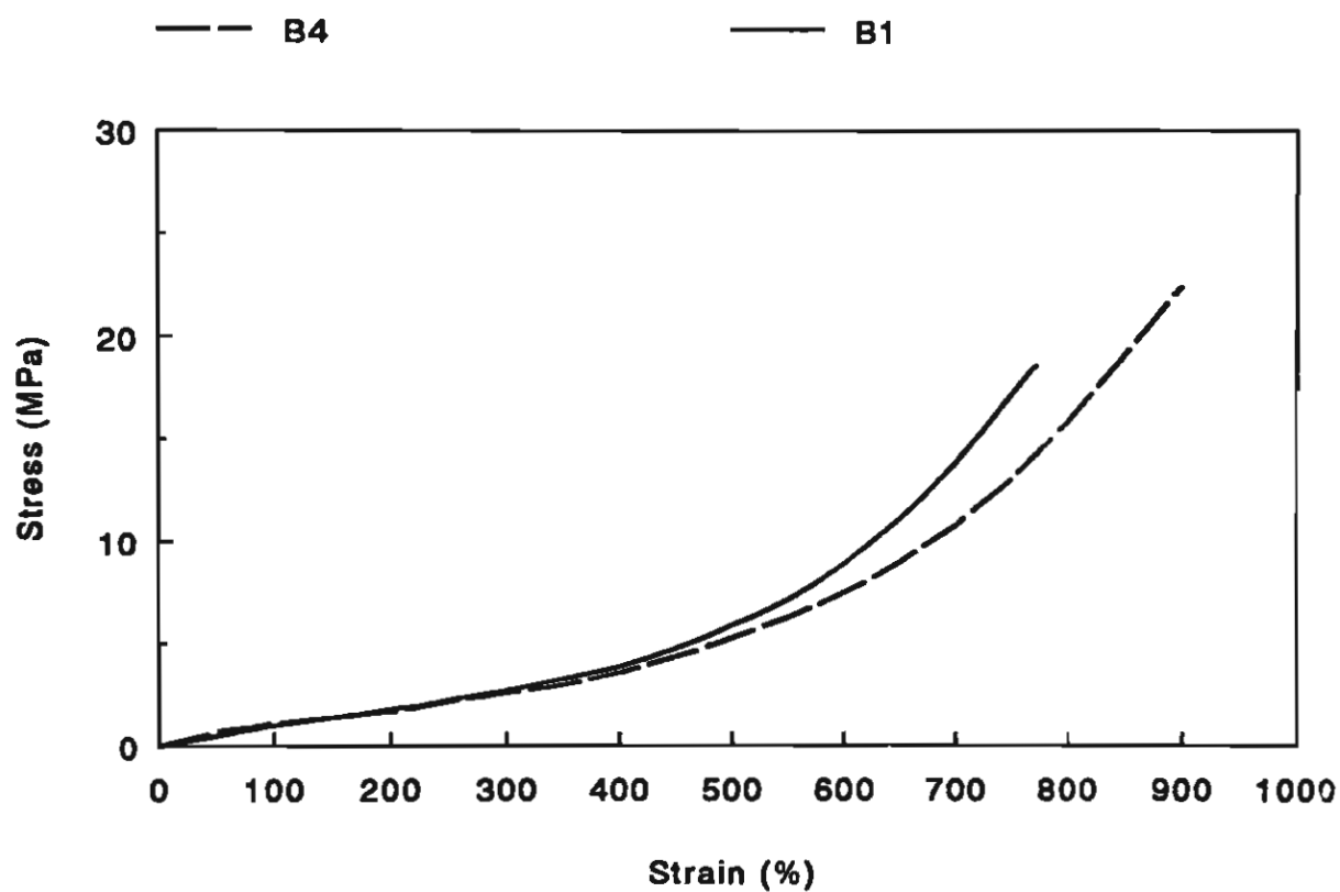
รูปที่ 4.15 กราฟเปรียบเทียบแสดงความเค้น-ความเครียด (Stress-strain curves) ระหว่าง B1 (30% SBR) และ B4 (30% ULDPE) ทดสอบด้วยอัตราเร็ว 500 มม./นาที
