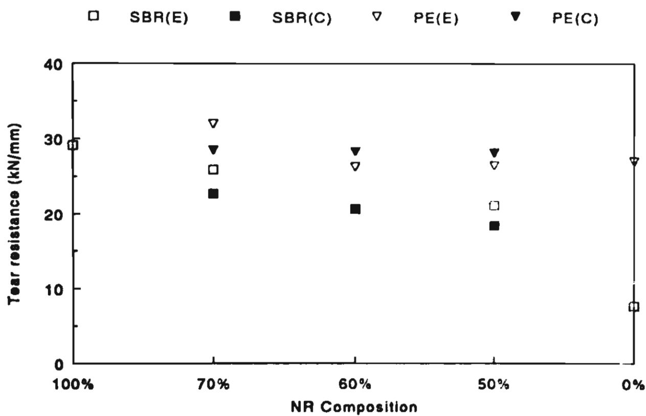
รูปที่ 4.19 กราฟแสดงการเปรียบเทียบความต้านทานการฉีกขาด(Tear resistance) ที่ได้จาก การทดลอง (E) และที่ได้จากการคำนวณ (C) ของยางผสมNR/SBR (SBR) และยางผสมNR/ULDPE (PE)
