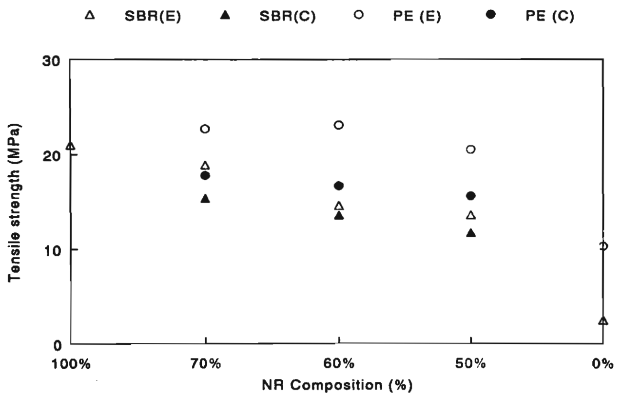
รูปที่4.13 กราฟแสดงการเปรียบเทียบค่าแรงดึงที่จุดขาด(Tensile strength) ที่ได้จากการทดลอง (E) และที่ได้จากการคำนวณ (C) ของยางผสมNR/SBR (SBR) และยางผสมNR/ULDPE (PE)
