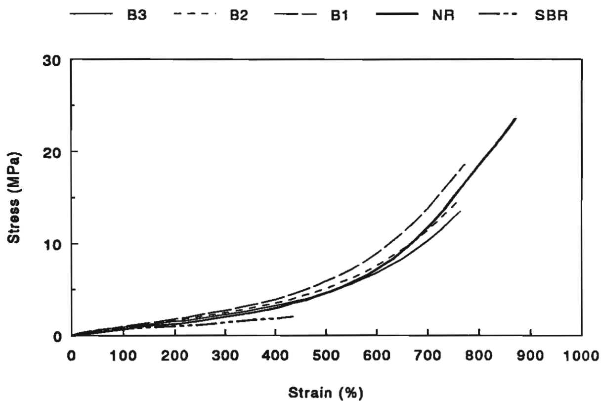
รูปที่ 4.11 กราฟเปรียบเทียบแสดงความเค้น-ความเครียด (Stress-strain curves) ของ NR SBR และ B1-B3 ทดสอบด้วยอัตราเร็ว 500 มม./นาที
