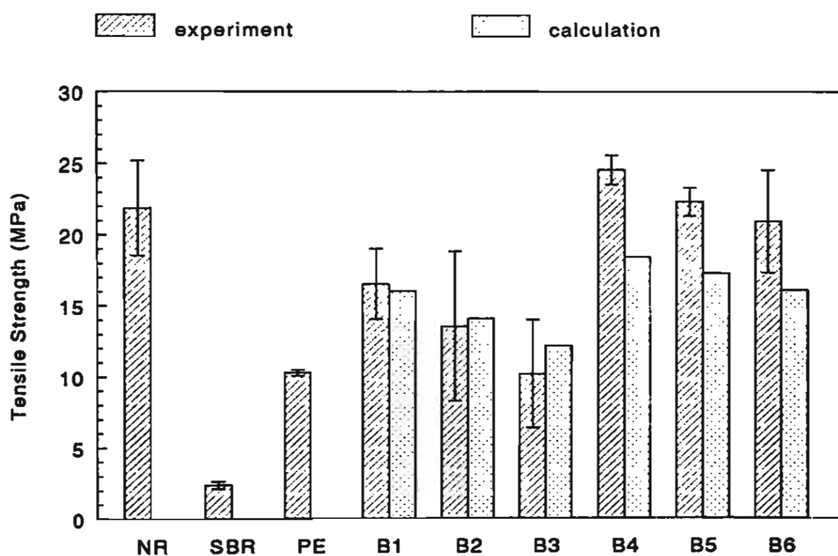
รูปที่ 5.5 กราฟแสดงการเปรียบเทียบค่าแรงดึงที่จุดขาด (Tensile strength) ที่ได้จากการทดลอง (experiment) และที่ได้จากการคำนวณ (calculation) ของ NR SBR ULDPPE ยางผสม NR/SBR (B1-B3) และยางผสม NR/ULDPPE (B4-B6)
