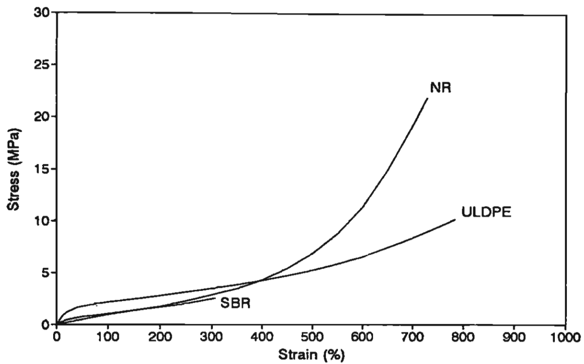
รูปที่5.1 กราฟเปรียบเทียบแสดงความเค้น-ความเครียด(Stress-strain curves)ของNR SBR และULDPE ทดสอบด้วยอัตราเร็ว 500 มม./นาที
