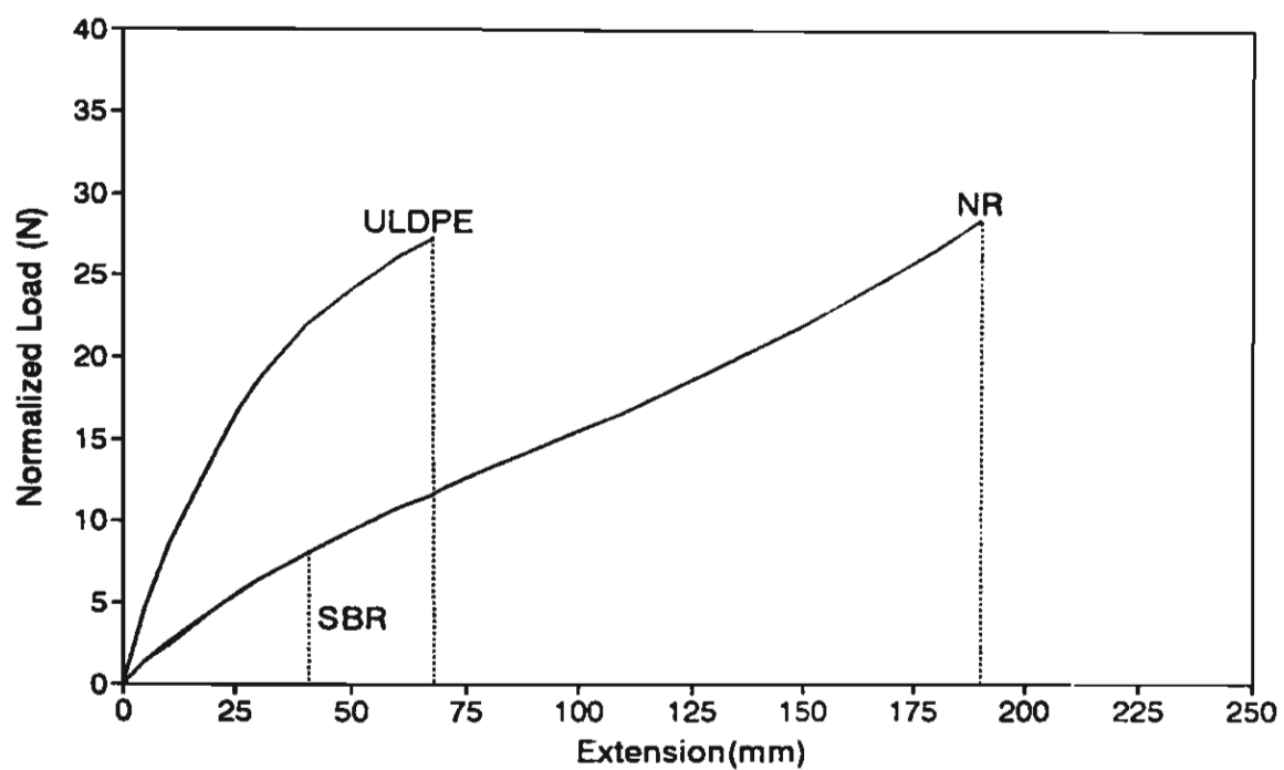
รูปที่ 4.20 กราฟเปรียบเทียบแสดง Load-extension curves จากการทดสอบความต้านทานการฉีกขาด (Tear resistance) ของ NR SBR และ ULDPE ทดสอบด้วยอัตราเร็ว 500 มม. / นาที
