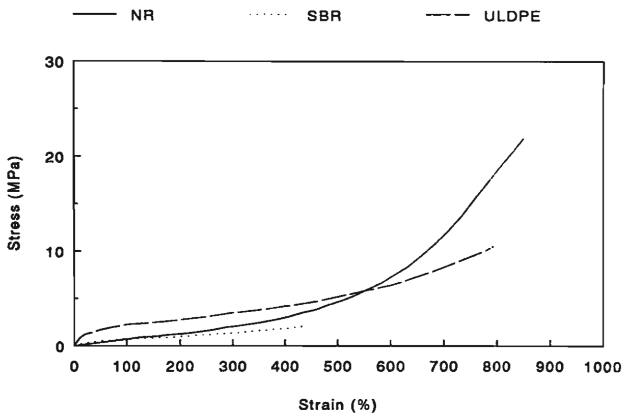
รูปที่ 4.10 กราฟเปรียบเทียบแสดงความเค้น-ความเครียด (Stress-strain curves) ของ NR SBR และ ULDPE ทดสอบด้วยอัตราเร็ว 500 มม./นาที
