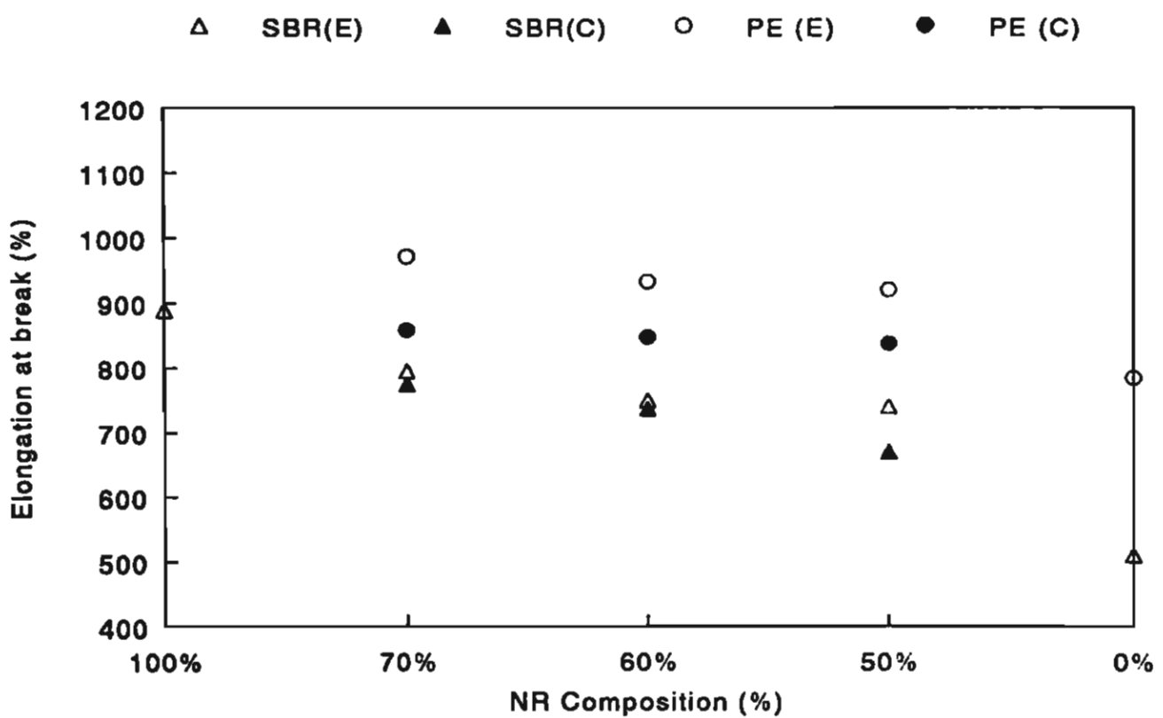
รูปที่ 4.14 กราฟแสดงการเปรียบเทียบระยะยืดที่จุดขาด (Elongation at break) ที่ได้จากการทดสอบ (E) และที่ได้จากการคำนวณ (C) ของยางผสม NR/SBR (SBR) และยางผสม NR/ULDPE (PE)
