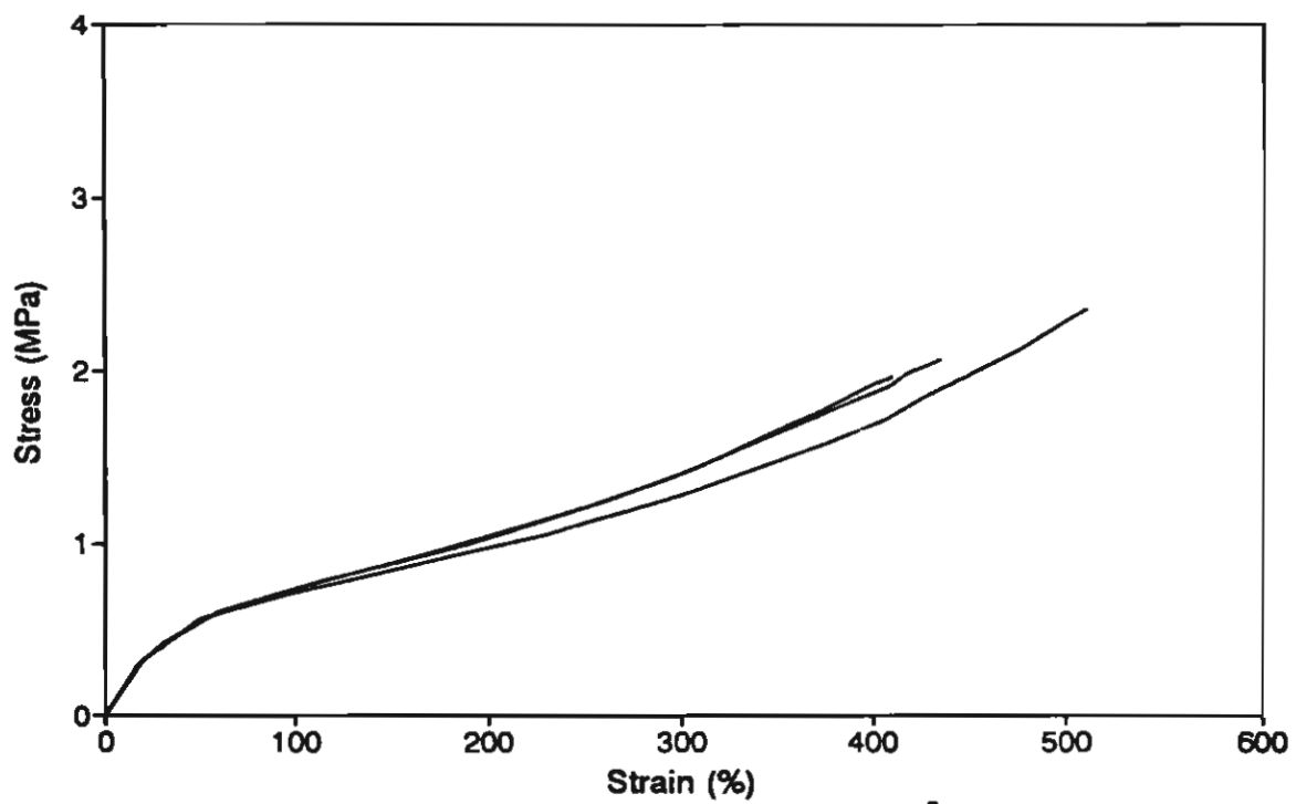
รูปที่ 4.2 กราฟแสดงความเค้น-ความเครียด (Stress-strain curves) ของ SBR ทดสอบด้วย อัตราเร็ว 500 มม./นาที
