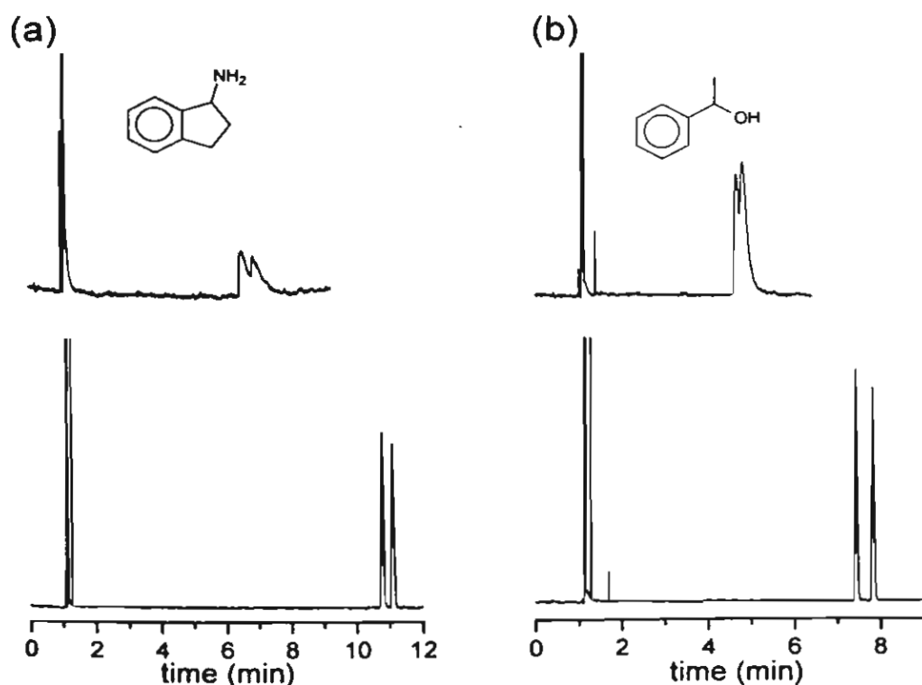
รูปที่ 5 โครมาโทแกรมของ (a) เอมีน #12 และ (b) แอลกอฮอล์ #15 ที่วิเคราะห์ด้วยคอลัมน์ CD-2 (ภาพล่าง) และคอลัมน์ CD-3 (ภาพบน) ที่อุณหภูมิ 120 °C
