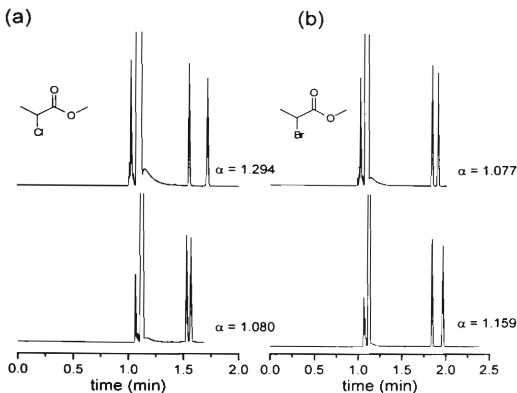
รูปที่ 6 โครมาโทแกรมของ (a) เอสเทอร์ #23 และ (b) เอสเทอร์ #24 ที่วิเคราะห์ด้วยคอลัมน์ CD-2 (ภาพล่าง) และคอลัมน์ CD-3 (ภาพบน) ที่อุณหภูมิ 120 °C
