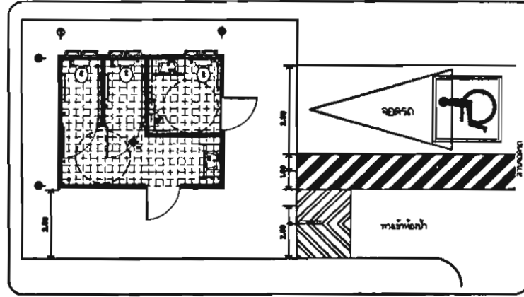
ผังบริเวณ TYPE 5 0.2 m 1 m 0.1 m 0.5 m
