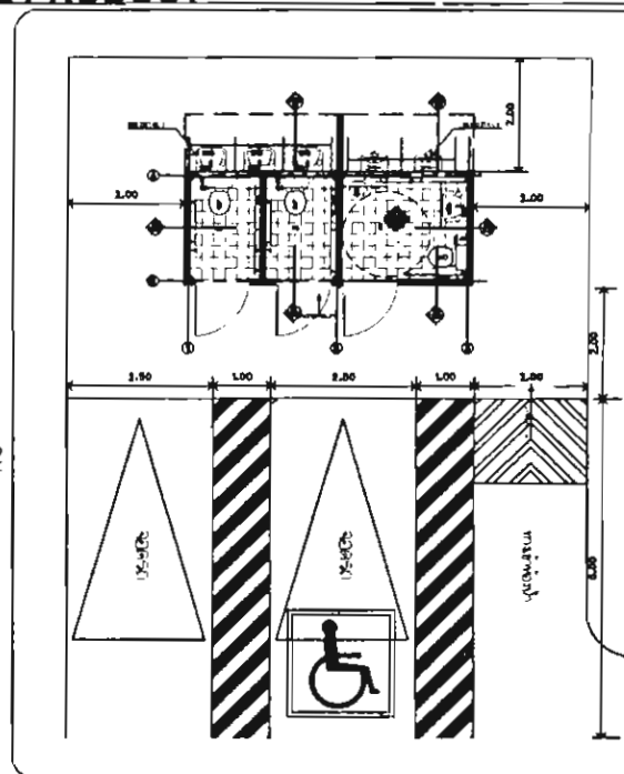
ผังบริเวณห้องน้ำ TYPE 4 0.2 m. 1 m. 0.1 m. 0.5 m.
