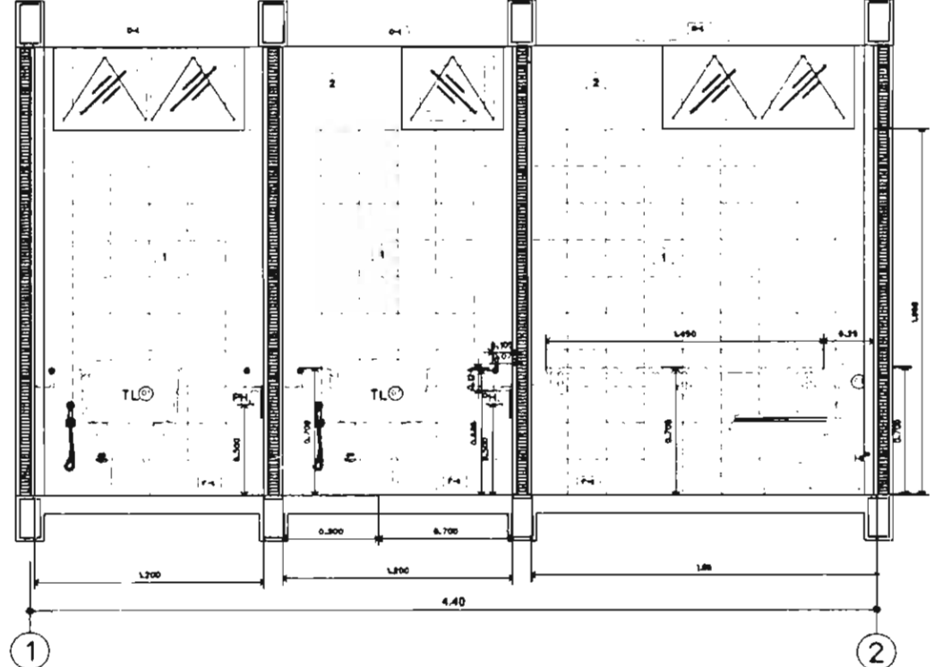
รูปตัดห้องสุขาหญิง 3.4 A3-87
