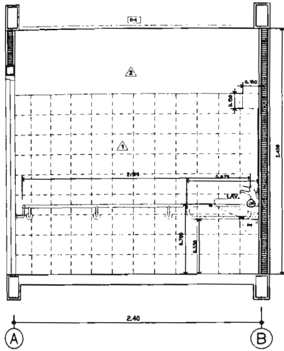
รูปตัดห้องสุขาหญิง E.2.4 A.E.2-07
