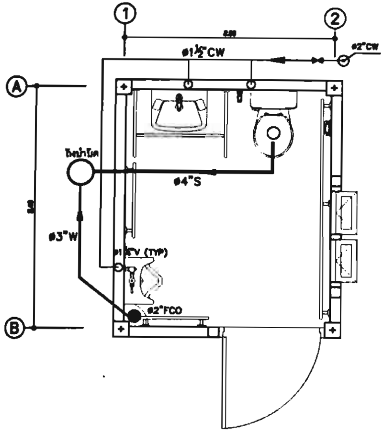
ผังสุขาภิบาลสุขาสาธารณะผู้สูงอายุและผู้พิการ (ชาย)
