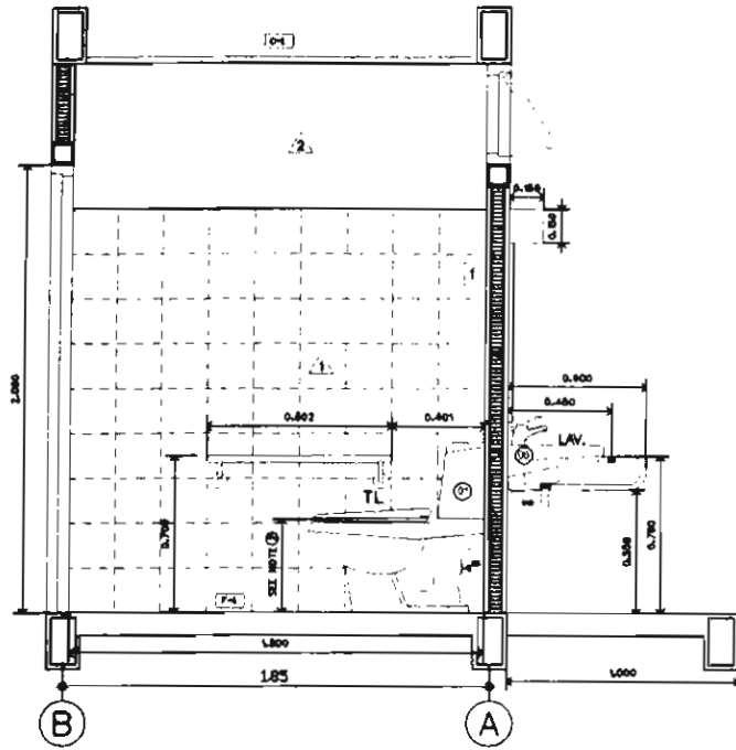
รูปตัดห้องส้วม อ่างล้างหน้า 4.1 A4-03
