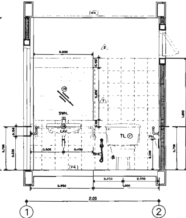
รูปตัดห้องสุขาหญิง E.2.5 A.E.2-07
