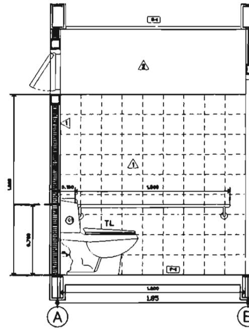
รูปด้านห้องสุขา 7
