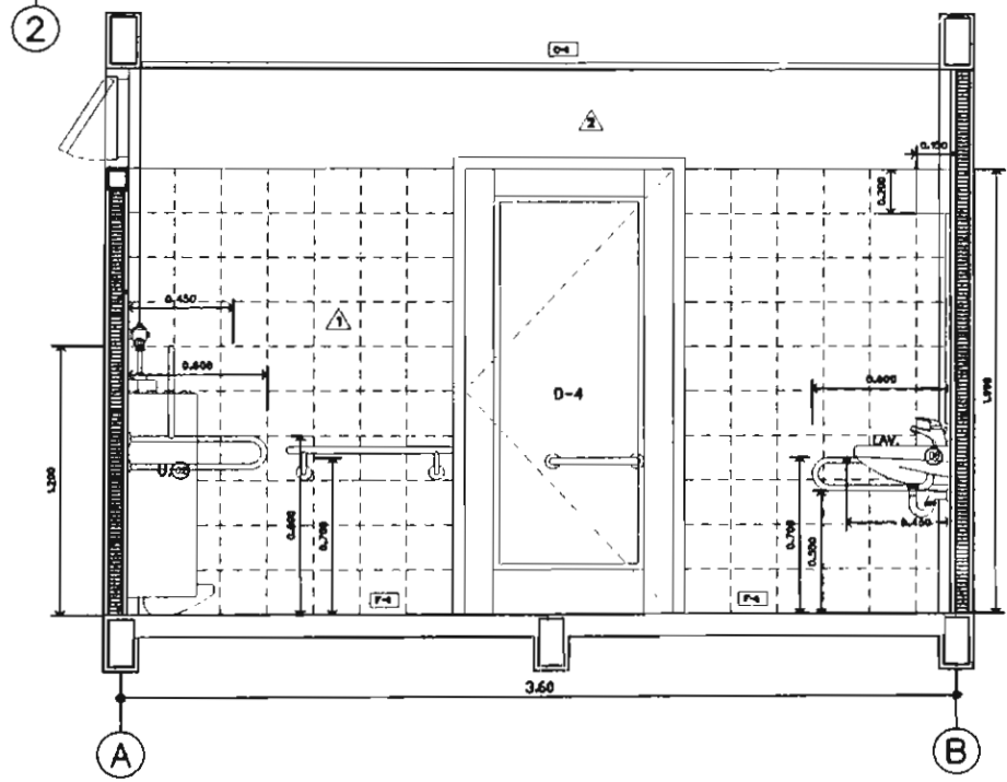
รูปด้านห้องสุขาชาย 2
