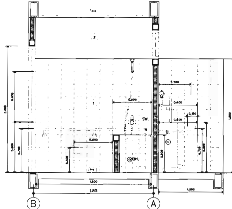
รูปตัดห้องอาบน้ำ โถบ้นชำระชาย 4.2 A4-05
