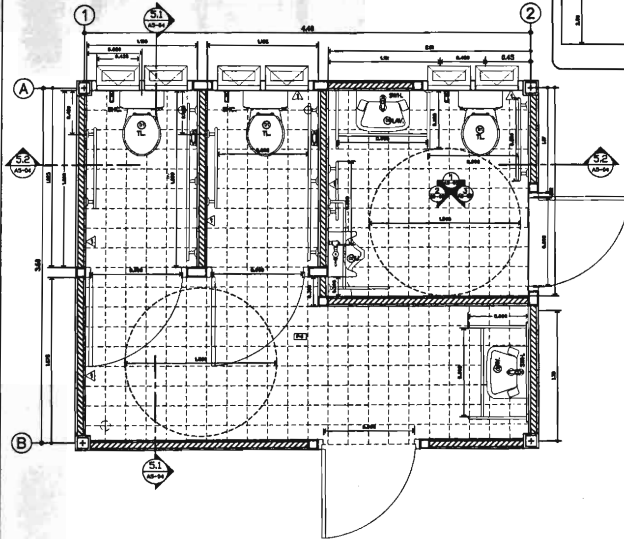
แบบ สุขาสาธารณะผู้สูงอายุและผู้พิการ TYPE 5
