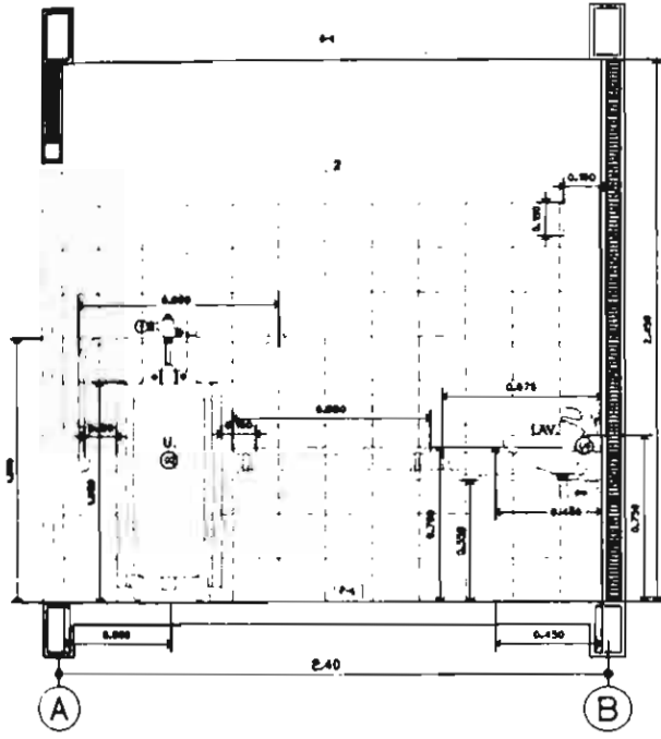
รูปตัดห้องสุขาชาย 2.2.1 AE 2-04
