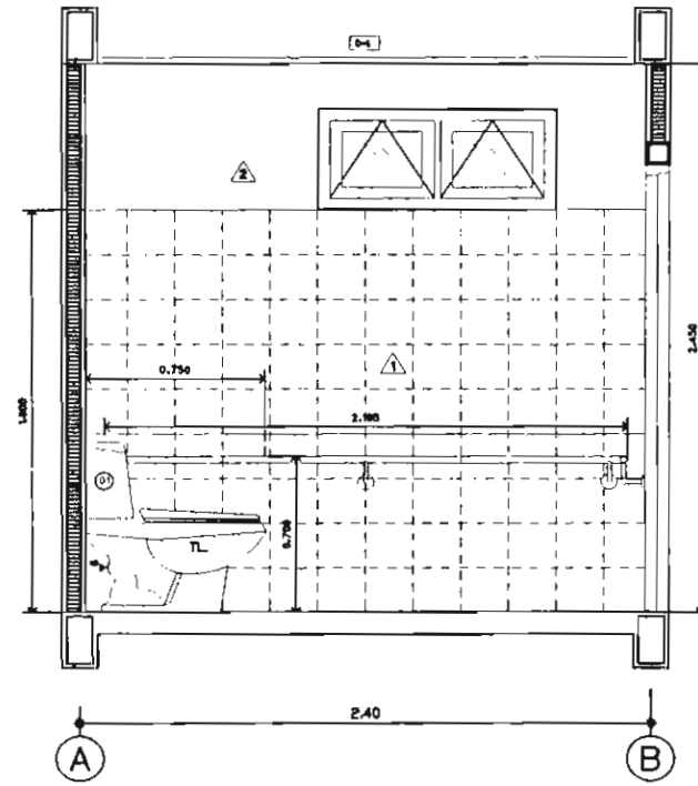
รูปตัดห้องสุขาหญิง E.2.6 A.E.2-07
