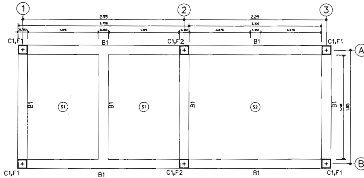
ผังโครงสร้าง TYPE 4
