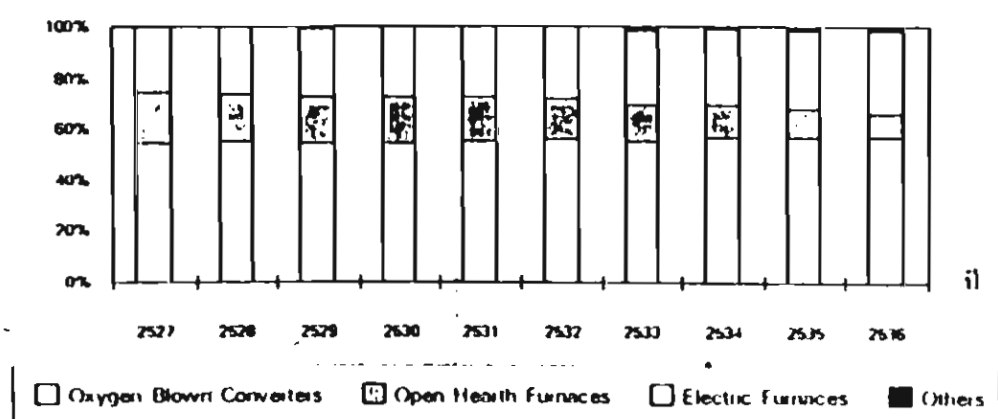
แผนภาพที่ 2.13 สัดส่วนผลผลิตเหล็กกล้าดิบตามประเภทของขบวนการผลิต ในช่วงปี 2527-2536
