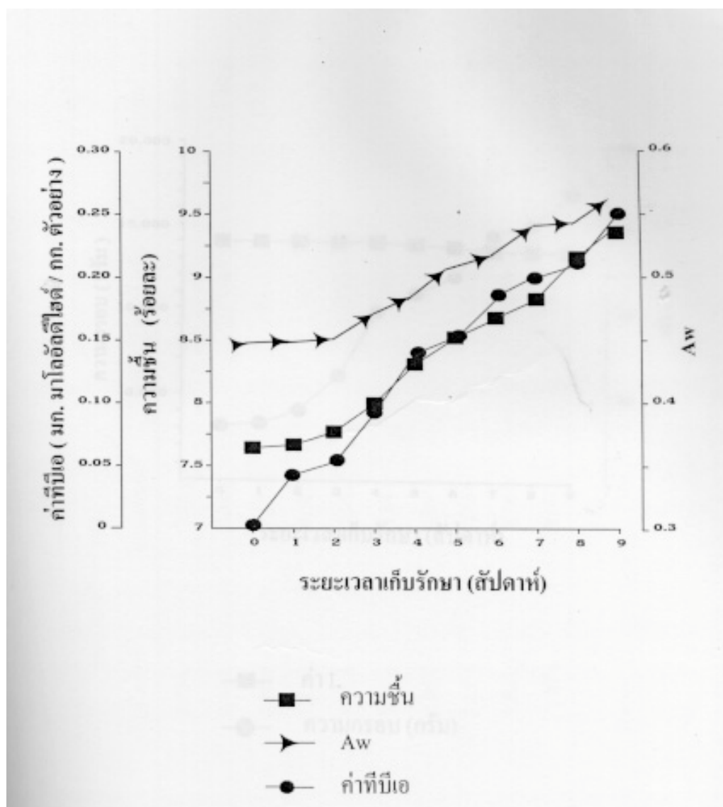
ภาพที่ 18 การเปลี่ยนแปลงค่าพีบีเอ ความชื้น และ Aw ของข้าวพองเสริมใยอาหารร้อยละ 1.5 ระหว่างการเก็บรักษา
