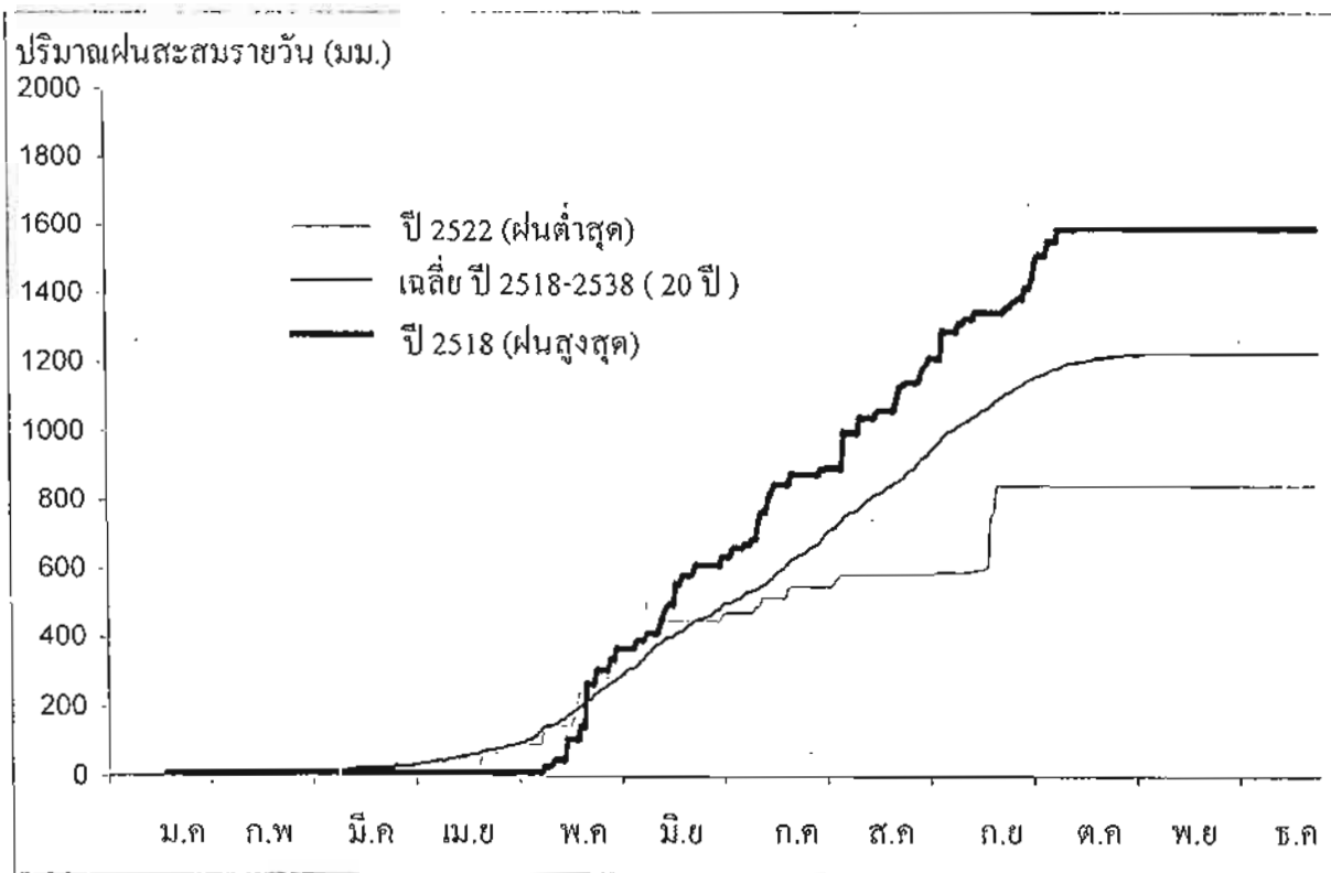
รูปที่ 25 การกระจายตัวของปริมาณฝนสะสม ของปีที่มีปริมาณฝนต่ำสุด ปีที่มีปริมาณฝนสูงสุด และ ปริมาณฝนเฉลี่ย ของ อ.พนมไพร จ.ร้อยเอ็ด
