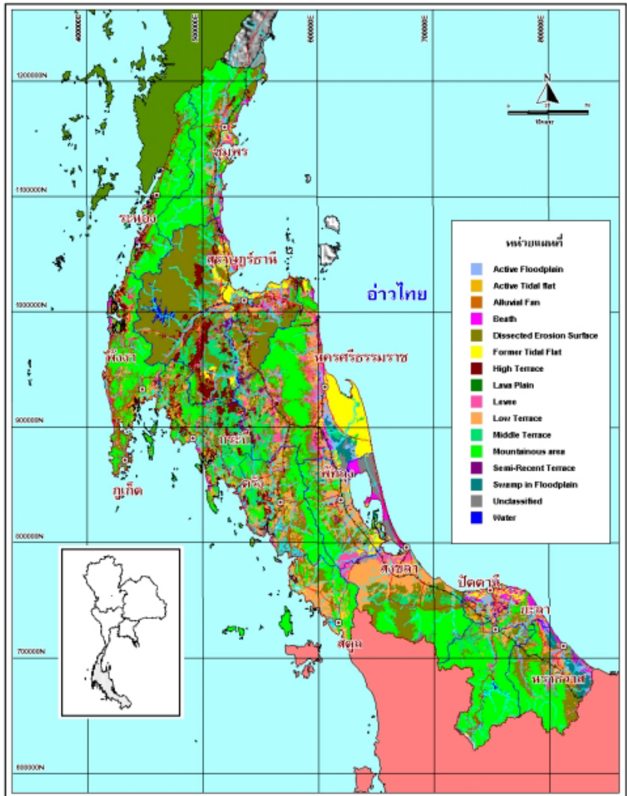
รูปที่ 2-10 สภาพพื้นที่ของภาคใต้
