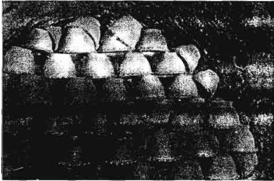
รูปที่ 4.18 การบรรจุผลิตภัณฑ์เข้าเตาเผา
