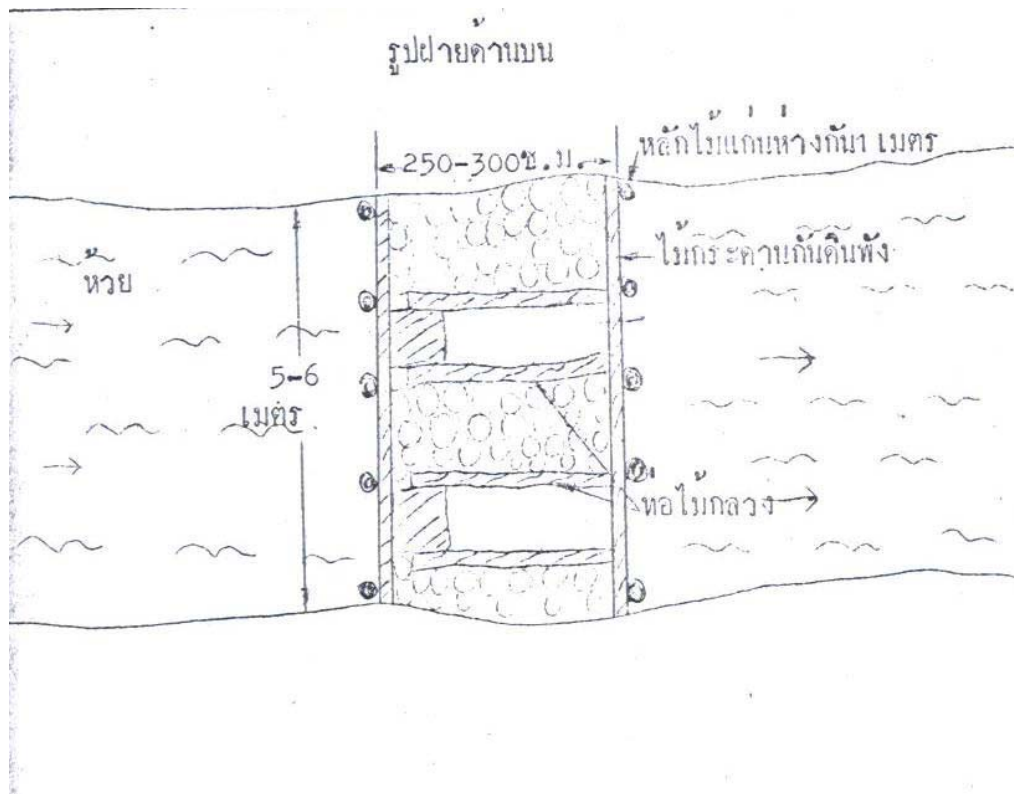
รูป 2.4 ฝายบ้านฝาง อ.หนองเรือ จ.ขอนแก่น
