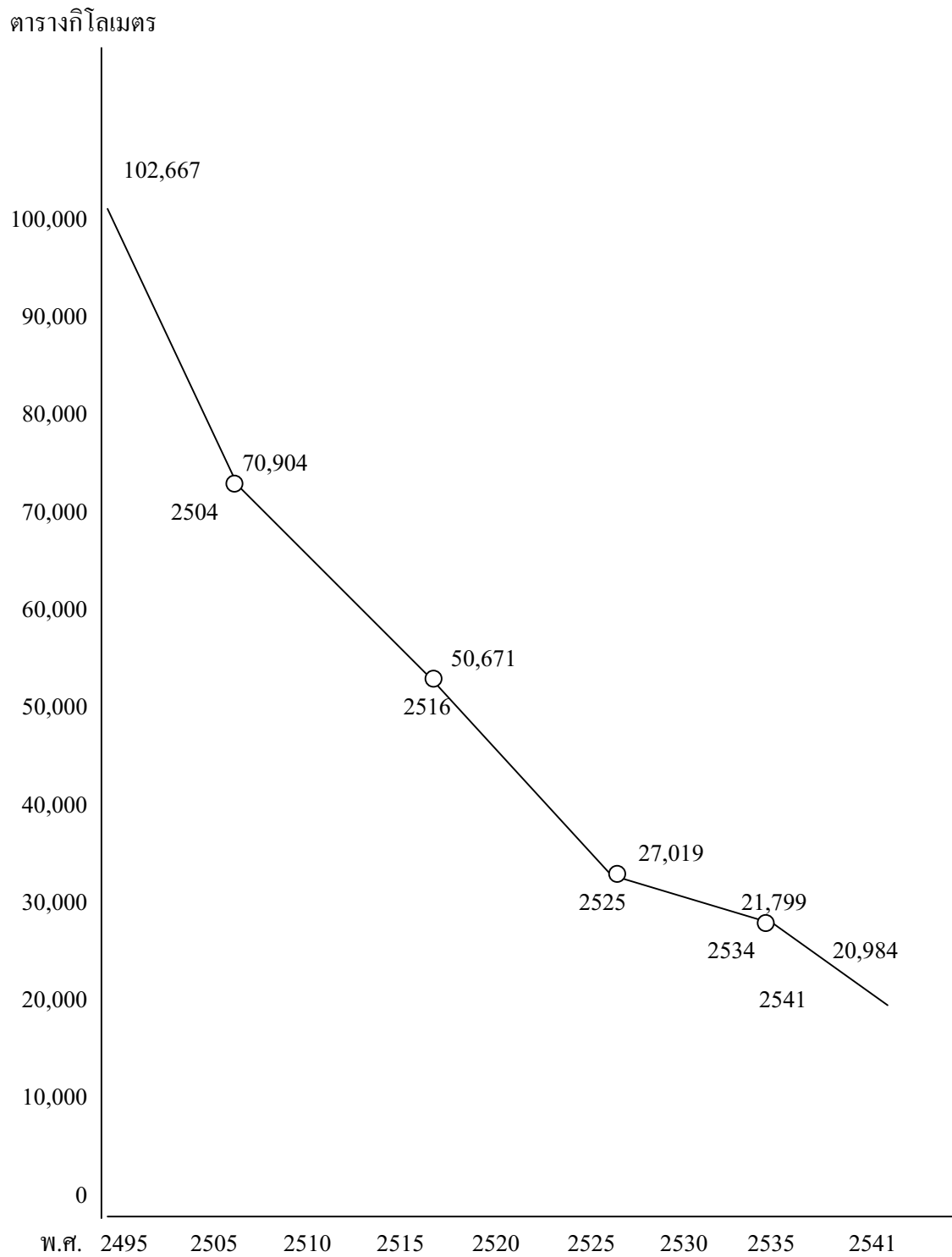
รูป 2.2 การลดลงของพื้นที่ป่าไม้ภาคอีสาน ตั้งแต่ พ.ศ. 2495-2541
