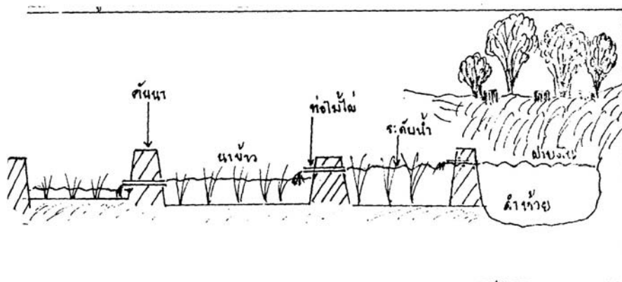
รูป 2.3 ฝายบ้านบัว อ.กุฉินคร จ.สกลนคร
