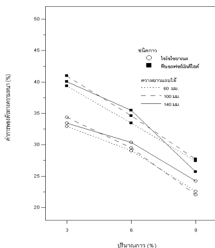
ภาพที่ 44 กราฟแสดงผลกระทบของชนิดกาก, ปริมาณกาก และความยาวของแถบไม้ ต่อการป้อนตัวทางความหนาของโอเอสแอล
