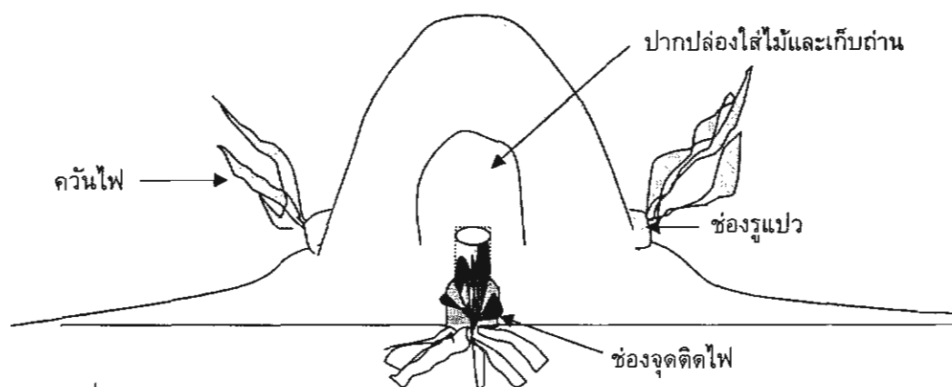
ภาพที่ 82 ภาพแสดงลักษณะการทำงานของเตาอบถ่านของพ่อถวิล รตภา
