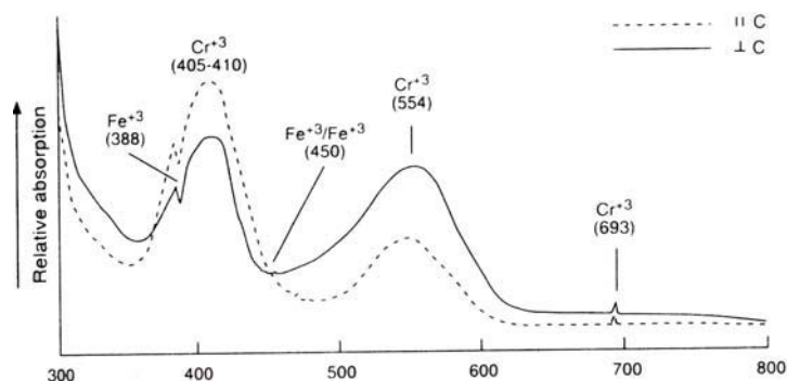
รูปที่ 4.18 ลักษณะกราฟของการดูดกลืนแสง UV-VIS-NIR ของพลอยคอร์ันดัม
