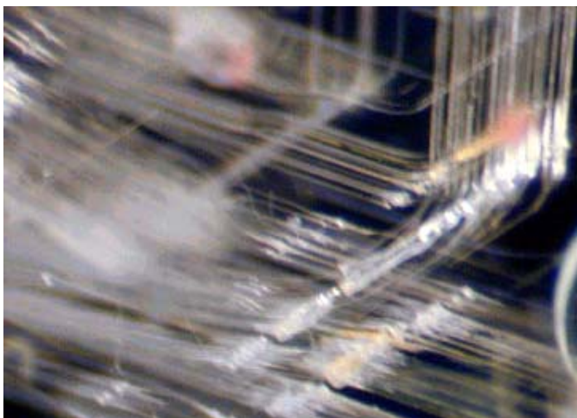
รูปที่ 3.24 มลทินท่อกลวง (Long tubes) วางตัวขนานกับแนวการเติบโตของ ผลึกแร่คอร์ันดัมในกลุ่มสีน้ำเงิน (SPI-B)
