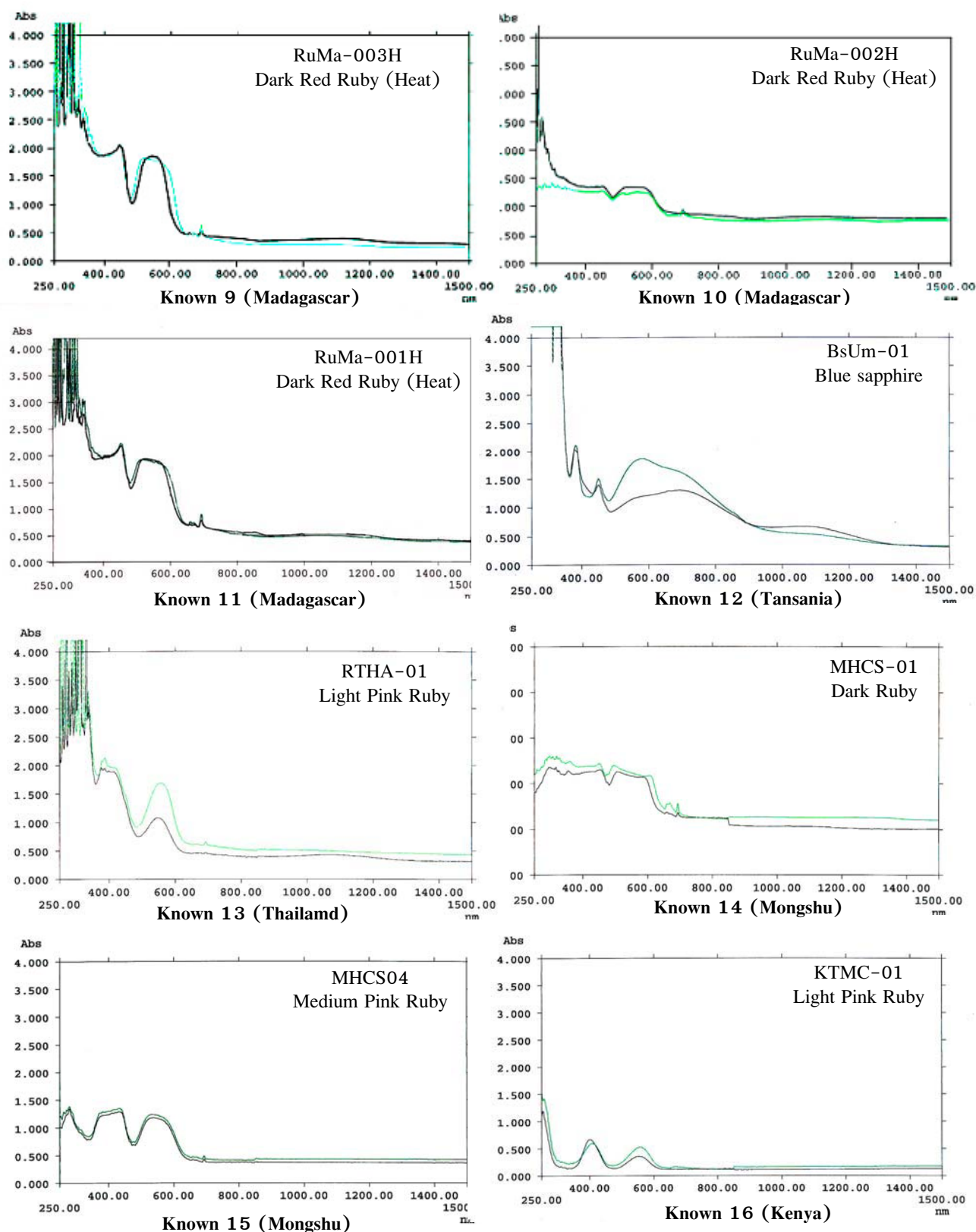
รูปที่ 4.56 ลักษณะสเปกตรัมของการดูดกลืนแสงช่วง UV-VIS-NIR ของตัวอย่างพลอยคอร์ันดัมที่ทราบแหล่งที่มา จำนวน 8 ตัวอย่าง จากทั้งหมด 24 ตัวอย่าง
