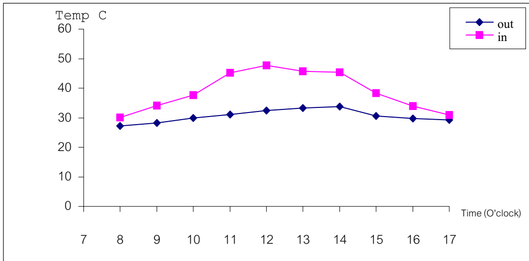
ภาพที่ 10 อุณหภูมิทั้งภายในและภายนอกกระโถมในเวลาต่างๆ
