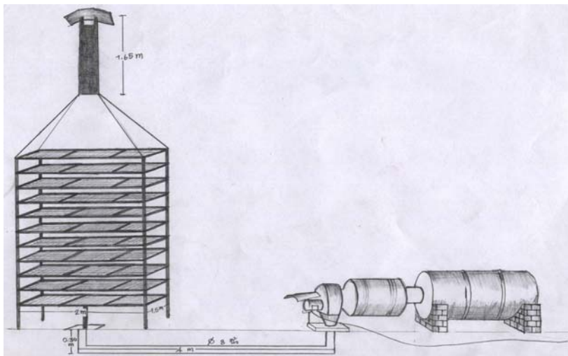
ภาพที่ 6 ลักษณะของ เครื่องอบหญ้าแห้งแบบ กระโจมปิรามิด
