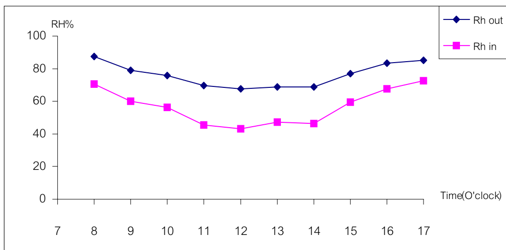
ภาพที่ 11 ความชื้นสัมพัทธ์ทั้งภายในและภายนอกกระโถมในเวลาต่างๆ
