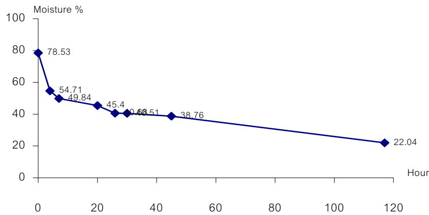
ภาพที่ 9 การเปลี่ยนแปลงของเปอร์เซ็นต์ความชื้นตามจำนวนชั่วโมงที่ใช้ในการอบในกระโจม
