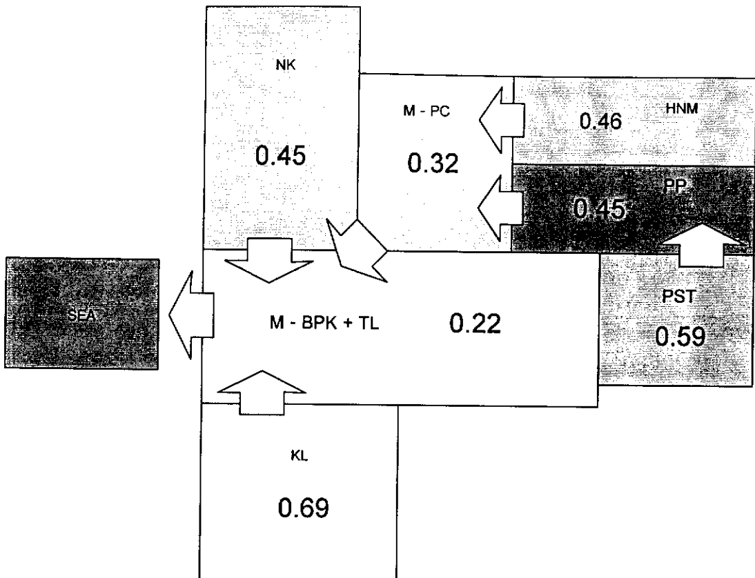
ภาพที่ 7 แผนภาพดัชนีบัญชีน้ำของอัตราส่วนปริมาณน้ำที่หมดไปต่อปริมาณน้ำเข้าทั้งหมดของ ฤดูฝน ในปี พ.ศ. 2537 (ปีฝนปกติ)
