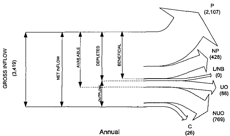
ภาพที่ 5 แผนภาพบัญชีน้ำของกลุ่มน้ำย่อยคลองพระสะถึง ปี พ.ศ. 2537 (ปีฝนปกติ)
