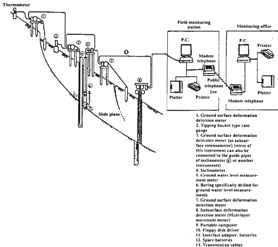
รูปที่ 2-18 ระบบการตรวจวัดการเคลื่อนตัวของลาดดินแบบอัตโนมัติ
