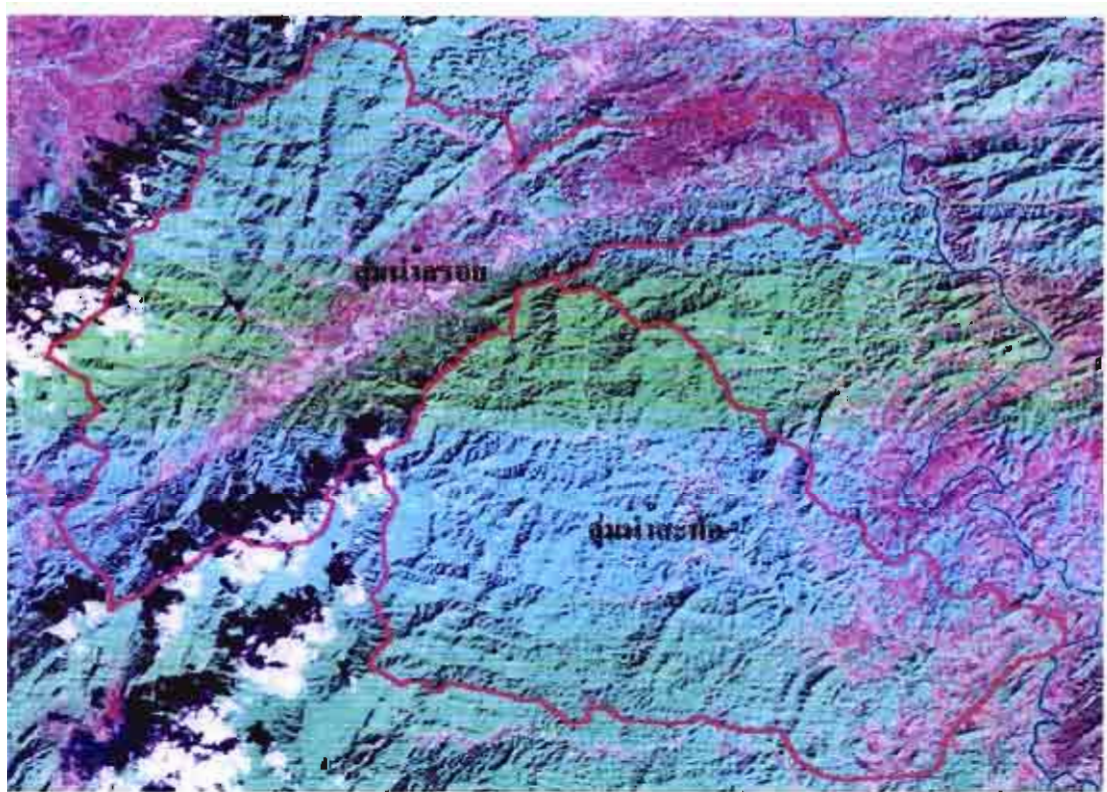
รูปที่ 8-21 ภาพถ่ายดาวเทียม LANDSAT TM GRB742 บริเวณกลุ่มน้ำสรอย - สะท้อ
