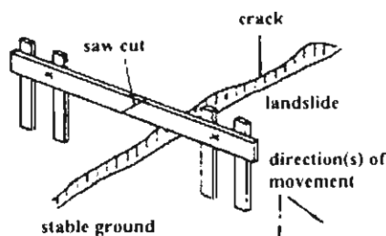
รูปที่ 2-17 การวัดการเคลื่อนตัวของลาดดินอย่างง่าย
