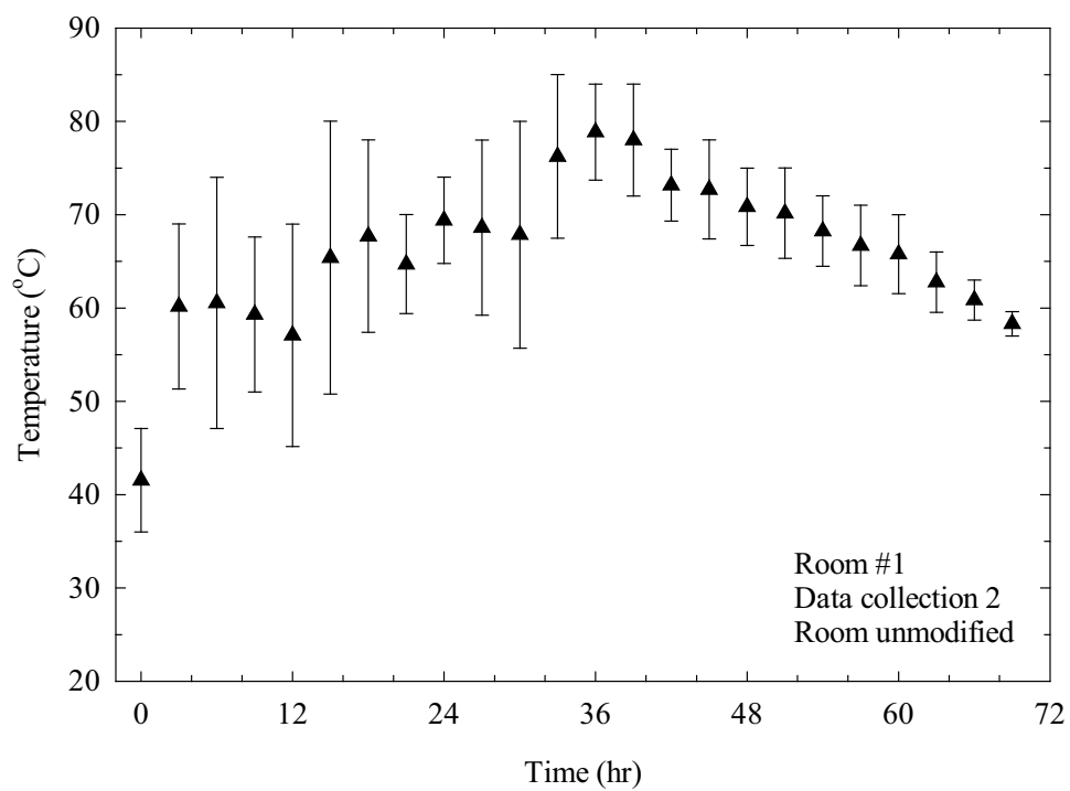
รูปที่ 6.4 อุณหภูมิในห้องรยางสำหรับห้องรตั่วอย่างหมายเลข 1 ครั้ที่ 2
