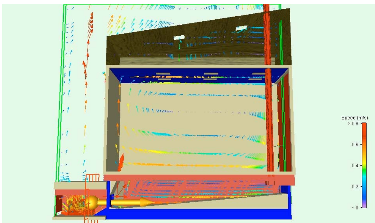
รูปที่ 7.17 การไหลของแก๊สในห้องที่ระบายกลางห้องตามความกว้าง
