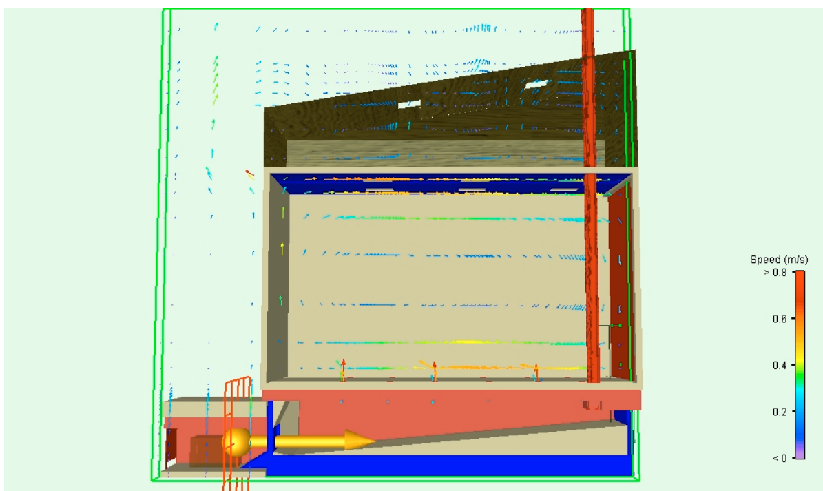
รูปที่ 7.18 การไหลของแก๊สในห้องที่ระบายช่องปล่อยแก๊ส
