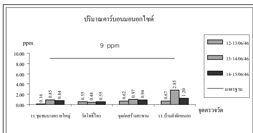
รูปที่ 3-7 ผลการตรวจวัดปริมาณฝุ่นละอองรวม ปริมาณฝุ่นละอองขนาดเล็กไม่เกิน 10 ไมครอน และปริมาณก๊าซคาร์บอนมอนอกไซด์ ระหว่างวันที่ 12-15 มิถุนายน 2546
