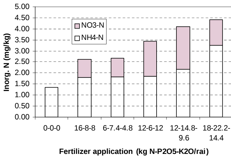
รูปที่ 2.23 ผลของปุ๋ยเคมีที่มีต่อปริมาณไนโตรเจน ( \text{NH}_4 และ \text{NO}_3 ) ในระดับความลึกต่าง ๆ ของดิน ชุดยางตลาด (YI) เมื่ออายุเก็บเกี่ยว
