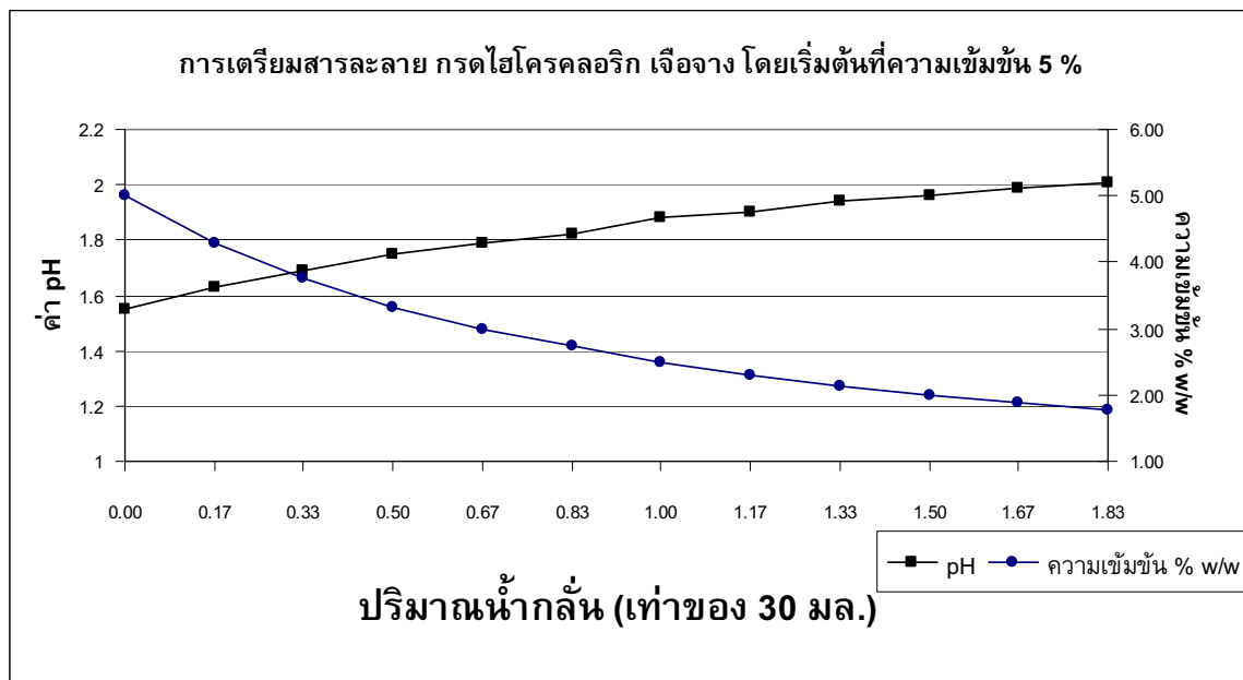
ภาพที่ 7-1 กราฟ แสดง ค่า pH ของสารละลาย กรดไฮโดรคลอริก ที่ความเข้มข้น 5% w/w เมื่อถูกเจือจาง
