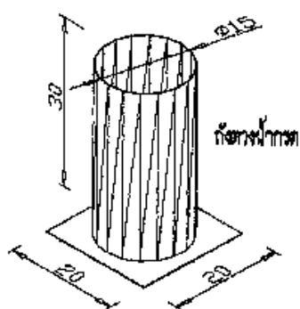
ถังตวงน้ำกาว
