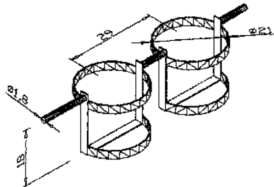
โครงถ้ำถังน้ำยาง
