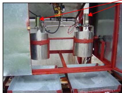
ภาพที่ 5.3 ชุดผสมน้ำยางกับน้ำกรด
