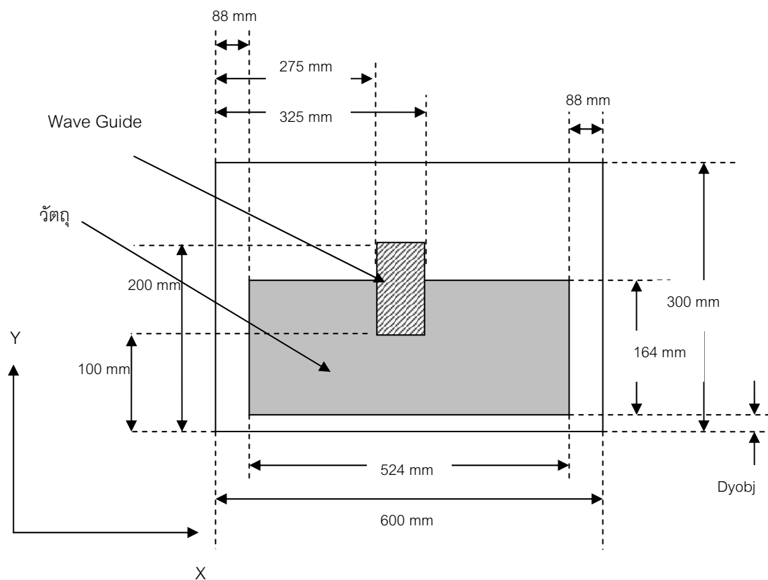
รูปที่ 52 ขนาด ตำแหน่งของท่อนำคลื่น ขนาดของโพรงสี่เหลี่ยม ขนาดของวัตถุ และตำแหน่งการวางวัตถุ
