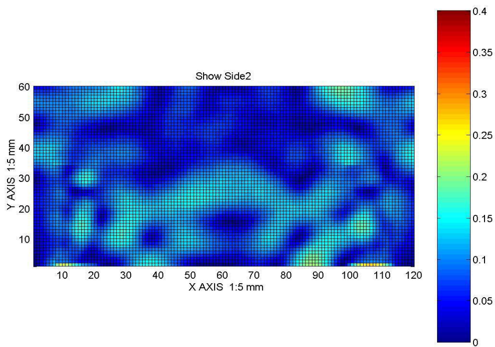
รูปที่ 51 สนามไฟฟ้าภายในวัตถุทรงกระบอกรูปวงแหวนที่ระนาบ YZ ที่ X = 300 มิลลิเมตร
