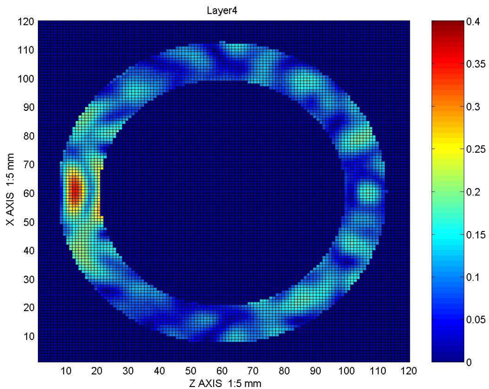
รูปที่ 48 สนามไฟฟ้าภายในวัตถุทรงกระบอกรูปวงแหวนที่ระนาบ XZ ที่ความหนา 120 มิลลิเมตรของวัตถุ
