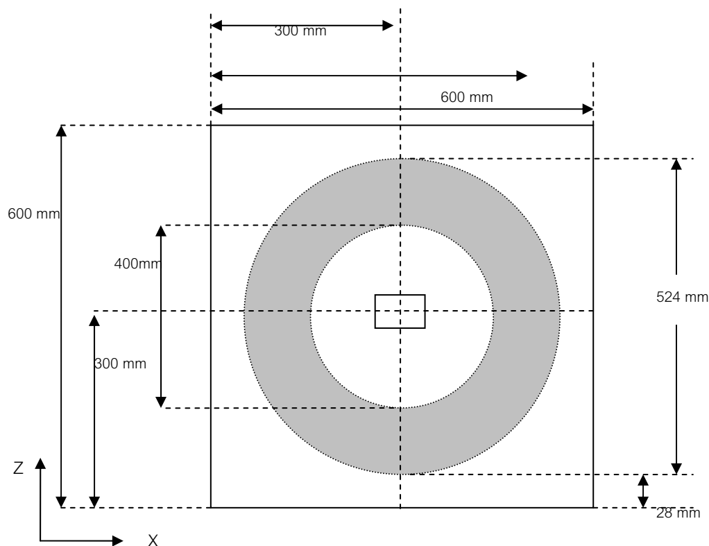
รูปที่ 62 ขนาด ตำแหน่งของท่อนำคลื่น ขนาดของโพรงสี่เหลี่ยม ขนาดของวัตถุ และตำแหน่งการวางวัตถุ
