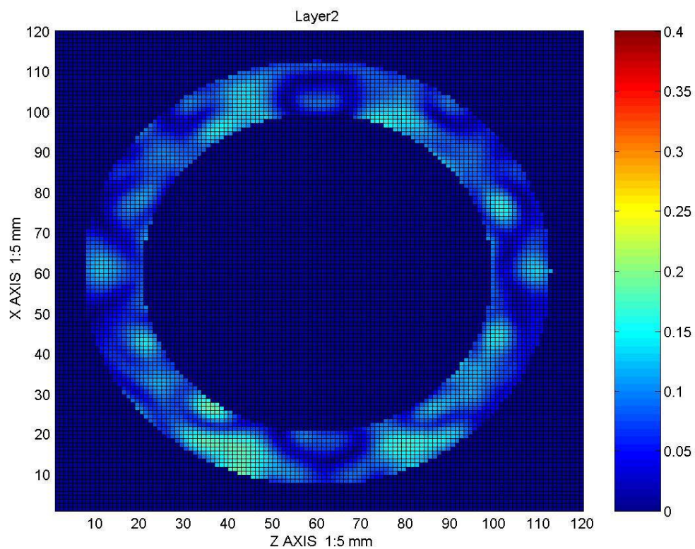
รูปที่ 64 สนามไฟฟ้าภายในวัตถุทรงกระบอกรูปวงแหวนที่ระนาบ XZ ที่ความหนา 40 มิลลิเมตรของวัตถุ
