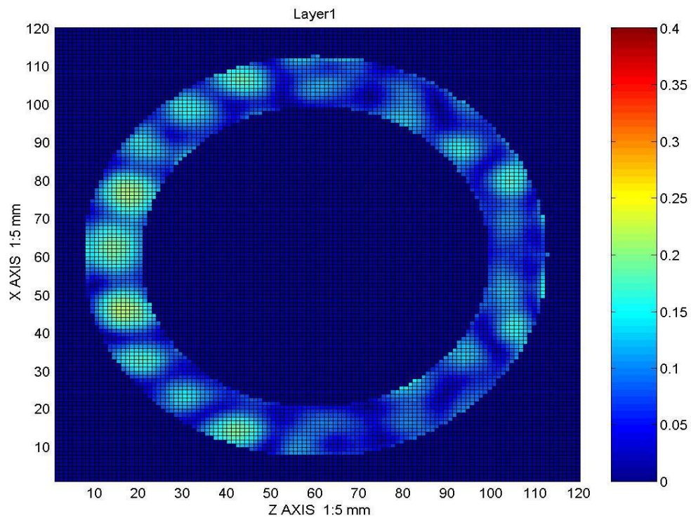
รูปที่ 54 สนามไฟฟ้าภายในวัตถุทรงกระบอกรูปวงแหวนที่ระนาบ XZ ที่ความหนา 0 มิลลิเมตรของวัตถุ
