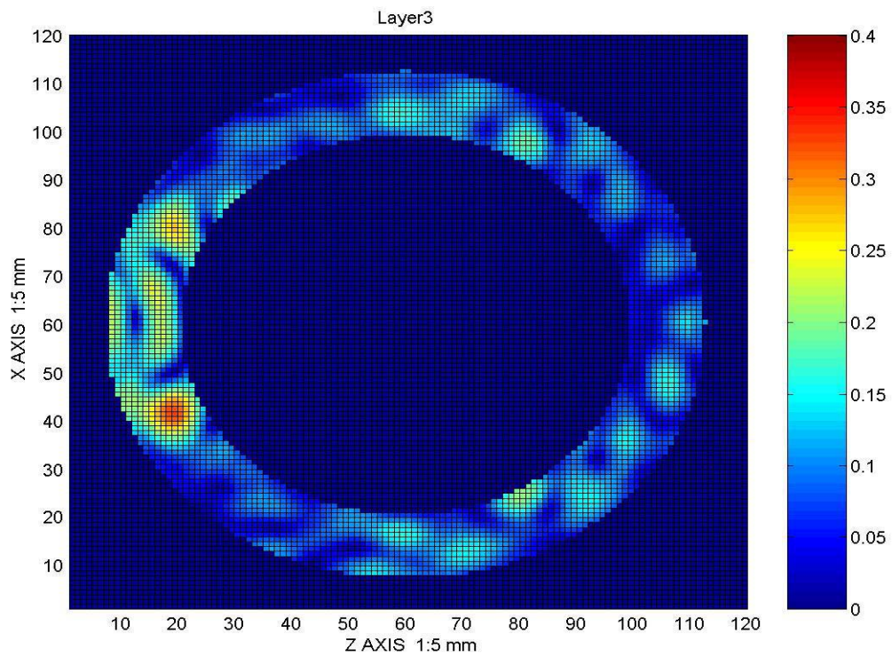
รูปที่ 47 สนามไฟฟ้าภายในวัตถุทรงกระบอกรูปวงแหวนที่ระนาบ XZ ที่ความหนา 80 มิลลิเมตรของวัตถุ
