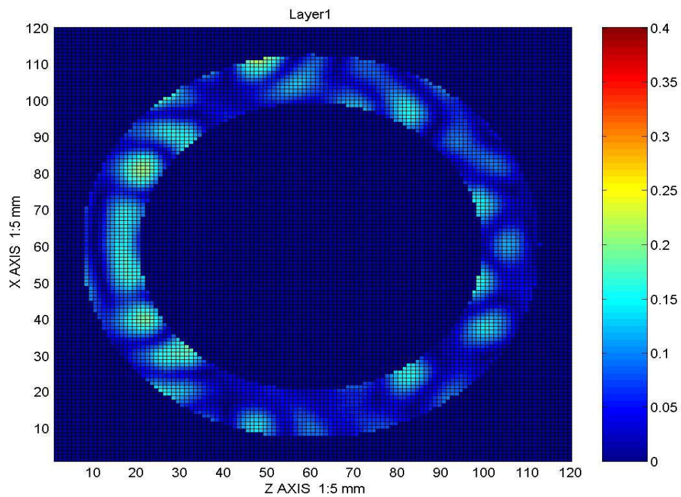
รูปที่ 45 สนามไฟฟ้าภายในวัตถุทรงกระบอกรูปวงแหวนที่ระนาบ XZ ที่ความหนา 0 มิลลิเมตรของวัตถุ
