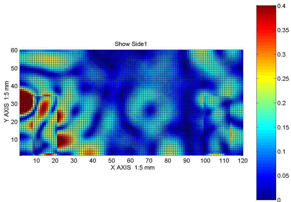
รูปที่ 50 สนามไฟฟ้าภายในวัตถุทรงกระบอกรูปวงแหวนที่ระนาบ XY ที่ Z = 300 มิลลิเมตร
