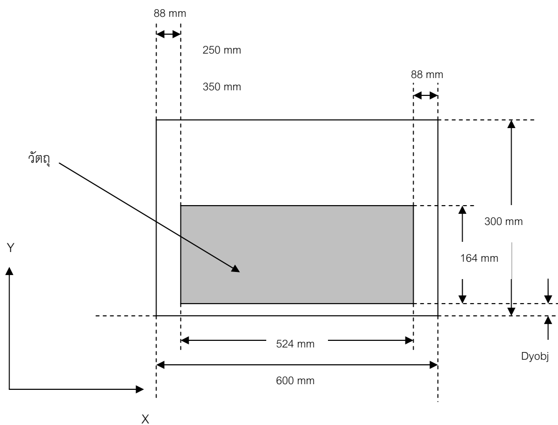
รูปที่ 61 ขนาด ตำแหน่งของท่อนำคลื่น ขนาดของโปรงสี่เหลี่ยม ขนาดของวัตถุ และตำแหน่งการวางวัตถุ
