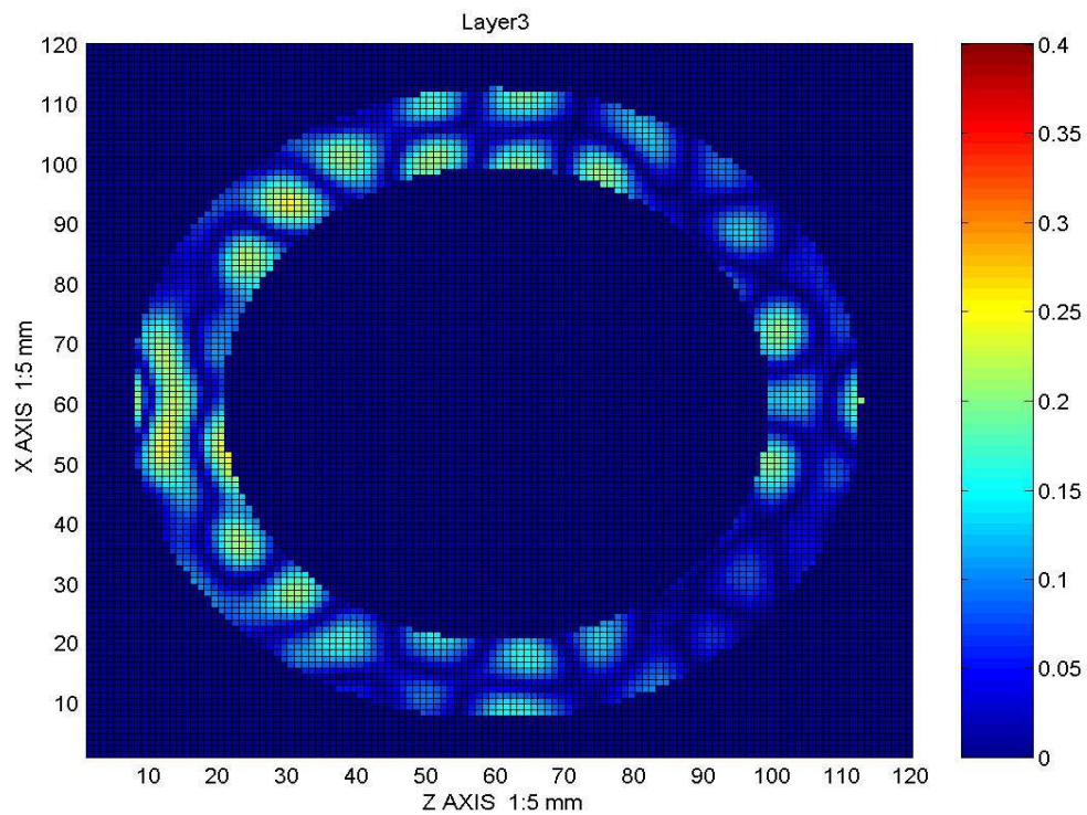
รูปที่ 56 สนามไฟฟ้าภายในวัตถุทรงกระบอกรูปวงแหวนที่ระนาบ XZ ที่ความหนา 80 มิลลิเมตรของวัตถุ
