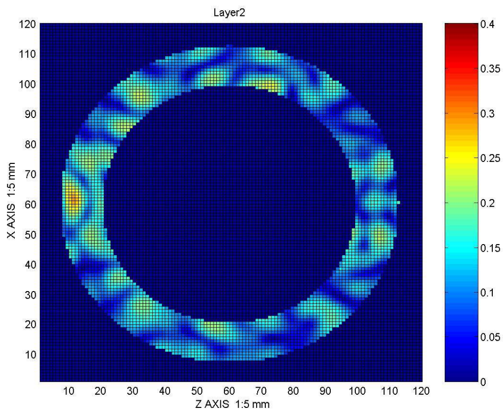
รูปที่ 55 สนามไฟฟ้าภายในวัตถุทรงกระบอกรูปวงแหวนที่ระนาบ XZ ที่ความหนา 40 มิลลิเมตรของวัตถุ
