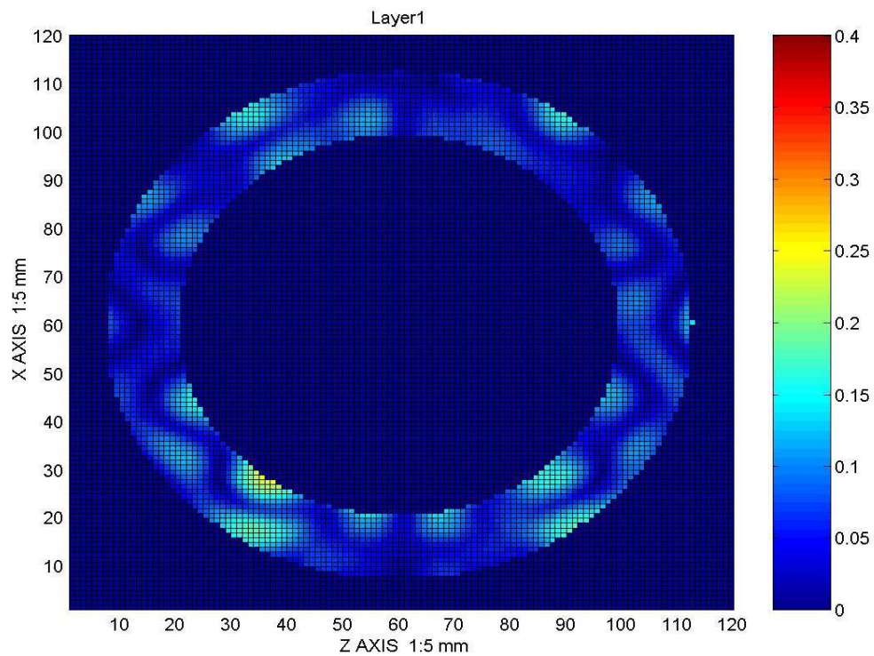
รูปที่ 63 สนามไฟฟ้าภายในวัตถุทรงกระบอกรูปวงแหวนที่ระนาบ XZ ที่ความหนา 0 มิลลิเมตรของวัตถุ
