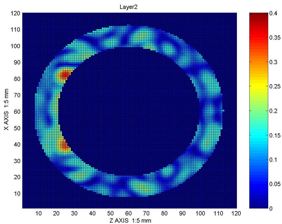
รูปที่ 46 สนามไฟฟ้าภายในวัตถุทรงกระบอกรูปวงแหวนที่ระนาบ XZ ที่ความหนา 40 มิลลิเมตรของวัตถุ
