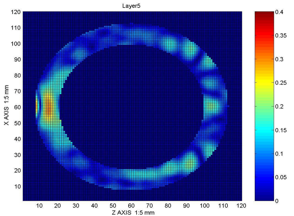
รูปที่ 49 สนามไฟฟ้าภายในวัตถุทรงกระบอกรูปวงแหวนที่ระนาบ XZ ที่ความหนา 160 มิลลิเมตรของวัตถุ
