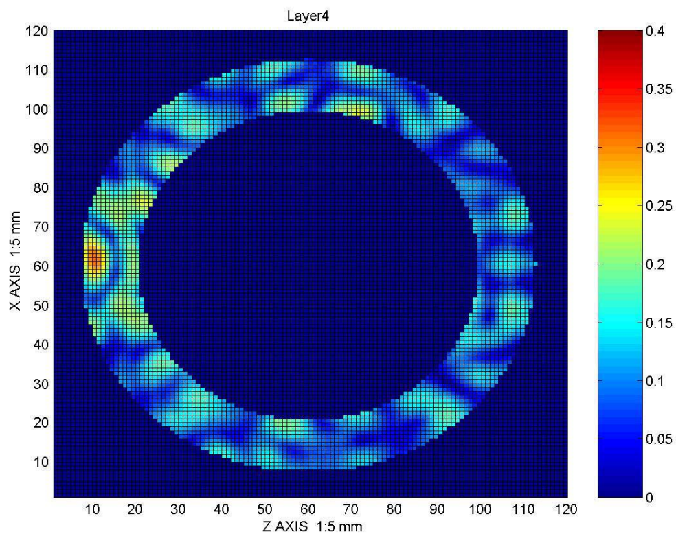
รูปที่ 57 สนามไฟฟ้าภายในวัตถุทรงกระบอกรูปวงแหวนที่ระนาบ XZ ที่ความหนา 120 มิลลิเมตรของวัตถุ
