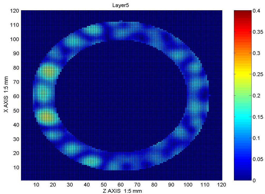
รูปที่ 58 สนามไฟฟ้าภายในวัตถุทรงกระบอกรูปวงแหวนที่ระนาบ XZ ที่ความหนา 160 มิลลิเมตรของวัตถุ
