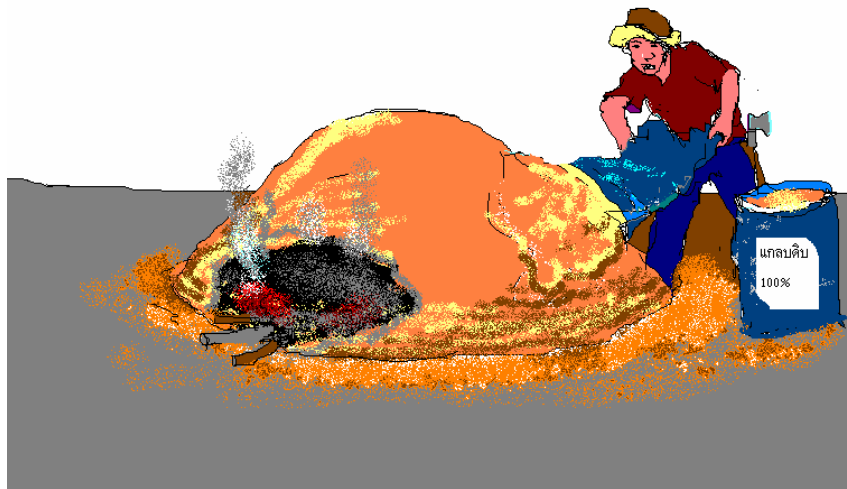
“ภาพที่ 71 การเผาถ่านด้วยแกลบดิบ”
