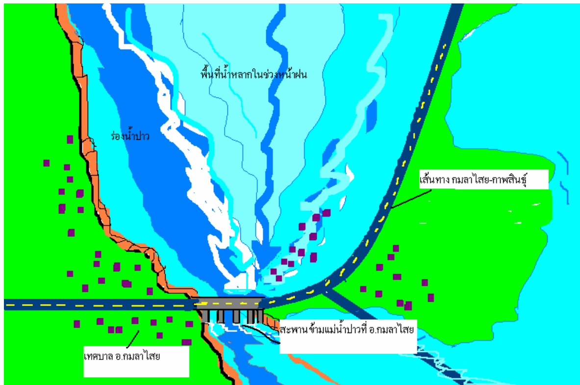
“ภาพที่ 29 ภาพแสดงลักษณะ “คอขวด” ที่บีบให้ช่องทางการไหลของน้ำแคบลง ที่สะพานข้ามแม่น้ำป่าว บริเวณ อำเภอ กมลาไสย”
