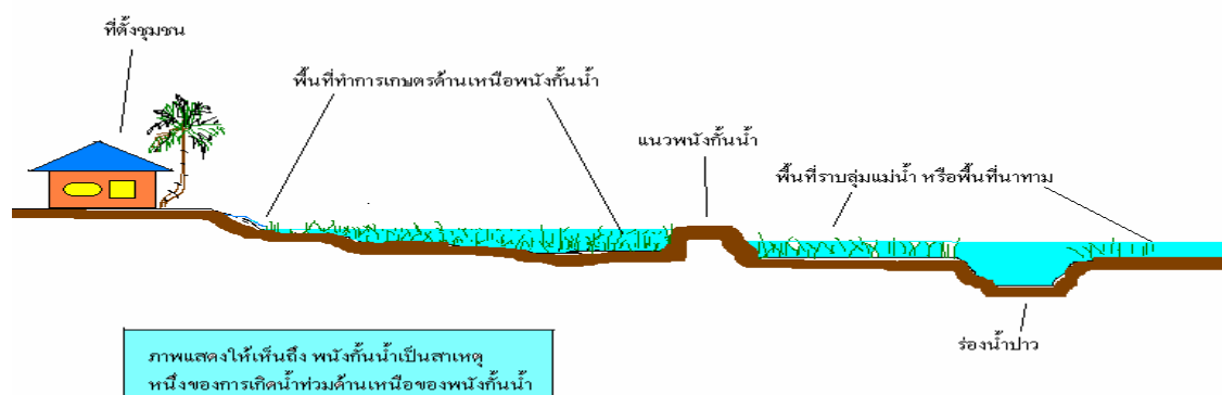
“ภาพที่ 40.ภาพหน้าตัดลักษณะการขวางทางน้ำไหลลงแม่น้ำของพนังกันน้ำ”
