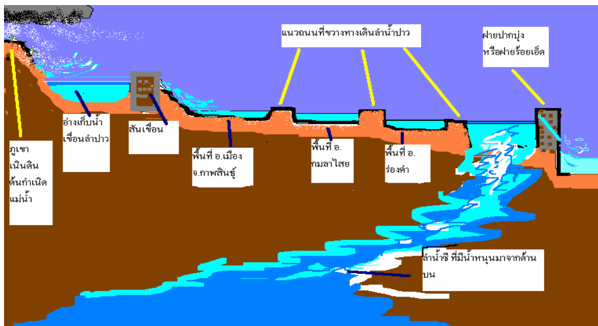
“ภาพที่ 32 ภาพแสดงการไหลของน้ำจาก ลุ่มน้ำปาวที่ต้องผ่านแนวถนนและสิ่งปลูกสร้างต่าง ๆ หลายชั้น ก่อนจะไหลลงสู่ลำน้ำชี”
