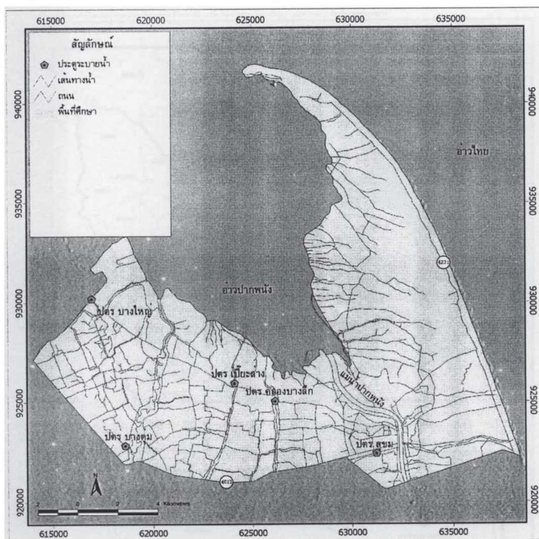
ภาพที่ 5-2 แผนที่ประตูปรับน้ำที่สร้างขึ้นในพื้นที่รอบอ่าง
