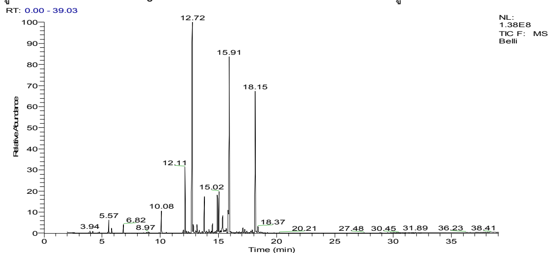
รูปที่ 4 GC/MS Chromatogram องค์ประกอบทางเคมีของน้ำหอมระเหยใบพลู
