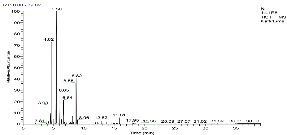
รูปที่ 3 GC/MS Chromatogram องค์ประกอบทางเคมีของน้ำหอมระเหยมะกรูด
