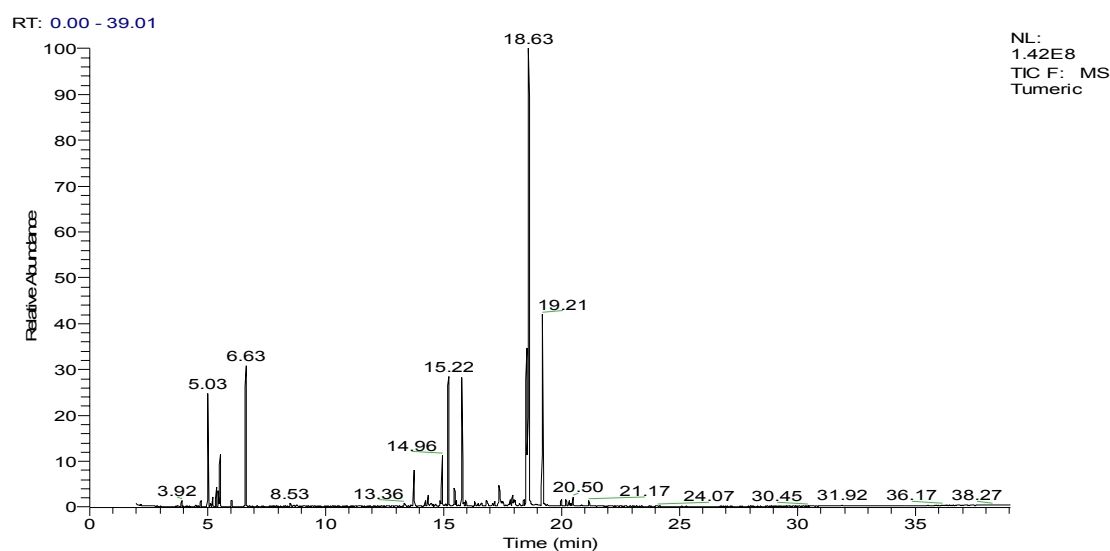
รูปที่ 5 GC/MS Chromatogram องค์ประกอบทางเคมีของน้ำหอมระเหยขมิ้นชัน
