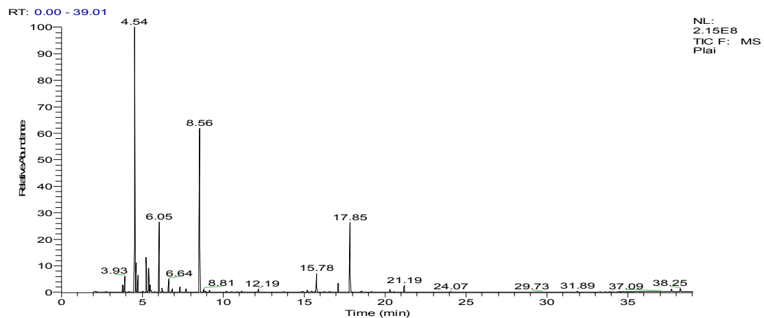
รูปที่ 6 GC/MS Chromatogram องค์ประกอบทางเคมีของน้ำหอมระเหยไพล
