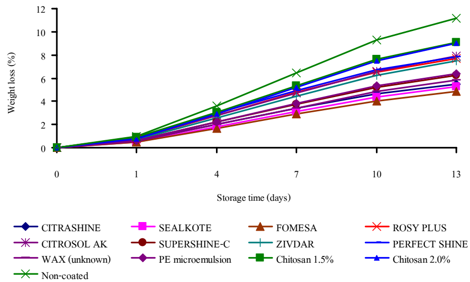
ภาพที่ 3 การเปลี่ยนแปลงการสูญเสียน้ำหนักของผลส้มพันธุ์สายน้ำผึ้งที่เคลือบผิวด้วยสารเคลือบผิวชนิดต่างๆ ระหว่างเก็บรักษาไว้ในอุณหภูมิห้อง ( 23 \pm 3 องศาเซลเซียส) ความชื้นสัมพัทธ์ 56 \pm 5 เปอร์เซ็นต์ เป็นเวลา 13 วัน
