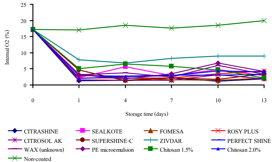
ภาพที่ 4 การเปลี่ยนแปลงปริมาณแก๊สออกซิเจนภายในผลของผลส้มพันธุ์สายน้ำผึ้งที่เคลือบผิวด้วยสารเคลือบผิวชนิดต่างๆ ระหว่างการเก็บรักษาไว้ในอุณหภูมิห้อง ( 23 \pm 3 องศาเซลเซียส) ความชื้นสัมพัทธ์ 56 \pm 5 เปอร์เซ็นต์ เป็นเวลา 13 วัน
