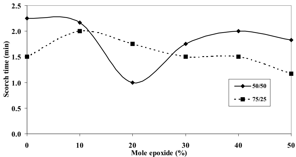
รูปที่ 60 ค่าเวลาสกอร์ชของยางเบลนด์ที่มีปริมาณหมู่อีพอกไซด์ต่างๆ
