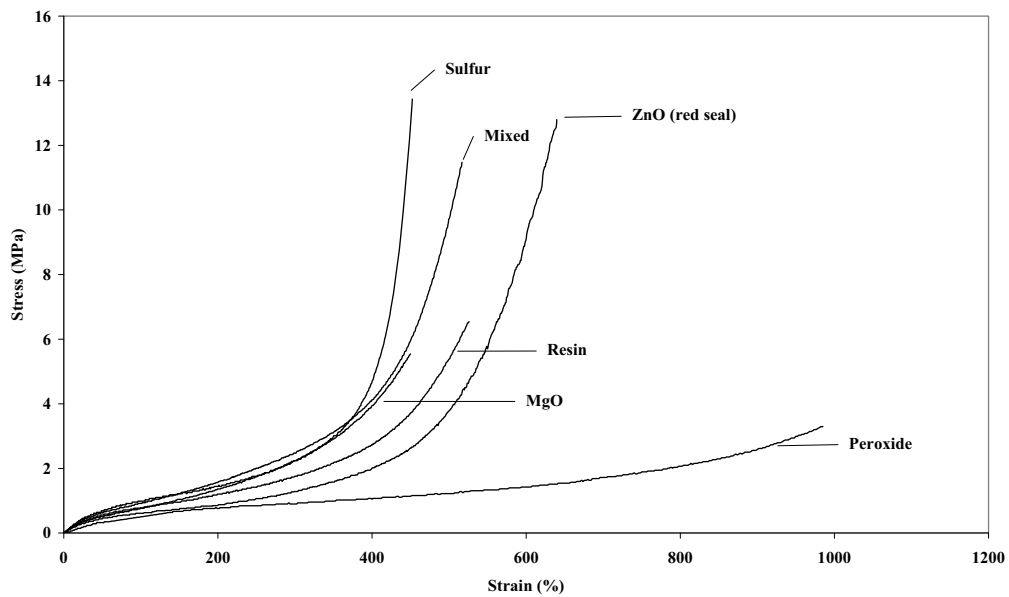
รูปที่ 29 Stress-strain curve ของยางเบลนด NR/CSM ที่ใช้ระบบการวัลคาไนซ์แบบต่างๆ
