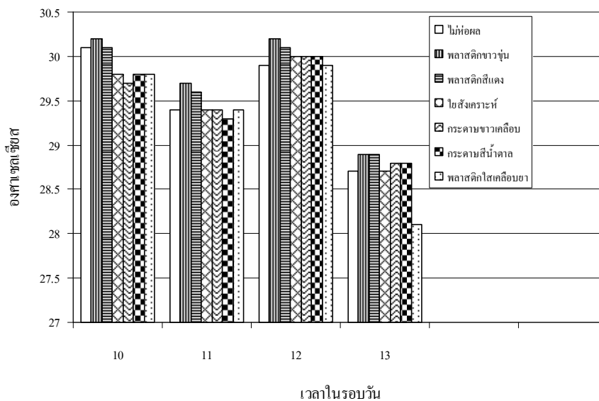
ภาพที่ 6 อุณหภูมิภายในถุงห่อส้มโอที่ทำจากวัสดุชนิดต่าง ๆ ในรอบวัน ในการห่อผลส้มโอพันธุ์ทับทิมสยาม หลังจากดอกบาน 1 เดือน ช่วงเช้ามีแสงแดดปกติ ส่วนช่วงบ่ายมีเมฆครึ้มสลับ (15 พย. 2551)
