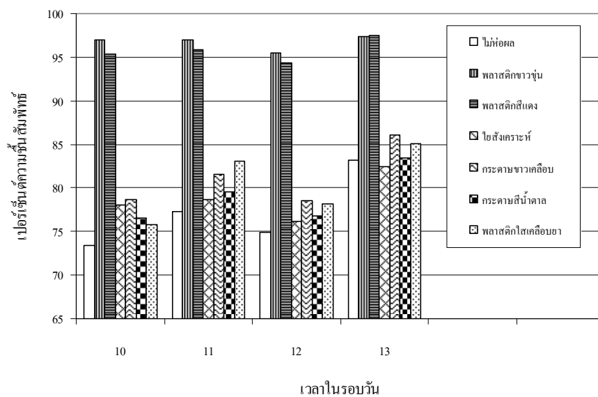
ภาพที่ 8 ความขึ้นสัมพัทธ์ภายในถุงห่อสัมโอที่ทำจากวัสดุชนิดต่าง ๆ ในรอบวัน ในการห่อผลส้มโอพันธุ์ทับทิมสยาม หลังจากดอกบาน 1 เดือน ช่วงเช้ามีแสงแดดปกติ ส่วนช่วงบ่ายมีเมฆครึ้มสลับ (15 พย. 2551)
