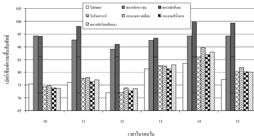
ภาพที่ 7 ความขึ้นสัมพัทธ์ภายในถุงห่อสัมโอที่ทำจากวัสดุชนิดต่าง ๆ ในรอบวัน ในการห่อผลส้มโอพันธุ์ทองดี หลังจากดอกบาน 1 เดือน ช่วงเช้ามีแสงแดดปกติ ส่วนช่วงบ่ายมีเมฆครึ้มสลับ (15 พย. 2551)
