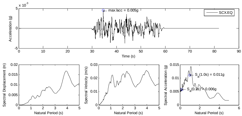
รูปที่ 3.14 ประวัติเวลาและสเปกตรัมของคลื่นแผ่นดินไหว San Fernando จากสถานีวัด Cholame-Shandon Array #2
