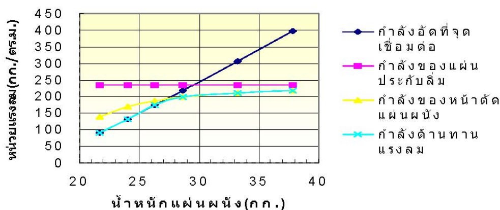
ภาพที่ 3.12 แผนภูมิองค์ประกอบควบคุมกำลังของแผ่นผนัง
