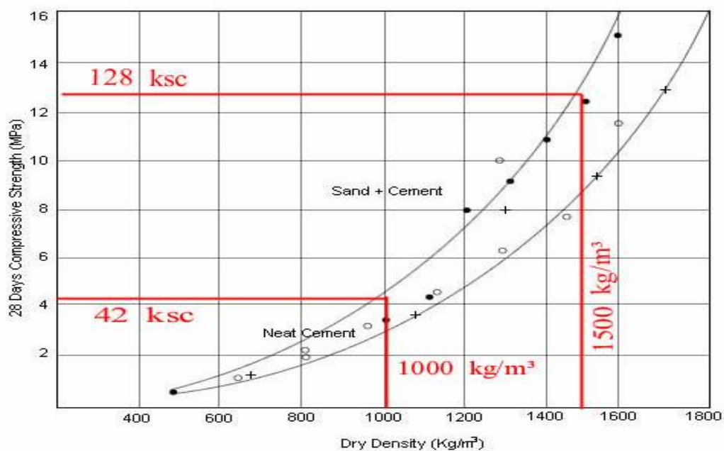
ภาพที่ 3.6 แสดงกราฟเปรียบเทียบค่ากำลังอัดประลัย (ผู้ผลิตในต่างประเทศ)
