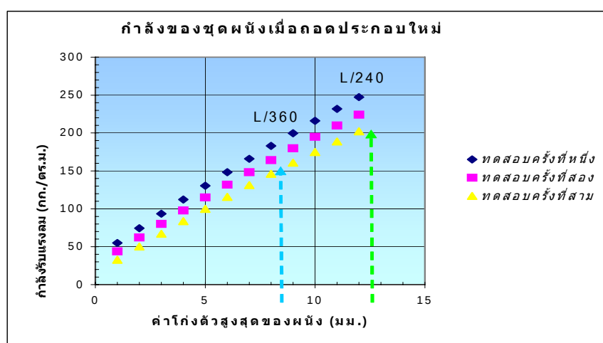
ภาพที่ 4.4 ความสัมพันธ์กำลังรับแรงลมกับค่าโก่งตัวของผนังโดยการถอดประกอบสามครั้ง
