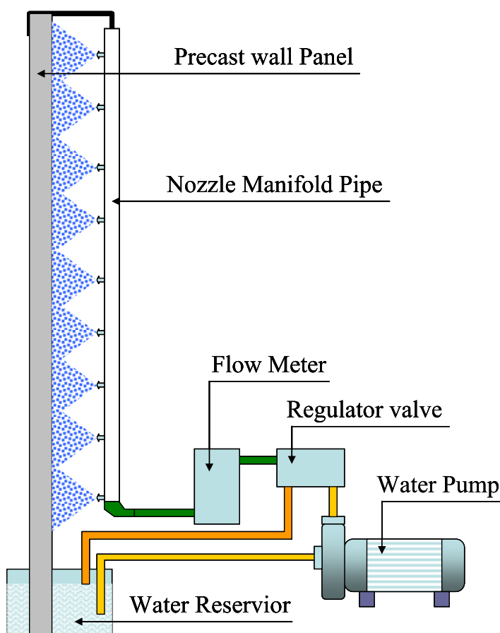
ภาพที่ 4.8 แสดงรูปด้านข้างของชุดผนังและระบบทดสอบความต้านทานการซึมผ่านของน้ำฝน
