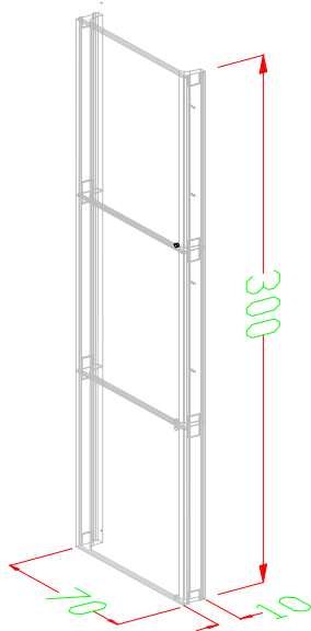
ภาพที่ 4.1 มิติของผนังตัวอย่างที่ใช้ทดสอบ(ชม.)
