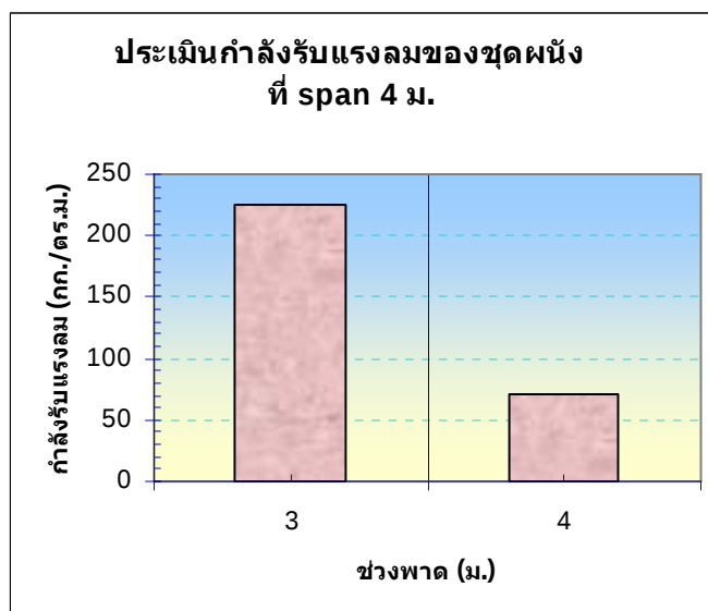
ภาพที่ 4.5 การใช้ค่าความต้านแรงดัดประสมประเมินกำลังรับแรงลมที่ช่วงพาด 4 ม.
