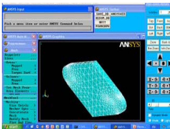
ภาพที่ 3.10 ภาพการวิเคราะห์ชุดต่อผนังโดยโปรแกรมไฟไนต์เอลิเมนต์
