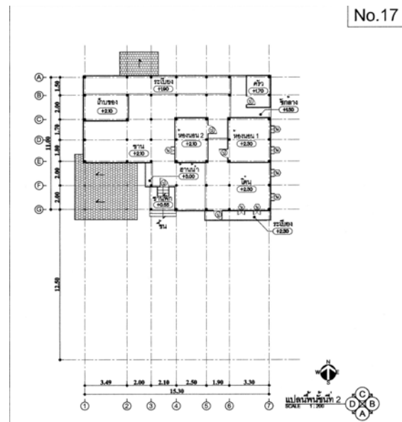
ภาพที่ 4.132 แสดงแปลนพื้นชั้นบน หลังที่ 17 ชุมชนพริ้วหนุ่ม ที่มา : จากการสำรวจ ปี พ.ศ.2552
