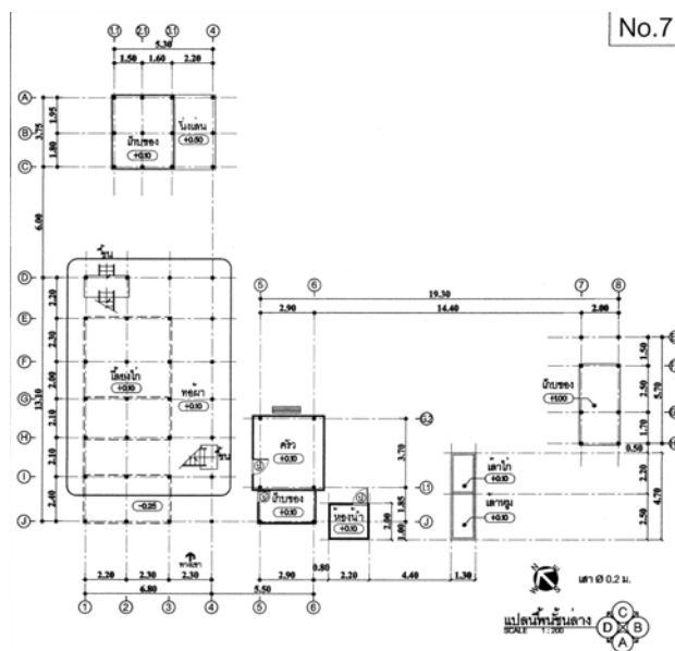
ภาพที่ 4.58 แสดงแปลนพื้นชั้นล่าง หลังที่ 7 ชุมชนนาเรือน
