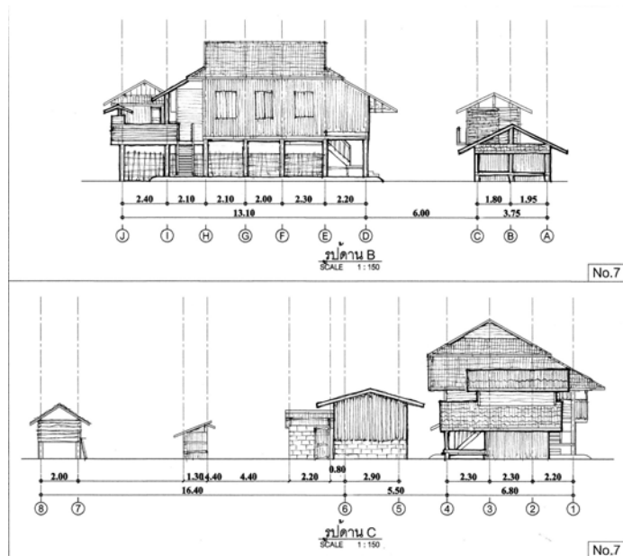
ภาพที่ 4.61 แสดงรูปด้าน B รูปด้าน C หลังที่ 7 ชุมชนนาเรือน ที่มา : จากการสำรวจ ปี พ.ศ. 2551
