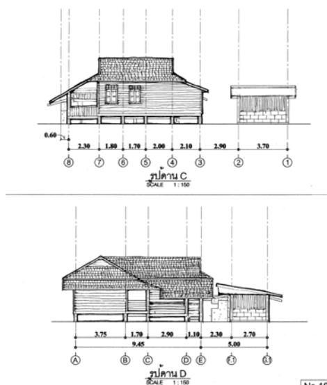
ภาพที่ 4.126 แสดงรูปด้าน C รูปด้าน D หลังที่ 16 ชุมชนพริ้วหนุ่ม ที่มา : จากการสำรวจ ปี พ.ศ. 2552
