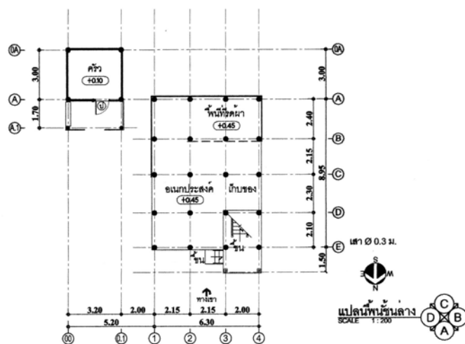
ภาพที่ 4.21 แสดงแปลนพื้นที่ชั้นล่าง หลังที่ 2 ชุมชนพรวัวหนุ่ม
