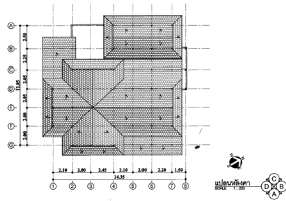
ภาพที่ 4.76 แสดงแปลนหลังคา หลังที่ 10 ชุมชนพร้าวหม่ม ที่มา : จากการสำรวจ ปี พ.ศ. 2552
