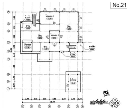
ภาพที่ 4.161 แสดงผังพื้นที่ชั้นบน หลังที่ 21 ชุมชนบ้านอาราม ที่มา : จากการสำรวจ ปี พ.ศ. 2552
