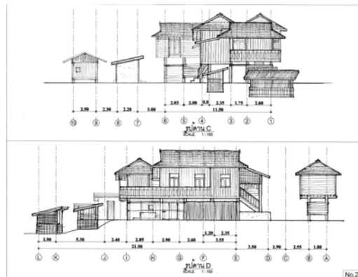
ภาพที่ 4.169 แสดงรูปด้าน D C หลังที่ 23 ชุมชนบ้านยางหลวง ที่มา : จากการสำรวจ ปี พ.ศ. 2552
