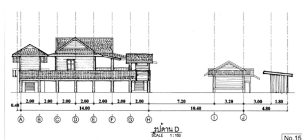
ภาพที่ 4.119 แสดงรูปด้าน D หลังที่ 15 ชุมชนพริ้วหนุ่ม ที่มา : จากการสำรวจ ปี พ.ศ. 2552
