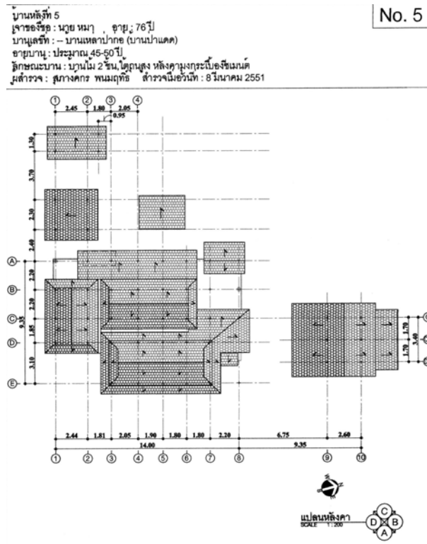
ภาพที่ 4.41 แสดงแปลนหลังคา หลังที่ 5 ชุมชนเหล่าปากอ (ป่าแดด) ที่มา : จากการสำรวจ ปี พ.ศ. 2551
