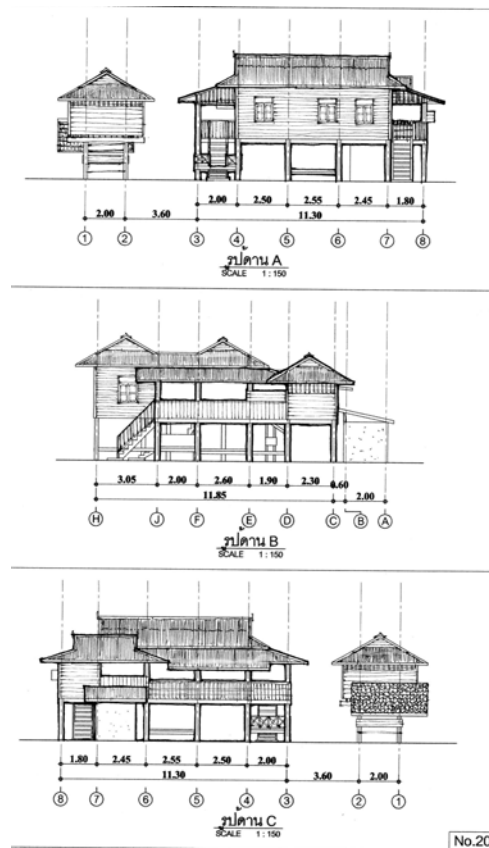
ภาพที่ 4.157 แสดงรูปด้าน A, B, C หลังที่ 20 ชุมชนบ้านอาราม ที่มา : จากการสำรวจ ปี พ.ศ. 2552
