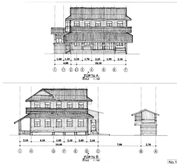
ภาพที่ 4.149 แสดงรูปด้าน A รูปด้าน B หลังที่ 19 ชุมชนพริ้วหนุ่ม ที่มา : จากการสำรวจ ปี พ.ศ. 2552
