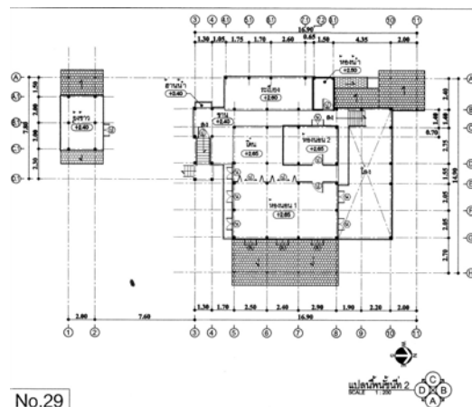
ภาพที่ 4.186 แสดงแปลนพื้นที่ชั้นบน หลังที่ 29 ชุมชนบ้านต้นตาล ที่มา : จากการสำรวจ ปี พ.ศ. 2552
