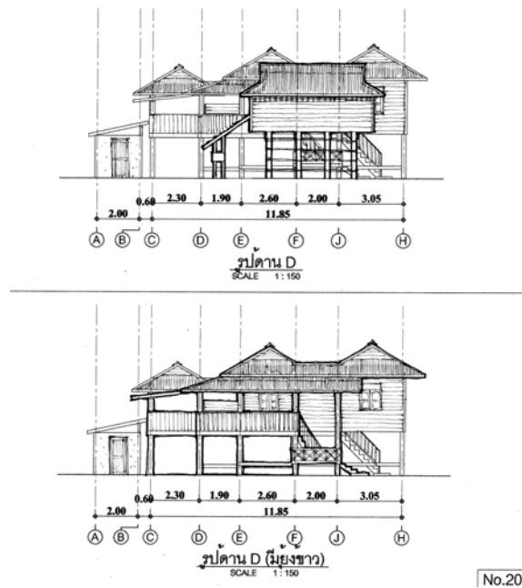
ภาพที่ 4.158 แสดงรูปด้าน D หลังที่ 20 ชุมชนบ้านอาราม ที่มา : จากการสำรวจ ปี พ.ศ. 2552
