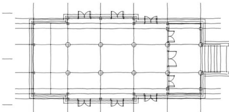
- ผังวิหารวัดพุทธเอ้น -
