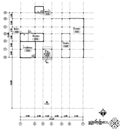
ภาพที่ 4.131 แสดงแปลนพื้นที่ชั้นล่าง หลังที่ 17 ชุมชนพร้าวหนุ่ม
