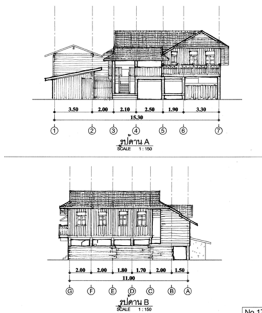
ภาพที่ 4.133 แสดงรูปด้าน A รูปด้าน B หลังที่ 17 ชุมชนพริ้วหนุ่ม ที่มา : จากการสำรวจ ปี พ.ศ. 2552
