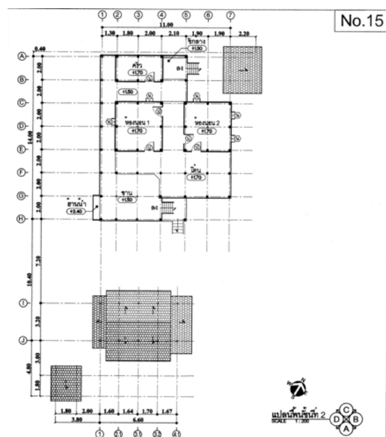
ภาพที่ 4.116 แสดงแปลนพื้นที่ชั้นบน หลังที่ 15 ชุมชนพริ้วหนุ่ม ที่มา : จากการสำรวจ ปี พ.ศ. 2552
