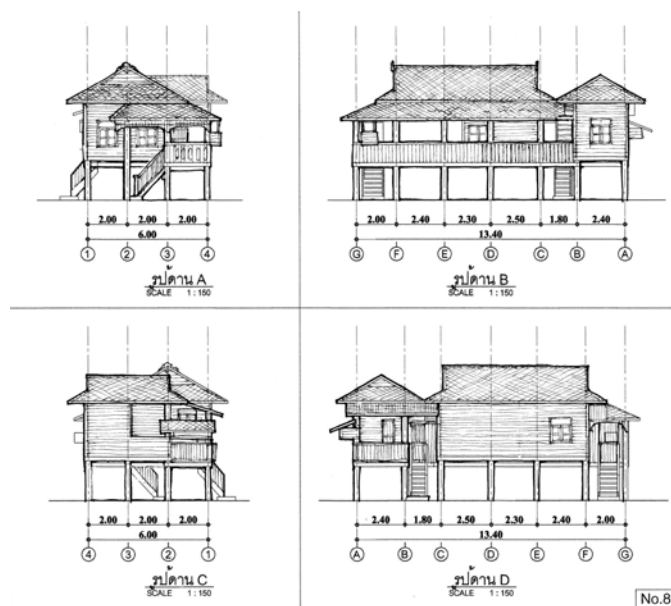
ภาพที่ 4.66 แสดงรูปด้าน หลังที่ 8 ชุมชนนาเรือน
