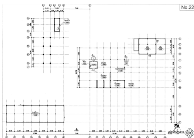
ภาพที่ 4.164 แสดงแปลนพื้นชั้นบน หลังที่ 22 ชุมชนบ้านเหล่า
