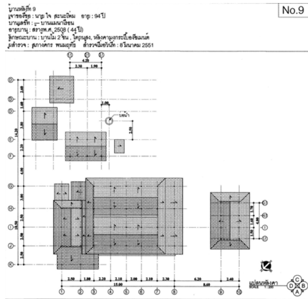
ภาพที่ 4.69 แสดงแปลนหลังคา หลังที่ 9 ชุมชนนาเรือน
