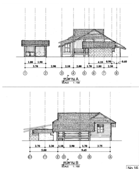
ภาพที่ 4.125 แสดงรูปด้าน A รูปด้าน B หลังที่ 16 ชุมชนพริ้วหนุ่ม ที่มา : จากการสำรวจ ปี พ.ศ. 2552
