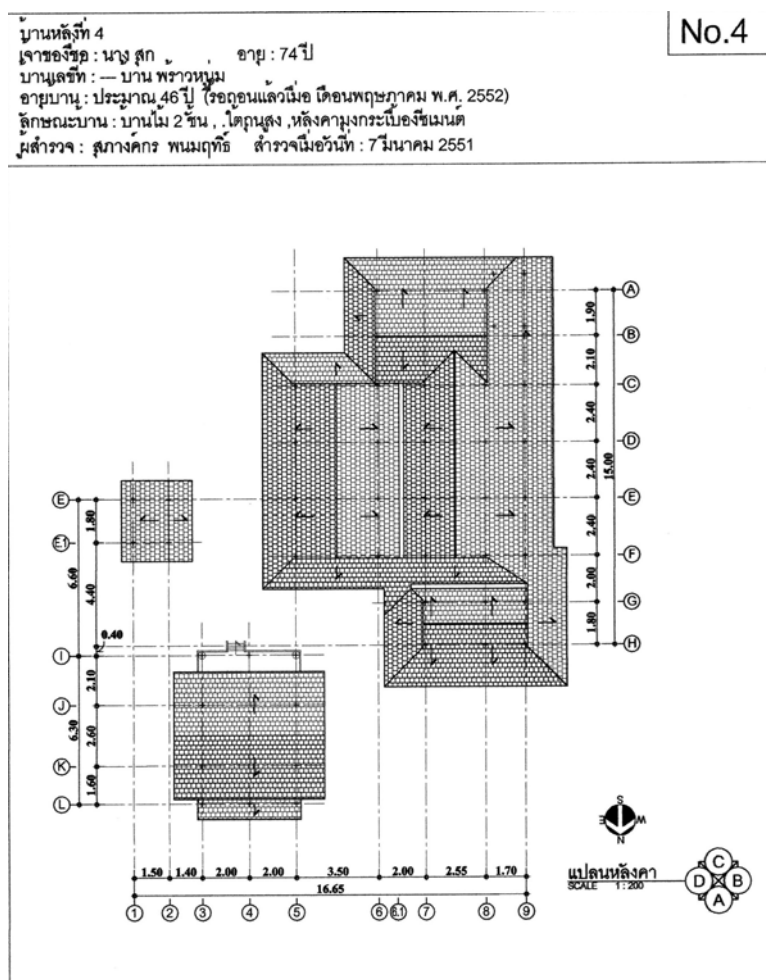
ภาพที่ 4.33 แสดงแปลนหลังคา หลังที่ 4 ชุมชนพร้าวหนุ่ม ที่มา : จากการสำรวจ ปี พ.ศ. 2551
