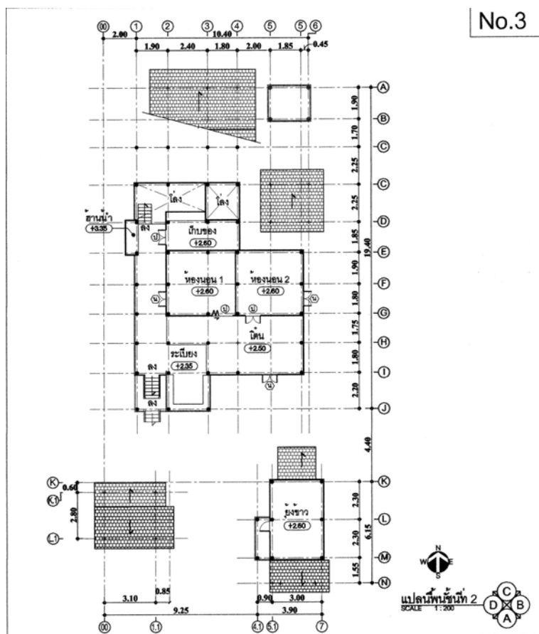
ภาพที่ 4.28 แสดงแปลนพื้นที่ชั้นบน หลังที่ 3 ชุมชนพรวัวหนุ่ม
