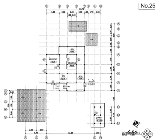
ภาพที่ 4.174 แสดงแปลนพื้นที่บน หลังที่ 25 ชุมชนบ้านไร่ ที่มา : จากการสำรวจ ปี พ.ศ. 2552
