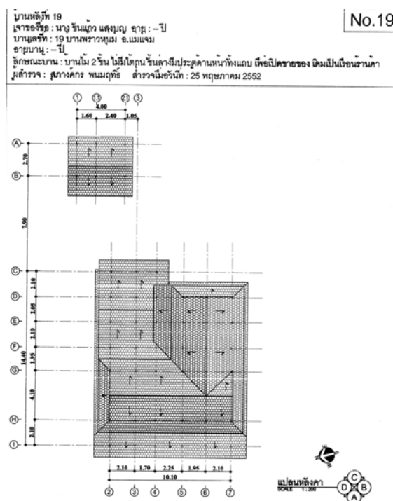
ภาพที่ 4.146 แสดงแปลนหลังคา หลังที่ 19 ชุมชนพรวัวหนุ่ม
