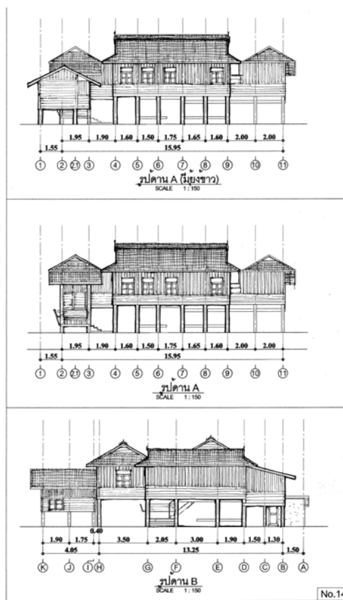
ภาพที่ 4.109 แสดงรูปด้าน A รูปด้าน B หลังที่ 14 ชุมชนพริ้วหนุ่ม ที่มา : จากการสำรวจ ปี พ.ศ. 2552
