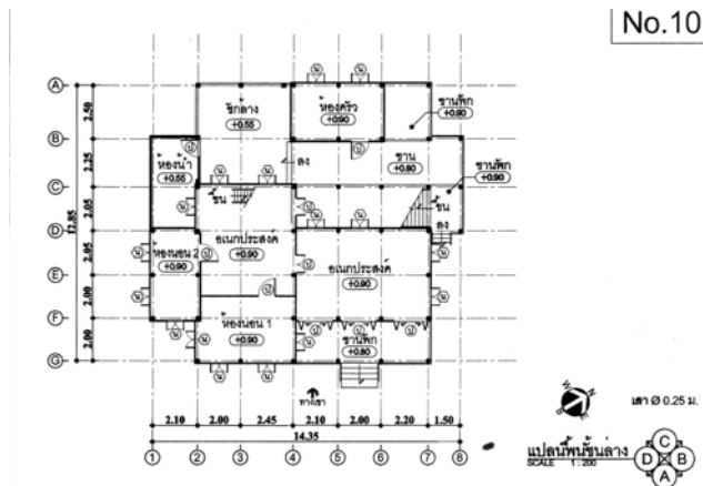
ภาพที่ 4.77 แสดงแปลนพื้นที่ชั้นล่าง หลังที่ 10 ชุมชนพร้าวหม่ม ที่มา : จากการสำรวจ ปี พ.ศ. 2552
