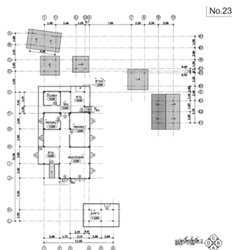
ภาพที่ 4.168 แสดงแปลนพื้นชั้นบนหลังที่ 23 ชุมชนบ้านยางหลวง
