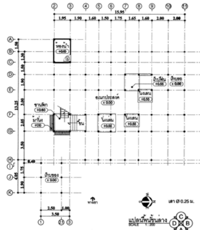
ภาพที่ 4.107 แสดงแปลนพื้นชั้นล่าง หลังที่ 14 ชุมชนพริ้วหนุ่ม ที่มา : จากการสำรวจ ปี พ.ศ. 2552
