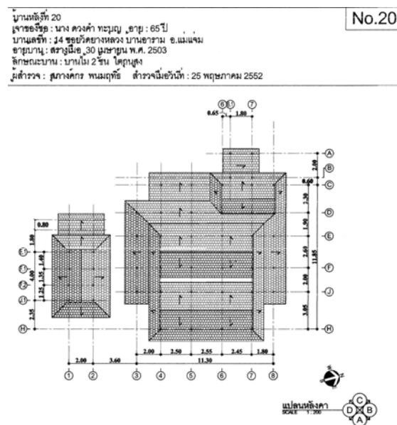
ภาพที่ 4.154 แสดงแปลนหลังคา หลังที่ 20 ชุมชนบ้านอาราม ที่มา : จากการสำรวจ ปี พ.ศ. 2552
