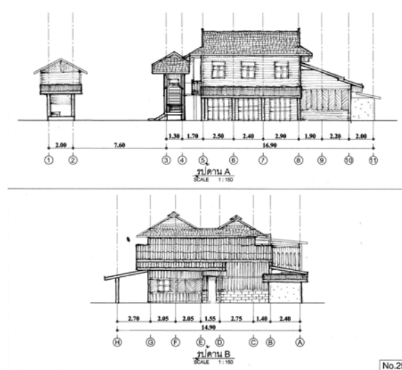
ภาพที่ 4.187 แสดงรูปด้าน A รูปด้าน B หลังที่ 29 ชุมชนบ้านต้นตาล ที่มา : จากการสำรวจ ปี พ.ศ. 2552
