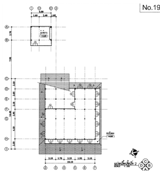
ภาพที่ 4.148 แสดงแปลนพื้นชั้นบน หลังที่ 19 ชุมชนพริ้วหนุ่ม ที่มา : จากการสำรวจ ปี พ.ศ.2552
