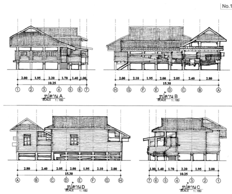
ภาพที่ 4.17 แสดงรูปด้าน หลังที่1 ชุมชนพริ้วหนุ่ม
