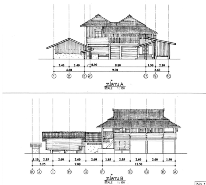
ภาพที่ 4.87 แสดงรูปด้าน A รูปด้าน B หลังที่ 11 ชุมชนพร้าวหนุ่ม
