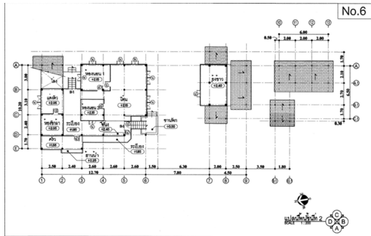
ภาพที่ 4.51 แสดงแปลนพื้นชั้นบน หลังที่ 6 ชุมชนเหล่าปากอ(ป่าแดด)
