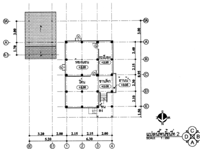
ภาพที่ 4.22 แสดงแปลนพื้นที่ชั้นบน หลังที่ 2 ชุมชนพรวัวหนุ่ม
