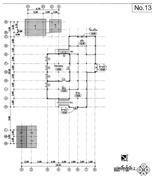
ภาพที่ 4.101 แสดงแปลนพื้นชั้นบน หลังที่ 13 ชุมชนบ้านเหล่า ที่มา : จากการสำรวจ ปี พ.ศ. 2552
