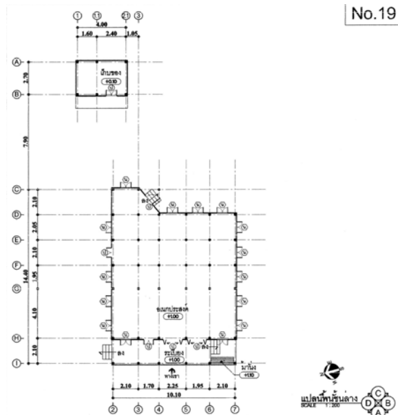
ภาพที่ 4.147 แสดงแปลนพื้นชั้นล่าง หลังที่ 19 ชุมชนพริ้วหนุ่ม ที่มา : จากการสำรวจ ปี พ.ศ.2552
