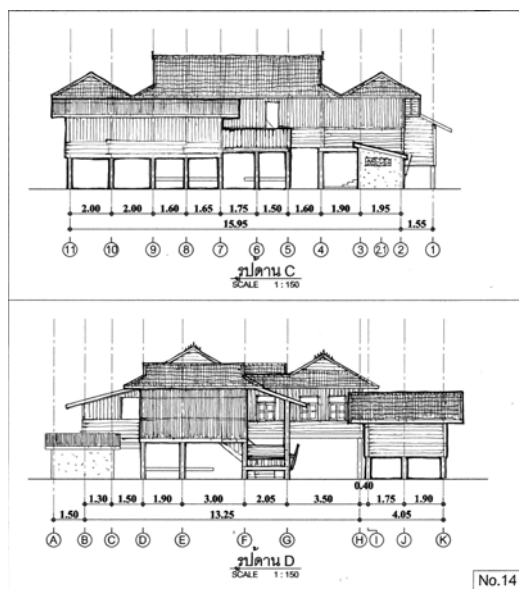
ภาพที่ 4.110 แสดงรูปด้าน C รูปด้าน D หลังที่ 14 ชุมชนพริ้วหนุ่ม ที่มา : จากการสำรวจ ปี พ.ศ. 2552
