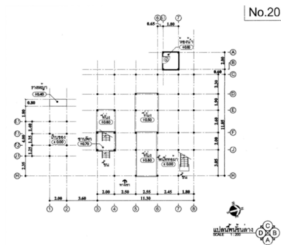
ภาพที่ 4.155 แสดงแปลนพื้นชั้นล่าง หลังที่ 20 ชุมชนบ้านอาราม ที่มา : จากการสำรวจ ปี พ.ศ. 2552
