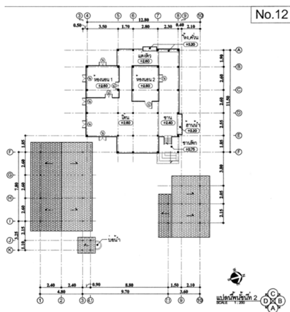
ภาพที่ 4.93 แสดงแปลนชั้นบน หลังที่ 12 ชุมชนพัวหมื่น ที่มา : จากการสำรวจ ปี พ.ศ. 2552
