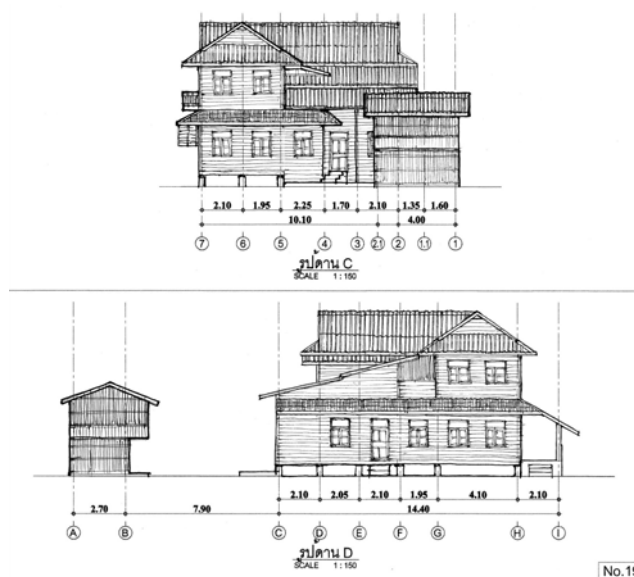
ภาพที่ 4.150 แสดงรูปด้าน C รูปด้าน D หลังที่ 19 ชุมชนพริ้วหนุ่ม ที่มา : จากการสำรวจ ปี พ.ศ. 2552
