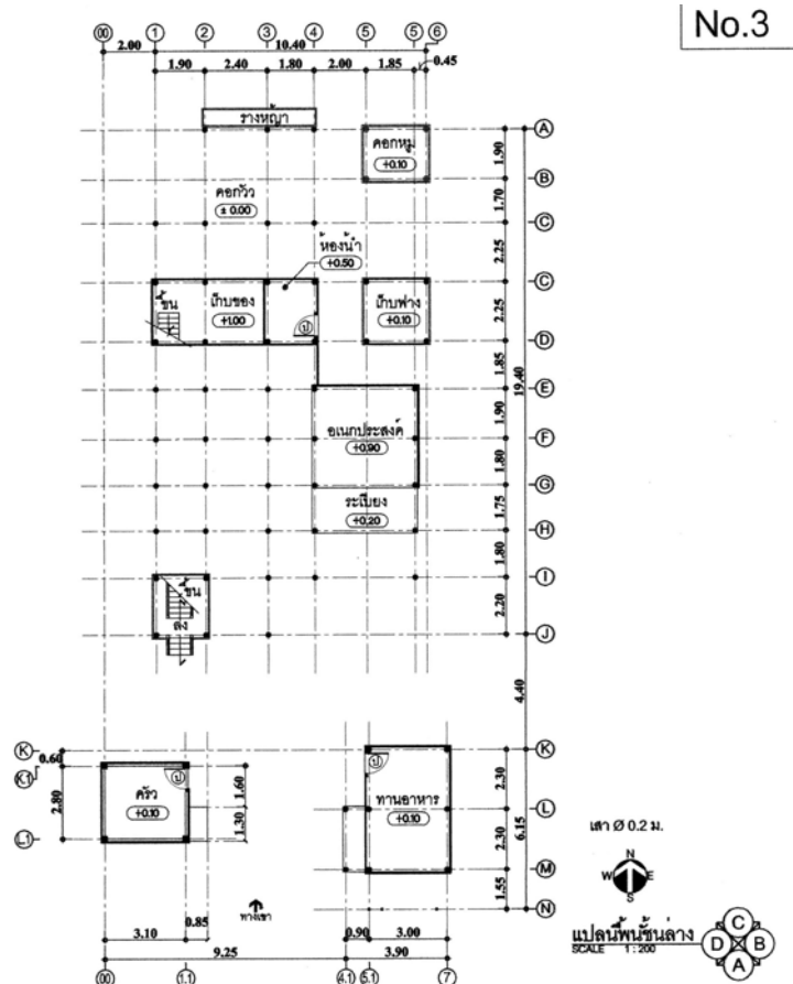
ภาพที่ 4.27 แสดงแปลนพื้นที่ชั้นล่าง หลังที่ 3 ชุมชนพริ้วหนุ่ม ที่มา : จากการสำรวจ ปี พ.ศ. 2551
