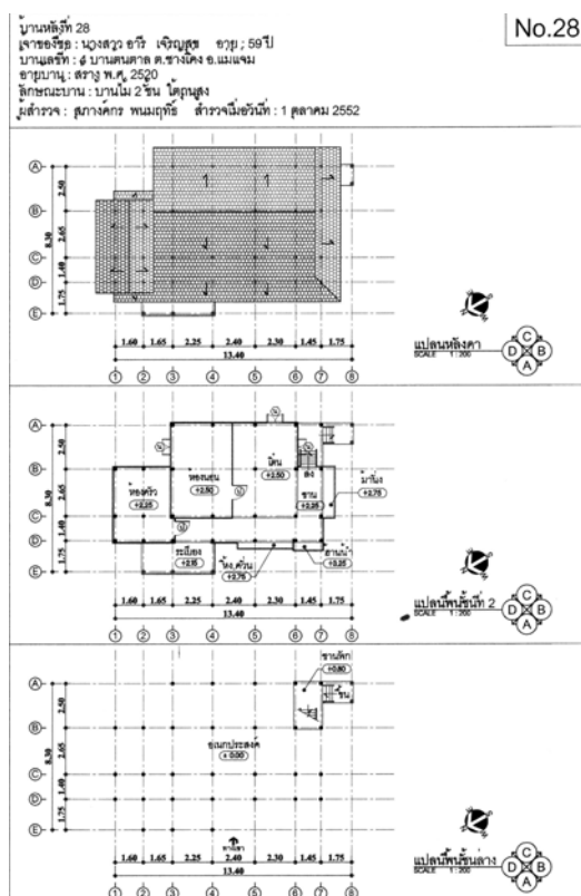
ภาพที่ 4.183 แสดงแปลนพื้นที่บ้าน หลังที่ 28 ชุมชนบ้านต้นตาล
