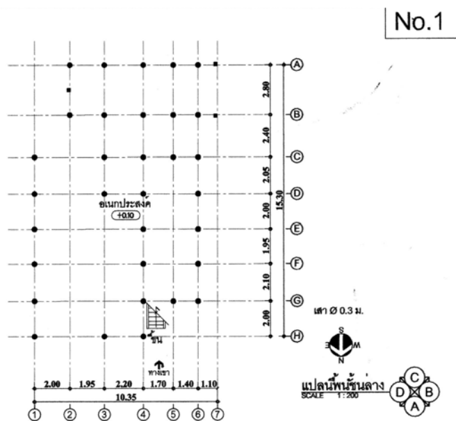
ภาพที่ 4.15 แสดงแปลนพื้นที่ชั้นล่าง หลังที่ 1 ชุมชนพรวัวหนุ่ม ที่มา : จากการสำรวจ ปี พ.ศ. 2551
