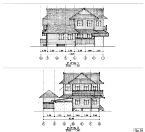
ภาพที่ 4.80 แสดงรูปด้าน C รูปด้าน D หลังที่ 10 ชุมชนพรวัวหนุ่ม
