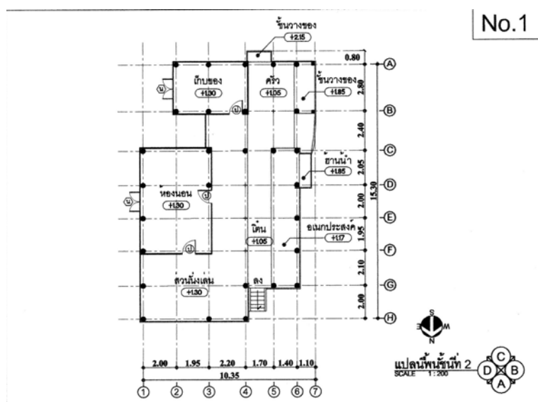
ภาพที่ 4.16 แสดงแปลนพื้นที่ชั้นบน หลังที่ 1 ชุมชนพรวัวหนุ่ม ที่มา : จากการสำรวจ ปี พ.ศ. 2551
