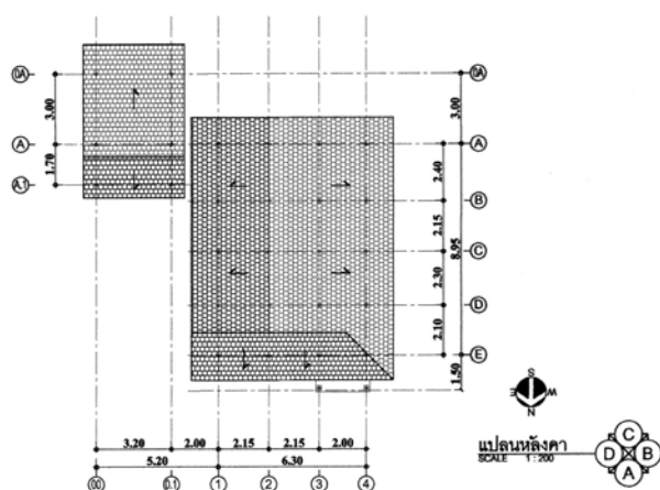
ภาพที่ 4.20 แสดงแปลนหลังคา หลังที่ 2 ชุมชนพรวัวหนุ่ม
