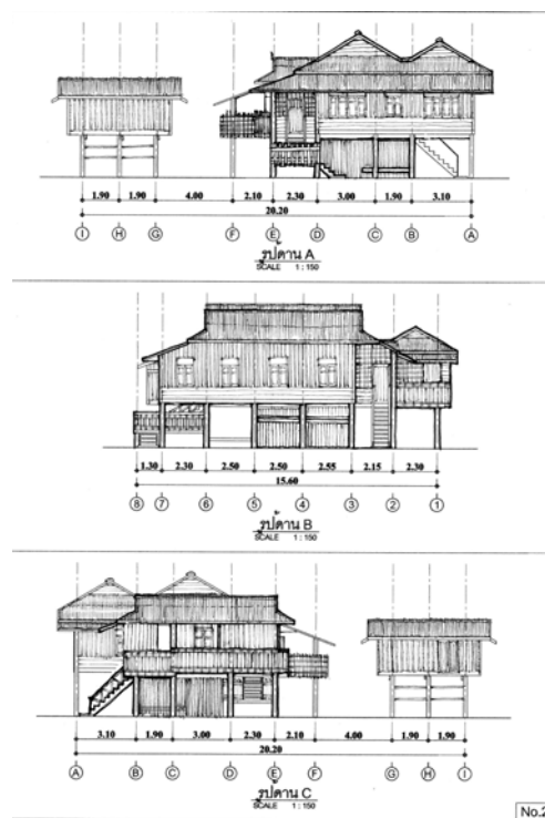
ภาพที่ 4.162 แสดงรูปด้าน A B C หลังที่ 21 ชุมชนบ้านอาราม ที่มา : จากการสำรวจ ปี พ.ศ. 2552
