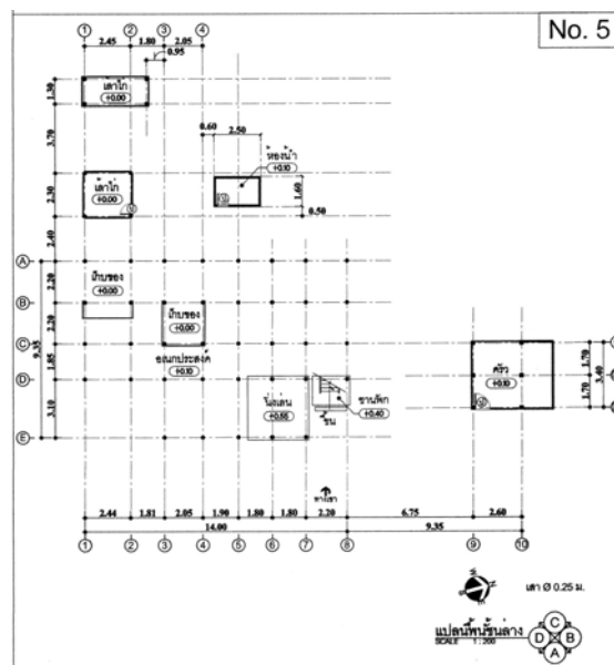
ภาพที่ 4.42 แสดงแปลนพื้นชั้นล่าง หลังที่ 5 ชุมชนเหล่าปากอ (ป่าแดด) ที่มา : จากการสำรวจ ปี พ.ศ. 2551
