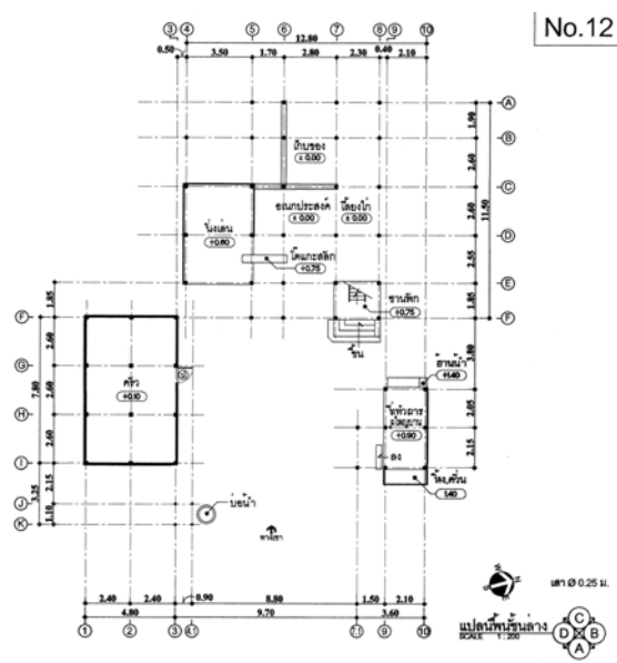
ภาพที่ 4.92 แสดงแปลนชั้นล่าง หลังที่ 12 ชุมชนพริ้วหนุ่ม ที่มา : จากการสำรวจ ปี พ.ศ. 2552
