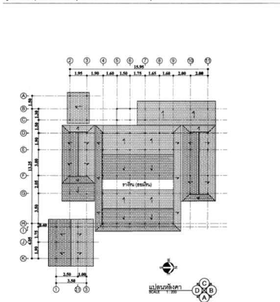
ภาพที่ 4.106 แสดงแปลนหลังคา หลังที่ 14 ชุมชนพร้าวหนุ่ม
