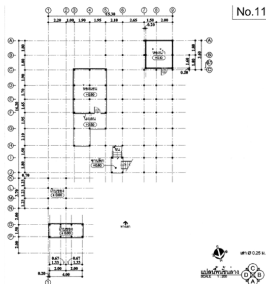
ภาพที่ 4.85 แสดงแปลนชั้นล่าง หลังที่ 11 ชุมชนพรวนหมื่น ที่มา : จากการสำรวจ ปี พ.ศ. 2552
