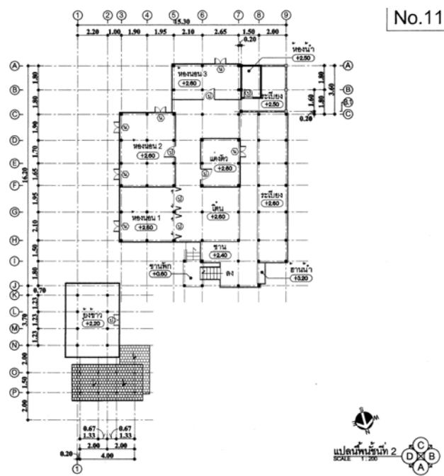
ภาพที่ 4.86 แสดงแปลนชั้นบน หลังที่ 11 ชุมชนพร้าวหนุ่ม
