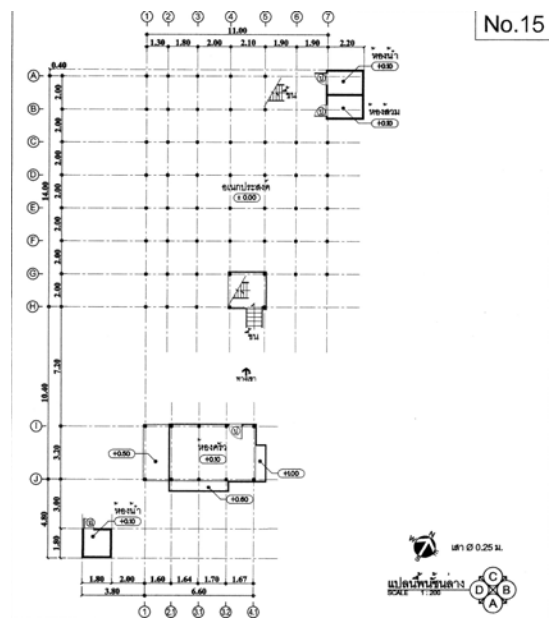
ภาพที่ 4.115 แสดงแปลนพื้นที่ชั้นล่าง หลังที่ 15 ชุมชนพริ้วหนุ่ม ที่มา : จากการสำรวจ ปี พ.ศ. 2552
