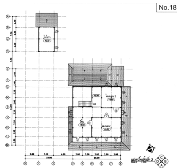
ภาพที่ 4.140 แสดงแปลนพื้นที่ชั้นบน หลังที่ 18 ชุมชนพร้าวหนุ่ม ที่มา : จากการสำรวจ ปี พ.ศ.2552
