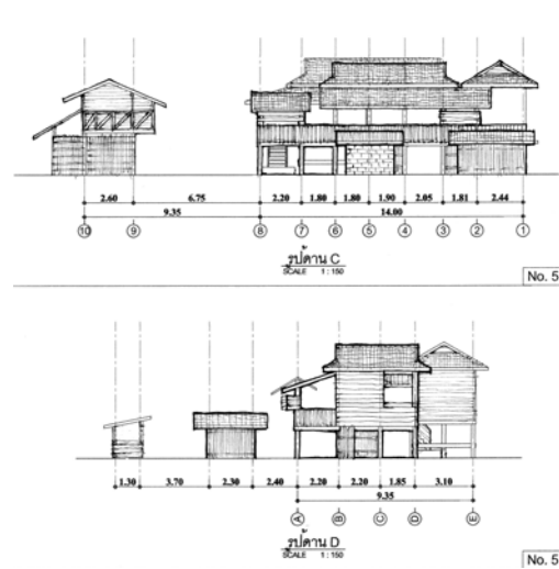
ภาพที่ 4.45 แสดงรูปด้าน C รูปด้าน D หลังที่ 5 ชุมชนเหล่าปากอ (ป่าแดด) ที่มา : จากการสำรวจ ปี พ.ศ. 2551
