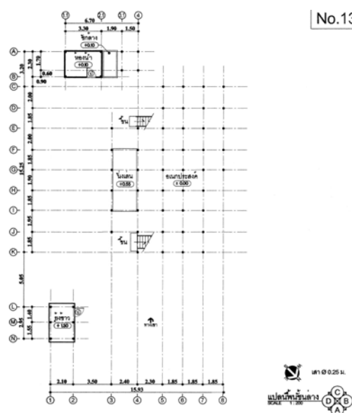
ภาพที่ 4.100 แสดงแปลนพื้นที่ชั้นล่าง หลังที่ 13 ชุมชนบ้านเหล่า ที่มา : จากการสำรวจ ปี พ.ศ. 2552
