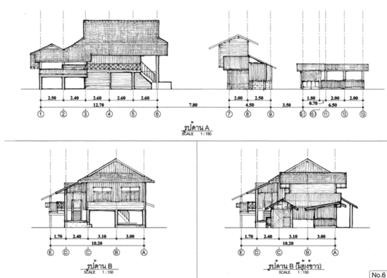
ภาพที่ 4.52 แสดงรูปด้าน A รูปด้าน B หลังที่ 6 ชุมชนเหล่าปากอ(ป่าแดด)
