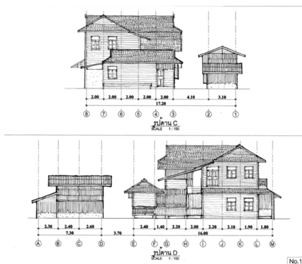
ภาพที่ 4.141 แสดงรูปด้าน C รูปด้าน D หลังที่ 18 ชุมชนพร้าวหนุ่ม ที่มา : จากการสำรวจ ปี พ.ศ. 2552
