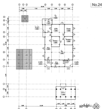
ภาพที่ 4.171 แสดงแปลนพื้นที่ชั้นบน หลังที่ 24 ชุมชนบ้านไร่ ที่มา : จากการสำรวจ ปี พ.ศ. 2552
