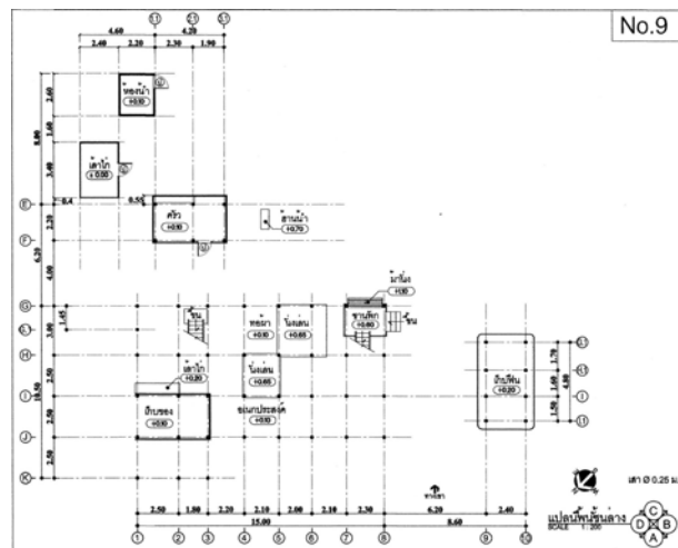
ภาพที่ 4.70 แสดงพื้นที่ชั้นล่าง หลังที่ 9 ชุมชนนาเรือน
