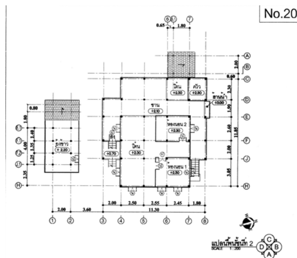
ภาพที่ 4.156 แสดงแปลนพื้นชั้นบน หลังที่ 20 ชุมชนบ้านอาราม ที่มา : จากการสำรวจ ปี พ.ศ. 2552
