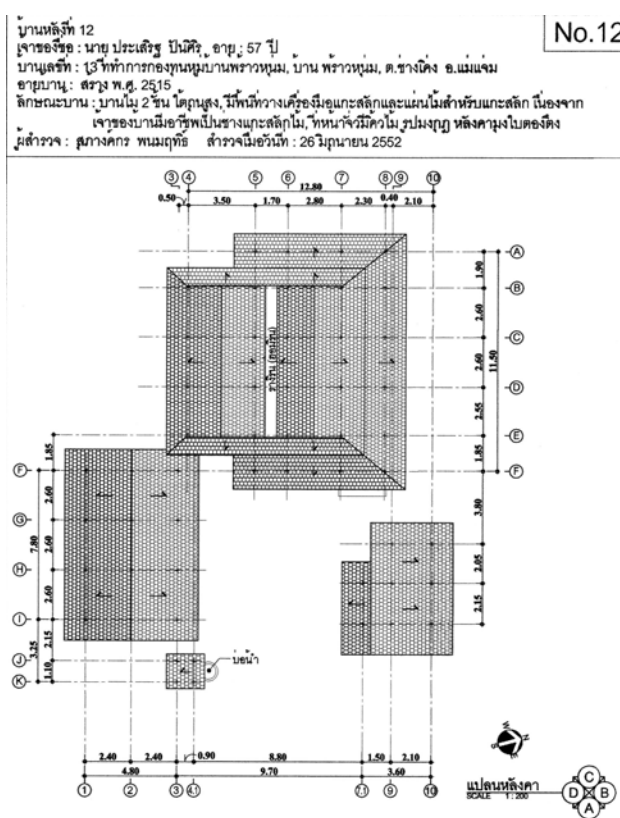
ภาพที่ 4.91 แสดงแปลนหลังคา หลังที่ 12 ชุมชนพรวัวหนุ่ม
