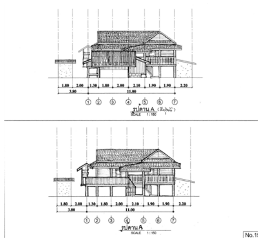
ภาพที่ 4.117 แสดงรูปด้าน A หลังที่ 15 ชุมชนพริ้วหนุ่ม ที่มา : จากการสำรวจ ปี พ.ศ. 2552
