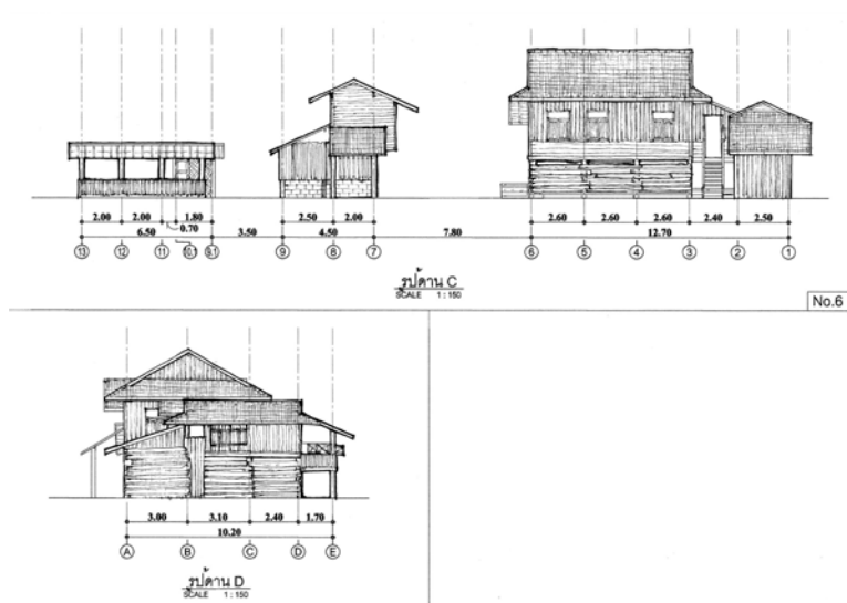
ภาพที่ 4.53 แสดงรูปด้าน C รูปด้าน D หลังที่ 6 ชุมชนเหล่าปากอ(ป่าแดด)
