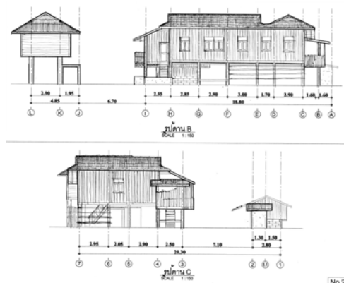
ภาพที่ 4.172 แสดงรูปด้าน B รูปด้าน C หลังที่ 24 ชุมชนบ้านไร่ ที่มา : จากการสำรวจ ปี พ.ศ. 2552
