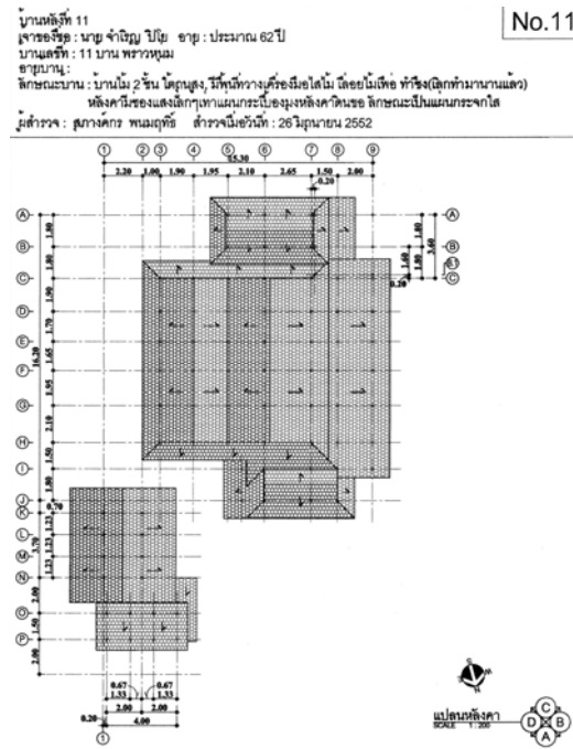
ภาพที่ 4.84 แสดงแปลนหลังคา หลังที่ 11 ชุมชนพรวนหมื่น ที่มา : จากการสำรวจ ปี พ.ศ. 2552
