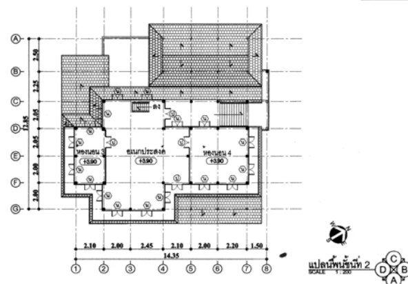
ภาพที่ 4.78 แสดงแปลนพื้นที่ชั้นบน หลังที่ 10 ชุมชนพรวัวหนุ่ม
