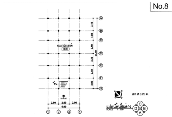
ภาพที่ 4.65 แสดงแปลนหลังคา หลังที่ 8 ชุมชนนาเรือน
