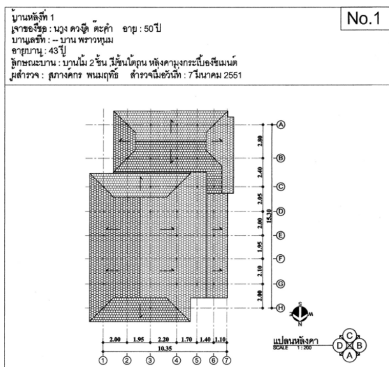
ภาพที่ 4.14 แสดงแปลนหลังคา บ้านหลังที่1 ชุมชนพร้าวหนูม
