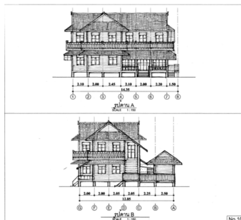
ภาพที่ 4.79 แสดงรูปด้าน A รูปด้าน B หลังที่ 10 ชุมชนพรวัวหนุ่ม
