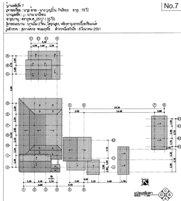
ภาพที่ 4.57 แสดงแปลนหลังคา หลังที่ 7 ชุมชนนาเรือน
