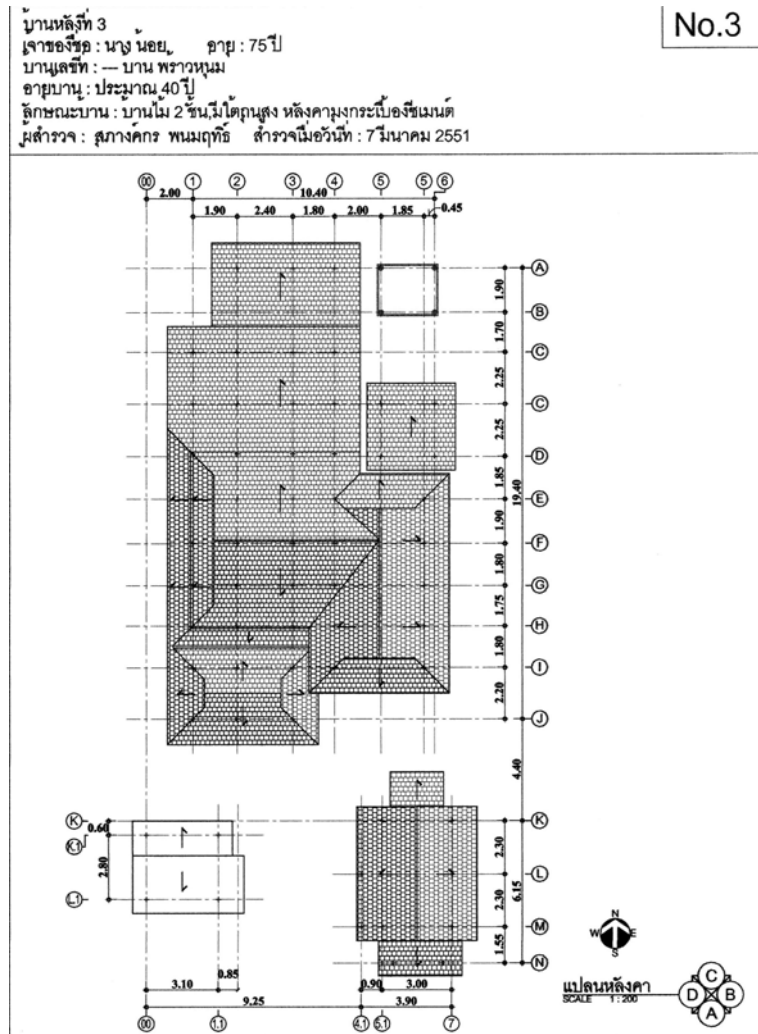
ภาพที่ 4.26 แสดงแปลนหลังคา หลังที่ 3 ชุมชนพรวนหม่ม ที่มา : จากการสำรวจ ปี พ.ศ. 2551
