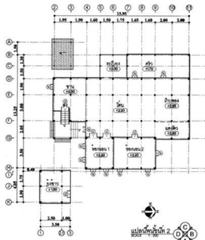
ภาพที่ 4.108 แสดงแปลนพื้นชั้นบน หลังที่ 14 ชุมชนพริ้วหนุ่ม ที่มา : จากการสำรวจ ปี พ.ศ. 2552
