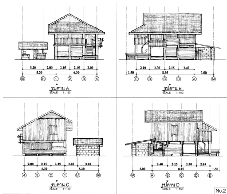
ภาพที่ 4.23 แสดงรูปด้าน หลังที่2 ชุมชนพรวัวหนุ่ม
