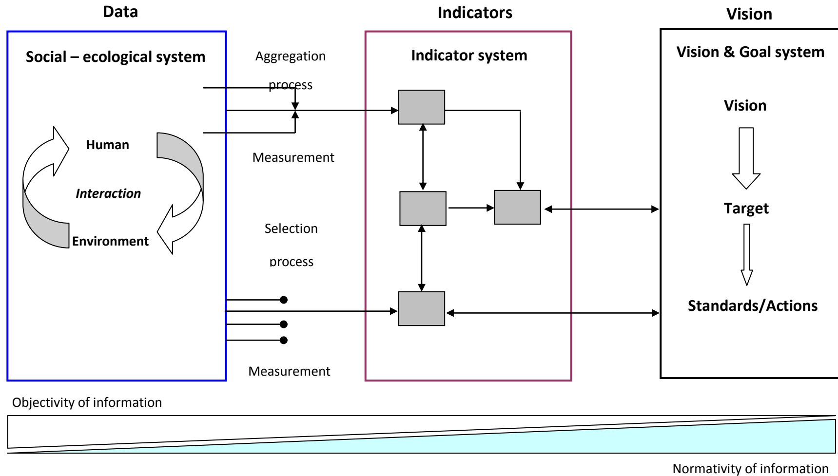
รูปที่ 3.4 แนวทางการพัฒนาดัชนีความล่อแหลม ภายใต้กระบวนการ Data-indicator-goal model (ดัดแปลงจาก Cabri-Volga Project Deliverable D3; www.cabri-volga.org )
