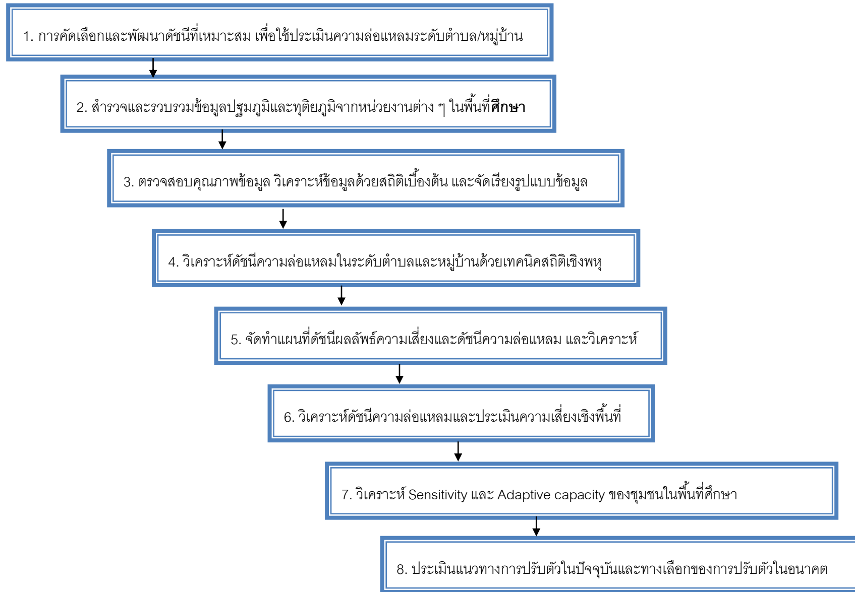
รูปที่ 3.2 ขั้นตอนการศึกษาวิจัยวิเคราะห์ความล่อแหลม และประเมินความเสี่ยงจากสภาวะความรุนแรงของฝน ในพื้นที่จังหวัดนครศรีธรรมราชและจังหวัดฉะเชิงเทรา
