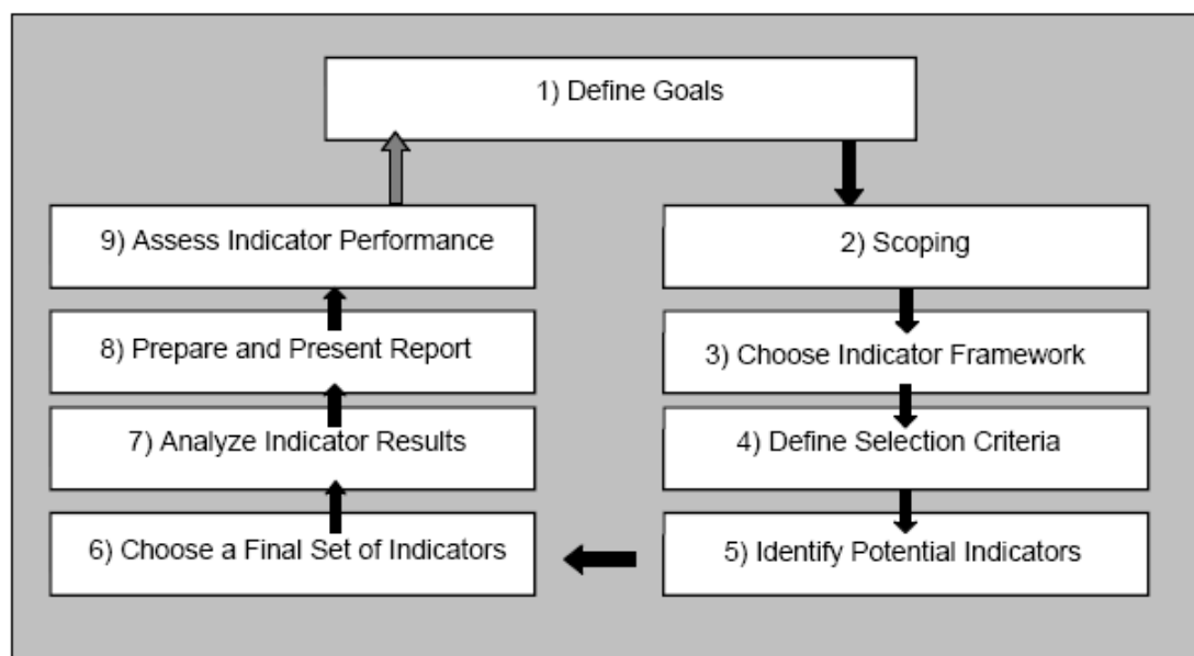
รูปที่ 3.5 ขั้นตอนการพัฒนาดัชนีความอ่อนแอ ภายใต้กระบวนการ Data-indicator-goal model (ดัดแปลงจาก Cabri-Volga Project Deliverable D3; www.cabri-volga.org )
