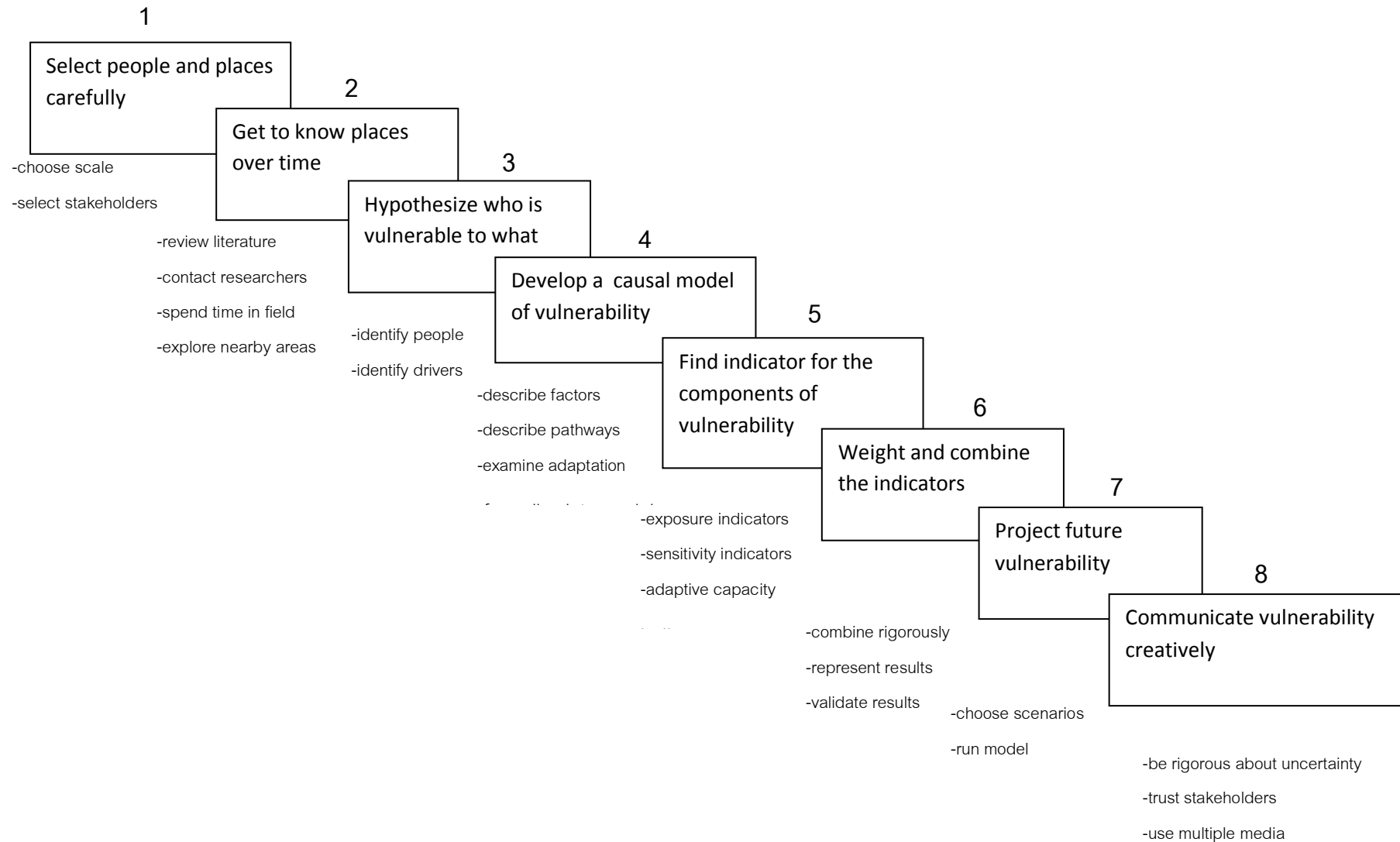
รูปที่ 2.13 ขั้นตอนสำหรับการประเมินความล่อแหลมจากการเปลี่ยนแปลงของโลกและการเปลี่ยนแปลงภูมิอากาศ
