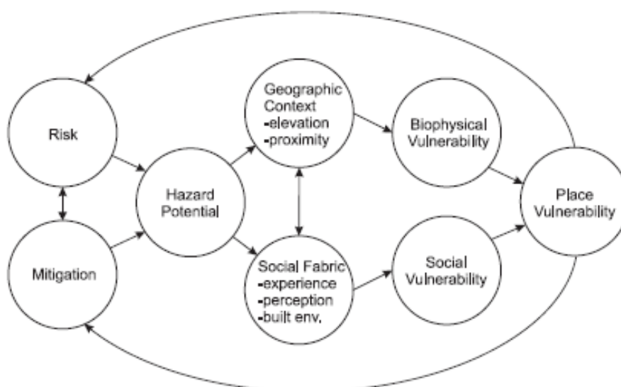
รูปที่ 2.8 องค์ประกอบของ Hazards-of-Place model of vulnerability
