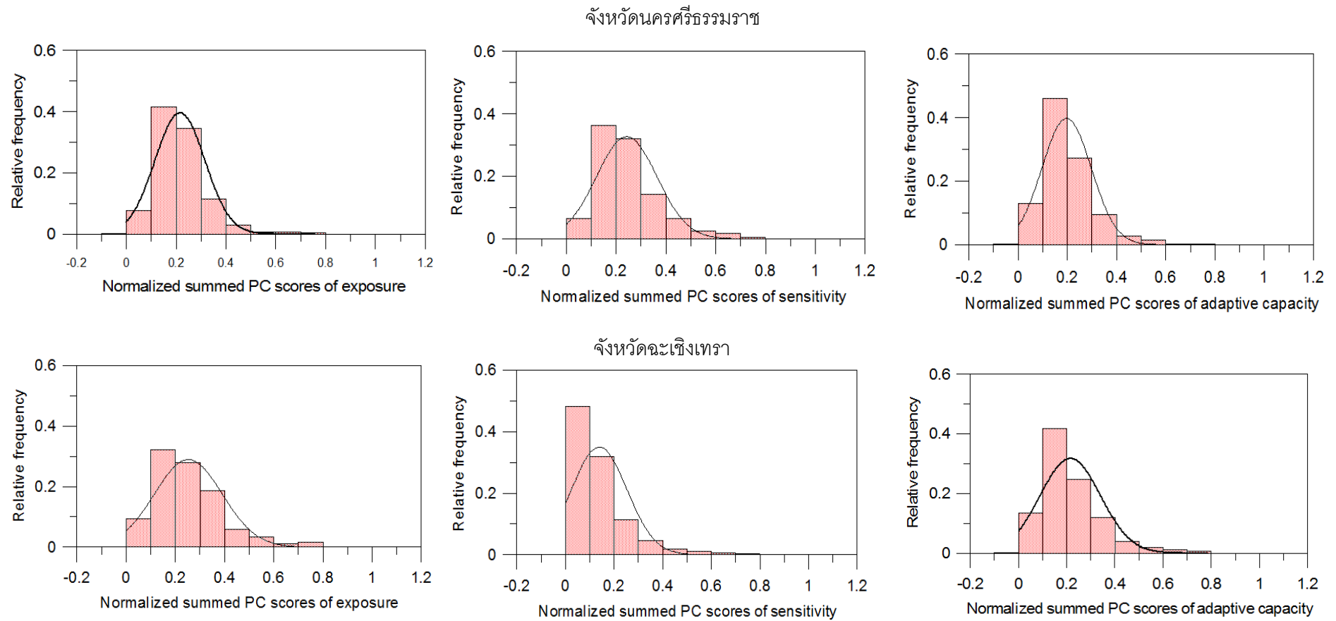
รูปที่ 4.38 Histogram ของ normalized summed PC scores
