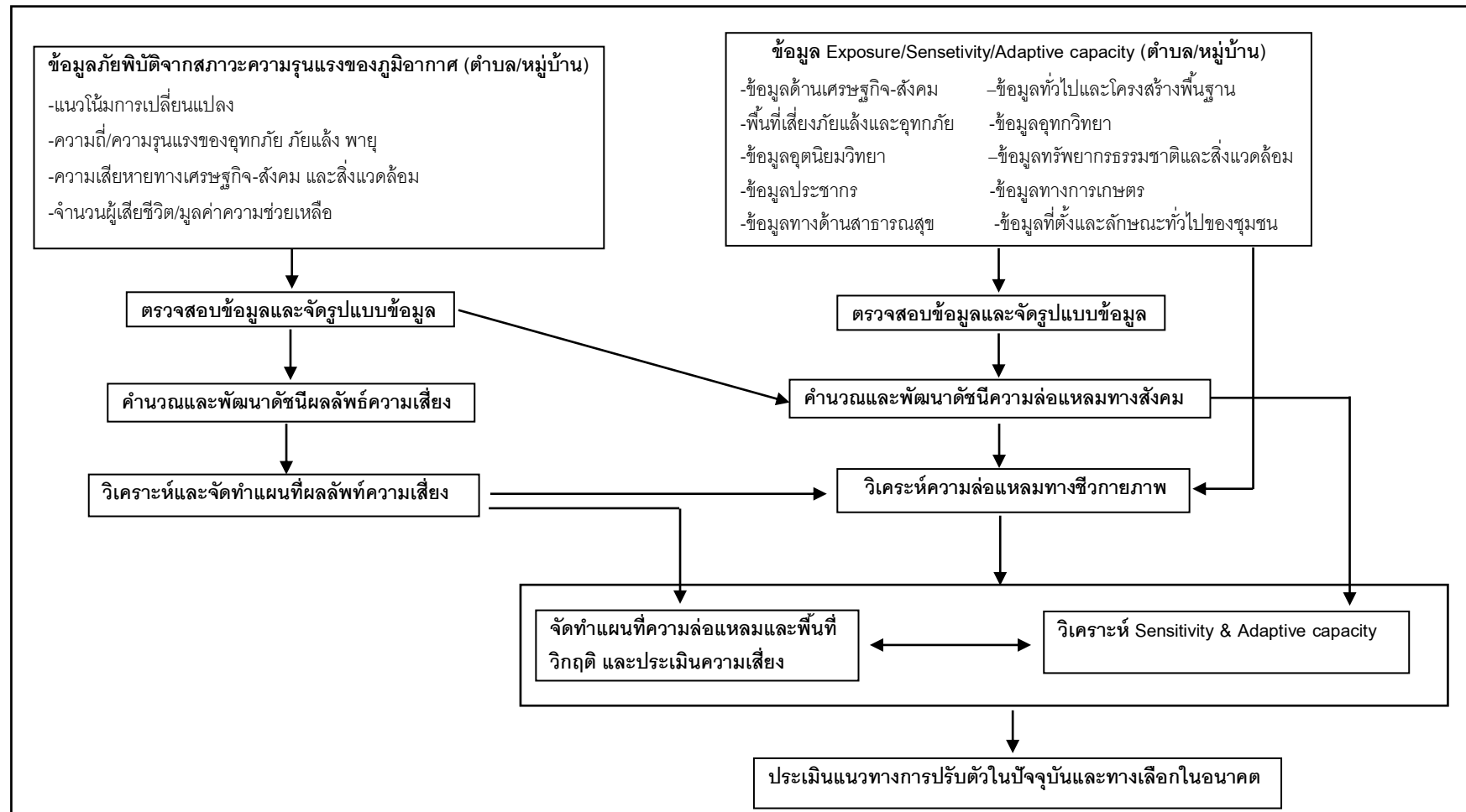
รูปที่ 3.1 กรอบแนวคิดของการศึกษาวิจัยการวิเคราะห์ความล่อแหลมและการประเมินความเสี่ยงในพื้นที่วิกฤติจากสภาวะความรุนแรงของฝน
