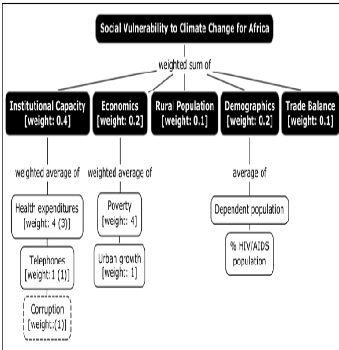
รูปที่ 2.20 โครงสร้างรวมของ Index of Social Vulnerability to Climate Change โดยดัชนีแสดงด้วยกล่องสีขาว Sub-indices และ SVA แสดงด้วยกล่องสีดำ
