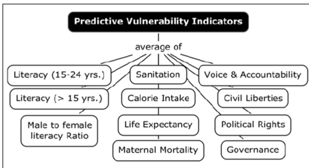
รูปที่ 2.22 โครงสร้างรวมของ Predictive Vulnerability Indicators โดยดัชนีแสดงด้วยกล่องสีขาว Sub-indices และ PIV แสดงด้วยกล่องสีดำ
