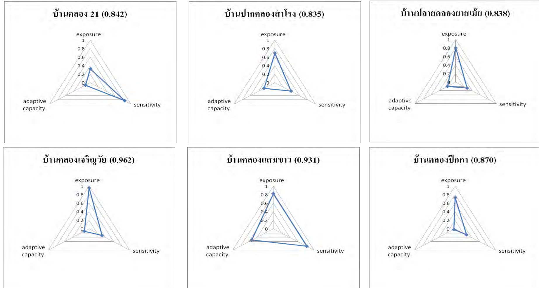
รูปที่ 4.52 Spider plot ของค่า Exposure score, Sensitivity score และ Adaptive capacity score ของหมู่บ้านในจังหวัดเชียงใหม่ ที่มีค่าดัชนี CoVi สูงกว่าเปอร์เซ็นต์ไทล์ที่ 80
