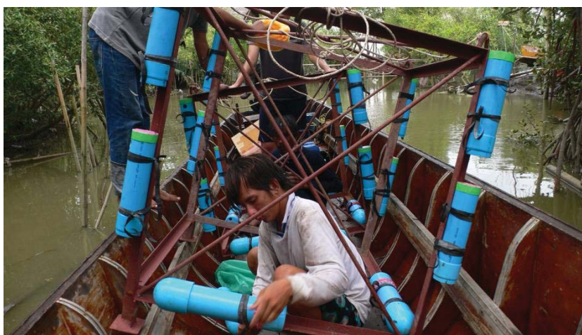
รูปที่ 7.4 รูปของเครื่องดักตะกอนที่ทำจากเหล็กฉากและท่อพีวีซี (แบบ 3 ระดับ)
