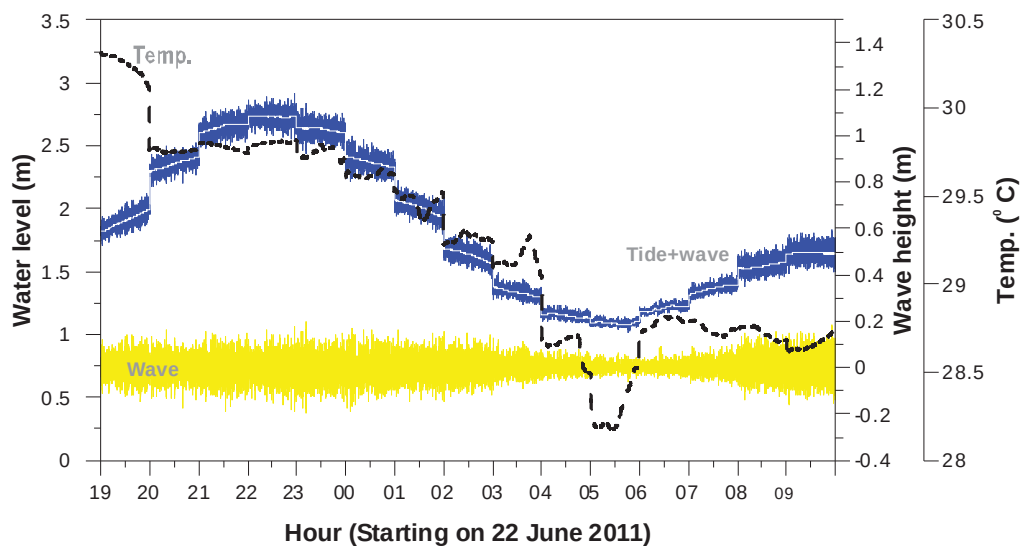
รูปที่ ก-100 ข้อมูล คลื่น น้ำขึ้นน้ำลง และอุณหภูมิ ในวันที่ 22-23 มิถุนายน พ.ศ. 2554
