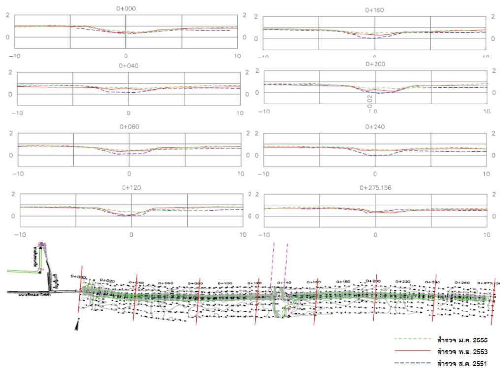
รูปที่ 5.2 (ล่าง) แสดงผลการสำรวจระดับพื้นที่ถนนบริเวณที่มีการติดตั้งโครงสร้างเสาสามเหลี่ยม “เชื่อมสลายกำลังคลื่น” โดยทำการรังวัดชั้นรายละเอียดห่างจากแนวเสาเข็มสามเหลี่ยมข้างละ 10 เมตร ตลอดแนวเชื่อมสลายกำลังคลื่น (บน) แสดงข้อมูลภาพตัดขวางของพื้นที่ถนนบริเวณที่มีการติดตั้งเชื่อมสลายกำลังคลื่นทุกๆ 40 เมตร โดยมีการเปรียบเทียบข้อมูลที่มีการตรวจวัดไว้เมื่อเดือนสิงหาคม พ.ศ. 2551, เดือนพฤศจิกายน พ.ศ. 2553 และ เดือนมกราคม พ.ศ. 2555
