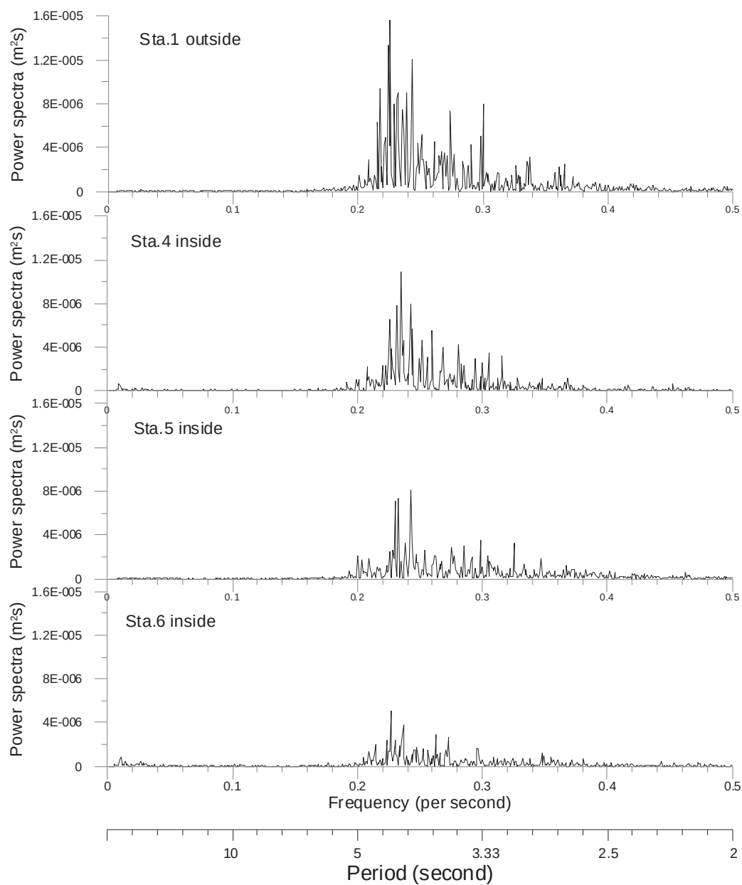
รูปที่ ก-85 พลังงานคลื่น เทียบกับความถี่ และคาบคลื่น ในวันที่ 20-21 กุมภาพันธ์ พ.ศ. 2554
