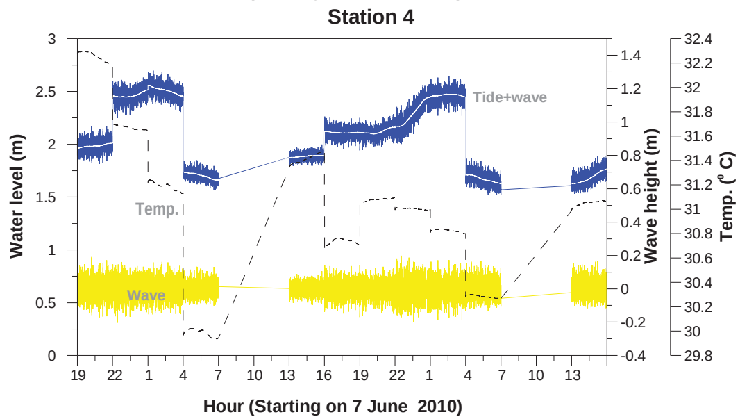
รูปที่ ก-35 ข้อมูล คลื่น น้ำขึ้นน้ำลง และอุณหภูมิ ในวันที่ 7-9 มิถุนายน พ.ศ. 2553
