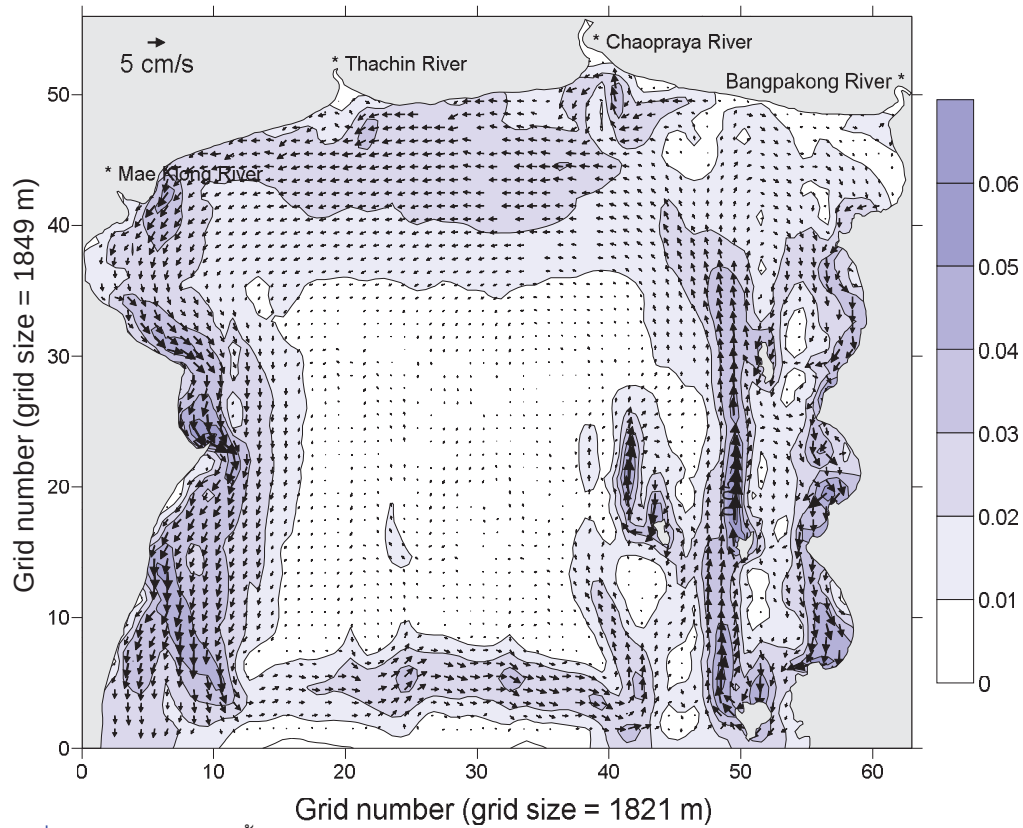
รูปที่ 9.9 ตัวอย่างกระแสน้ำสุทธิสำหรับช่วงฤดูมรสุมตะวันออกเฉียงเหนือในเดือนพฤศจิกายน-ธันวาคม พ.ศ. 2553
