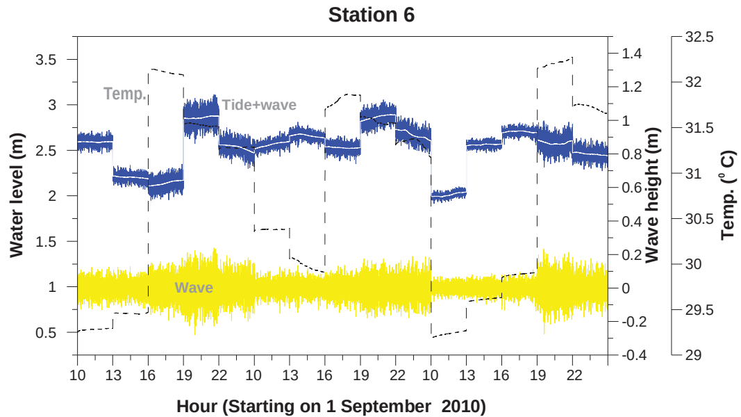
รูปที่ ก-57 ข้อมูล คลื่น น้ำขึ้นน้ำลง และอุณหภูมิ ในวันที่ 1-3 กันยายน พ.ศ. 2553
