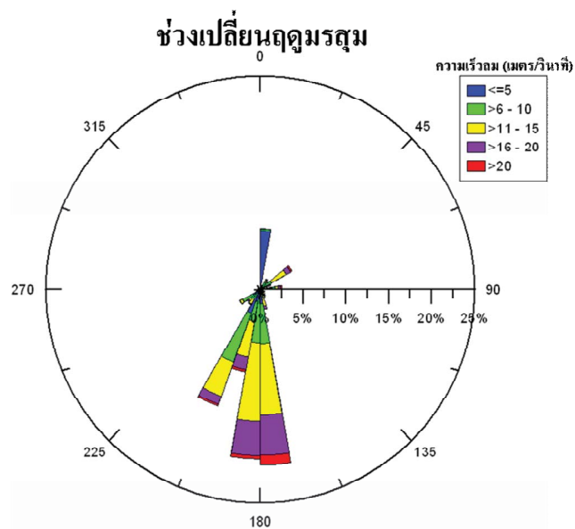
รูปที่ 2.4 Wind rose แสดงทิศทางและความเร็วลมช่วงเปลี่ยนฤดูมรสุม
