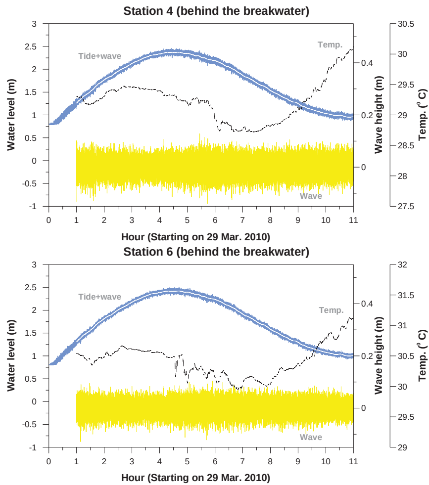
รูปที่ ก-22 ข้อมูล คลื่น น้ำขึ้นน้ำลง และอุณหภูมิ ในวันที่ 29 พฤศจิกายน พ.ศ. 2553
