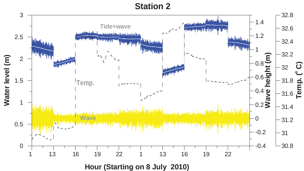
รูปที่ ก-41 ข้อมูล คลื่น น้ำขึ้นน้ำลง และอุณหภูมิ ในวันที่ 8-9 กรกฎาคม พ.ศ. 2553
