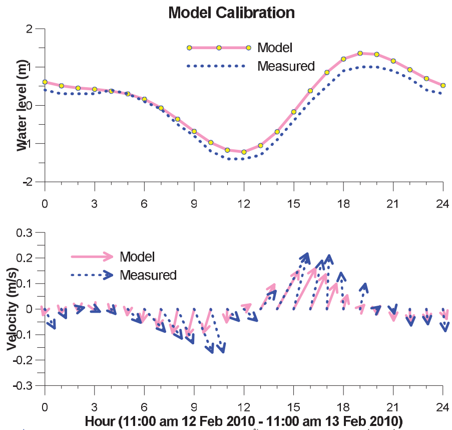
รูปที่ 9.3 การเปรียบเทียบแบบจำลองการไหลเวียนของน้ำกับข้อมูลการตรวจวัดที่ชายฝั่งบ้านขุนสมุทรจีน เมื่อวันที่ 12-13 กุมภาพันธ์ พ.ศ. 2553
