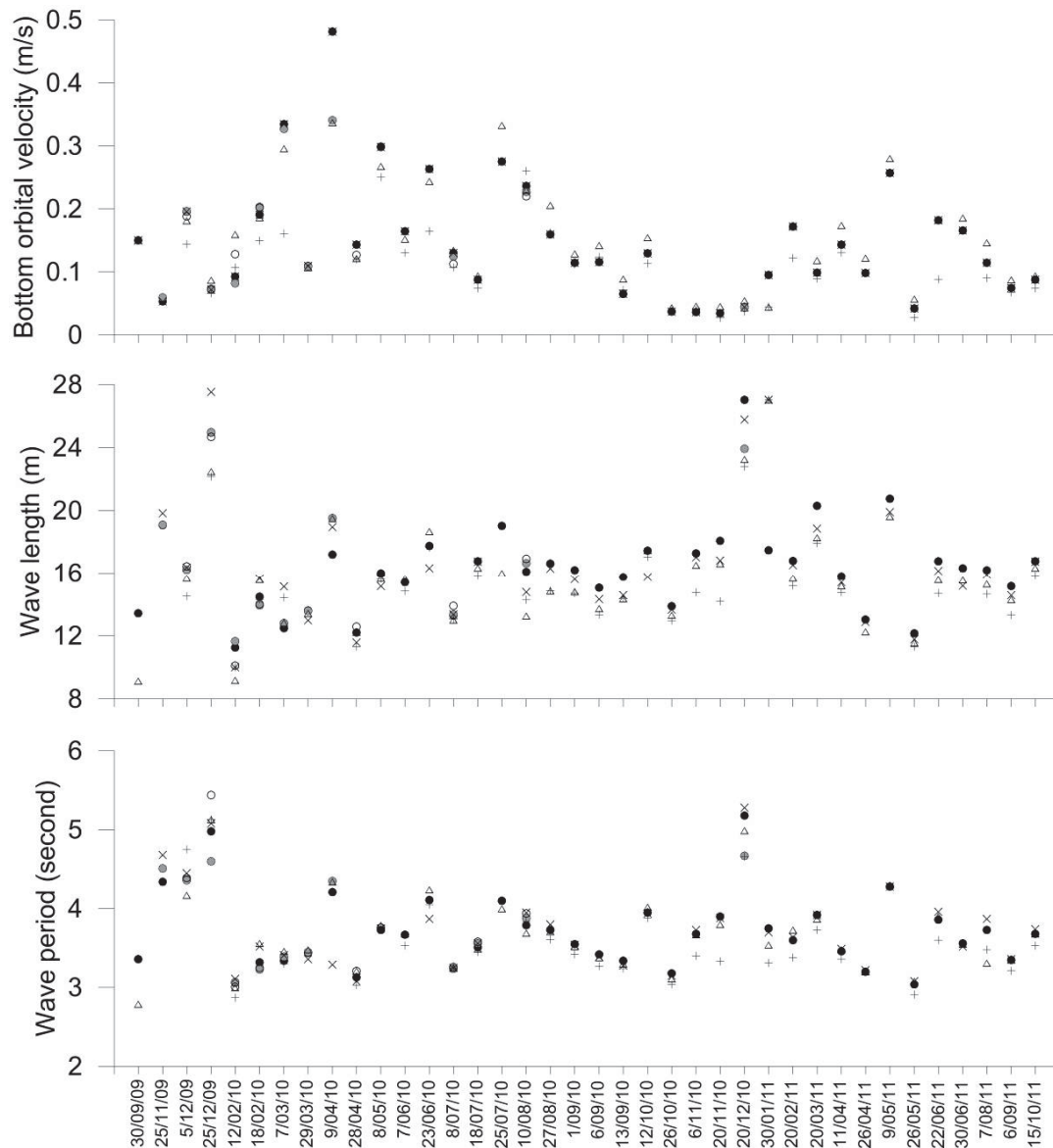
รูปที่ 3.5 ความเร็วกระแสน้ำเป็นวงเนื่องจากคลื่นที่ตื้นน้ำ (Bottom orbital velocity, m/s) ความยาวคลื่น (Wave length, m) และคาบคลื่น (Wave period, second) (วงกลมสีดำ วงกลมสีขาว และวงกลมสีเทา คือจุดตรวจวัดคลื่นด้านหน้า เขื่อนจุดที่ 1 จุดที่ 2 และจุดที่ 3 ตามลำดับ สามเหลี่ยม เครื่องหมายบวก และเครื่องหมายกากบาท คือจุดตรวจวัดคลื่นด้านหลังเขื่อนจุดที่ 4 จุดที่ 5 และจุดที่ 6 ตามลำดับ)
