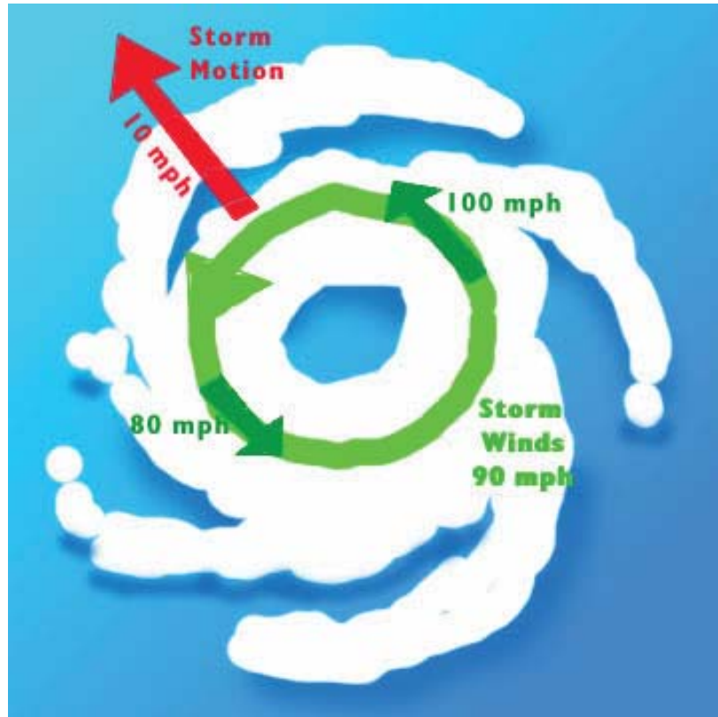
รูปที่ 2.11 แบบจำลองการหมุนของลมรอบพายุในทิศทวนเข็มนาฬิกา และความเร็วลมที่สอดคล้องกับทิศทางการเคลื่อนที่
