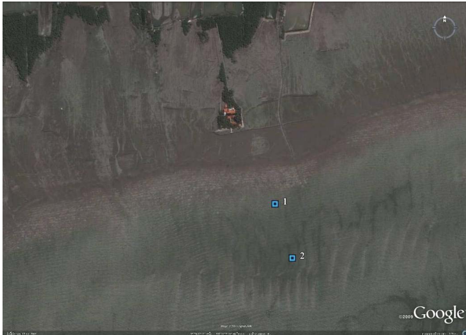
รูปที่ 7.5 จุดติดตั้งเครื่องดักตะกอน จุดที่ 1 และ 2 ห่างจากชายฝั่งประมาณ 0.8 และ 1.3 กิโลเมตร ตามลำดับ
