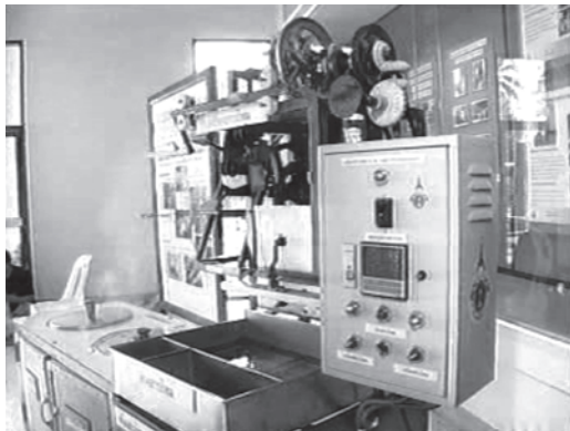
ภาพที่ 5 แสดงการควบคุมอุณหภูมิอย่างสาวใหม่ ที่ปรับตั้งค่าได้พร้อมจอแสดงผล
