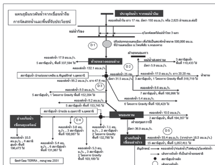
ภาพที่ 2 แผนภูมิแนวผันน้ำจากเขื่อนน้ำจี้ม และพื้นที่รับประโยชน์ในประเทศไทย
