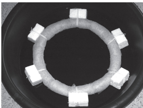
ภาพที่ 3: การทดลองใช้ทุ่นลอยจากแกลบควบคุมคราบน้ำมัน
