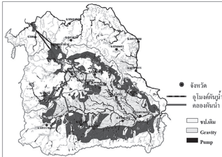
ภาพที่ 3 แสดงแนวผันน้ำโขงจากปากแม่น้ำเลย สู่พื้นที่ชลประทาน 15 จังหวัดภาคอีสาน
