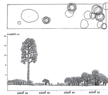
ภาพที่ 2 โปรไฟล์ในทามในป่าทามลำเซบาย ตำบลนาแก อำเภอดำเขื่อนแก้ว จังหวัดยโสธร
