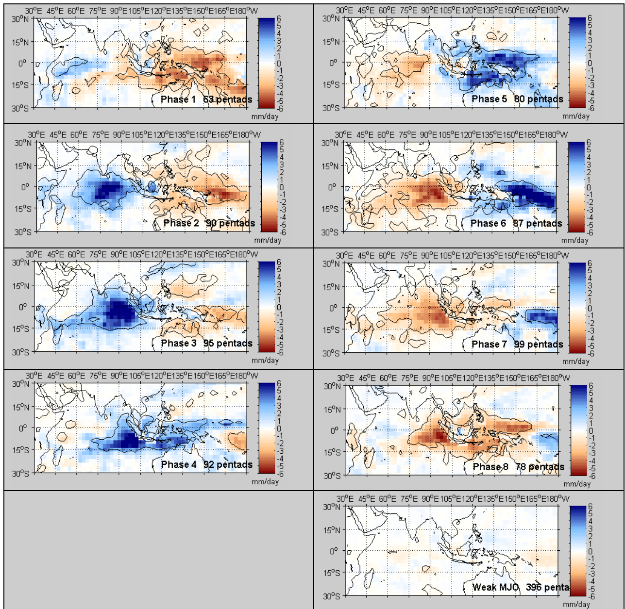
รูปที่ 4.6 เช่นเดียวกับรูปที่ 4.4 เฉพาะระหว่างเดือนพฤศจิกายนถึงเดือนเมษายน
