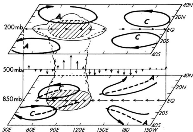
รูปที่ 2.3 แผนภาพแสดงการไหลเวียนอากาศที่สัมพันธ์กับปรากฏการณ์ MJO สัญลักษณ์ก่อนเมฆแทนศูนย์กลางของกลุ่มเมฆฝน ลูกศรแสดงทิศทางของความเร็วลมที่ระดับ 850 hPa และ 200 hPa และความเร็วลมในแนวตั้งที่ระดับ 500 hPa ตัวอักษร A และ C แทน anticyclones และ cyclones ตามลำดับ เส้นประแทน troughs กับ ridges ที่มา: Rui and Wang (1990)
