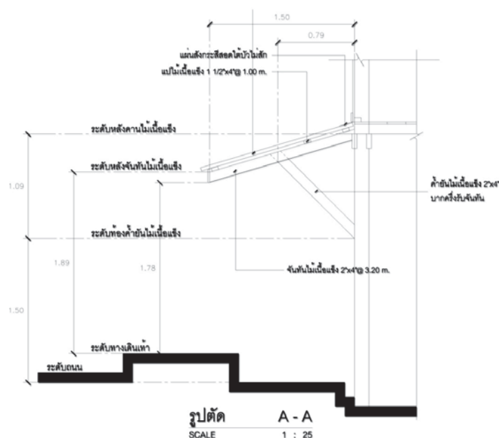
ภาพ 1-2 รายละเอียดตัดกันอาคารการปรับปรุงอาคาร (เจ้าของบ้านคุณบุญจิรา ทองเขียว)
