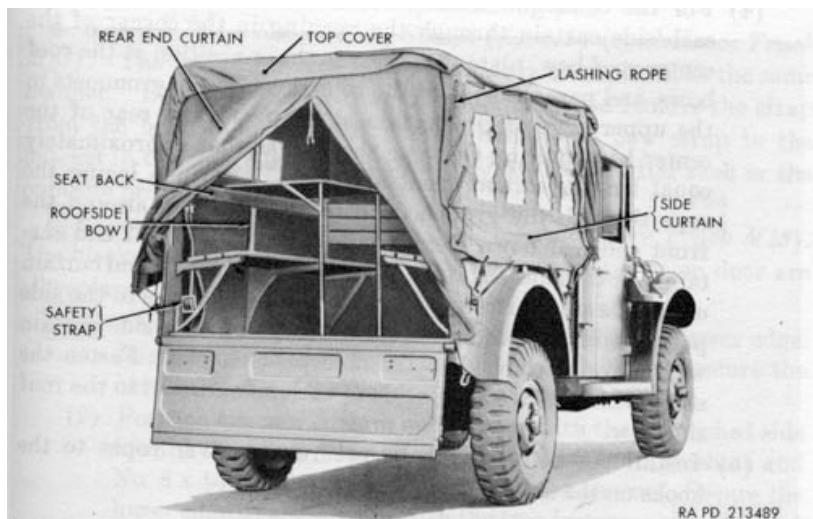
รูปที่ 2.17 รถบรรทุก M42 Dodge 3/4 ton 4x4 Command Truck (ด้านหลัง)
