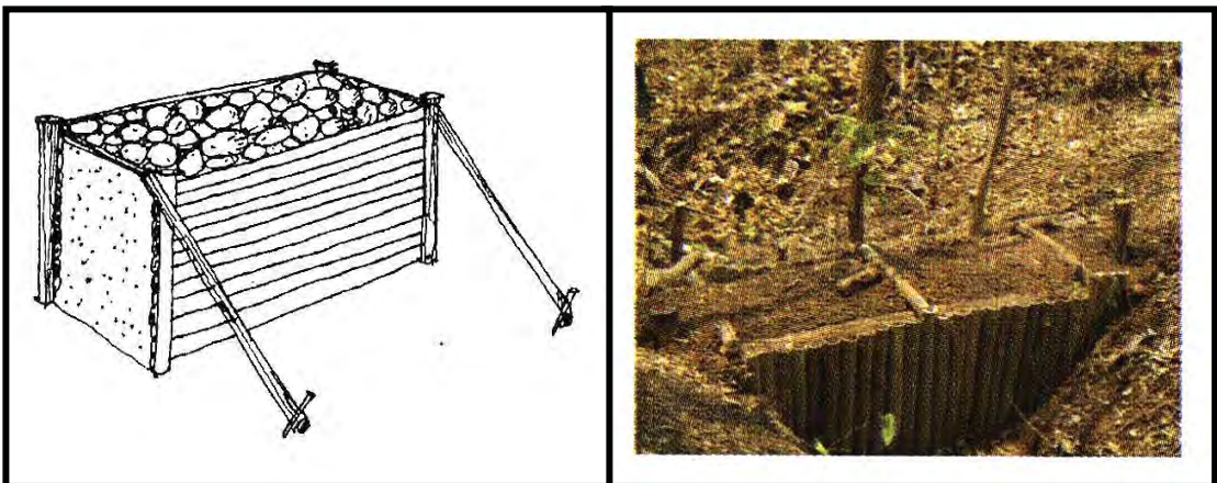
รูปที่ 2.7 ฝายไม้แกนดินเหนียว
